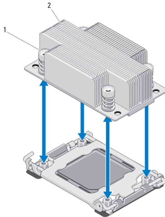
Figure 14. Installation et retrait d'un dissipateur de chaleur
