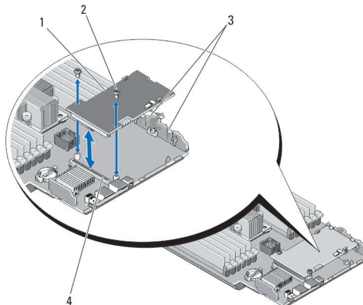
Abbildung 22. PCIe-Erweiterungskarte/Speichercontrollerkarte entfernen und installieren
