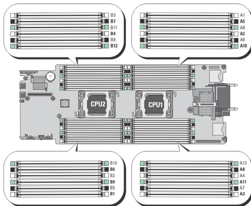
Abbildung 7. Positionen der Speichersockel
