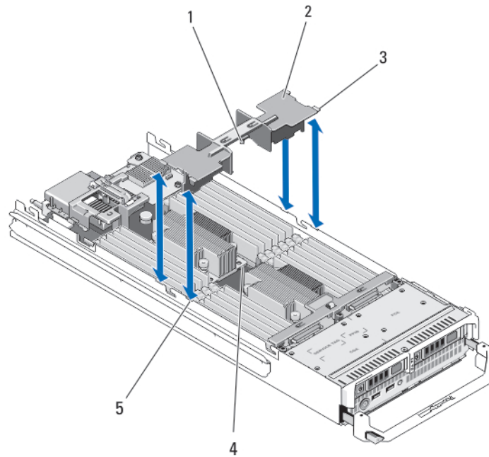
Abbildung 6. Kühlgehäuse installieren und entfernen
