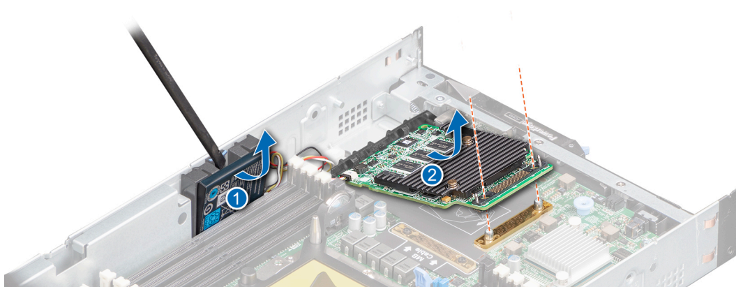
图 45: 卸下 RAID 控制器电池
