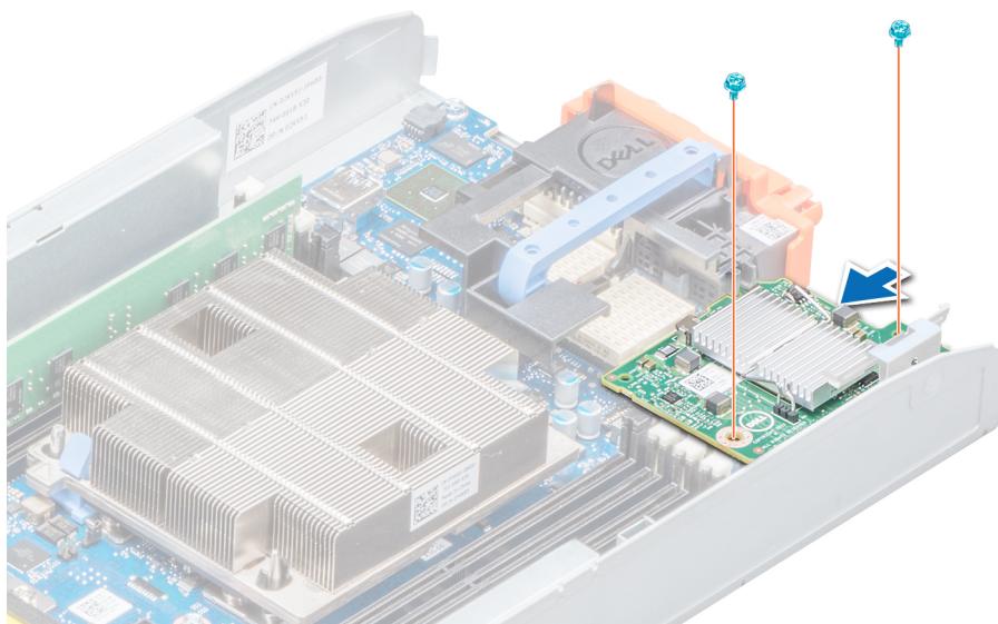
图 39: 安装网络子卡
