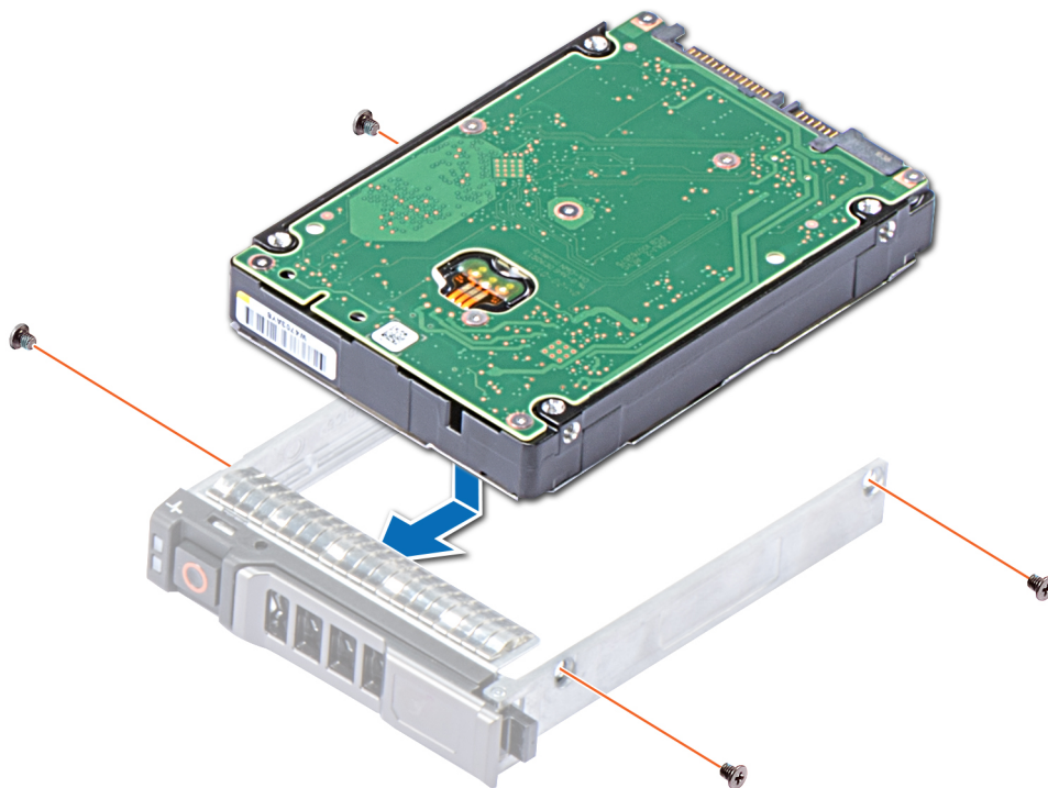
图 19: 将驱动器安装到驱动器托盘中
