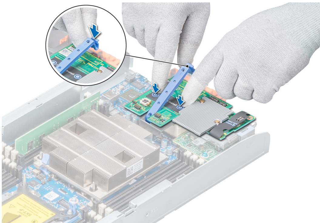
图 41: 安装 PCIe 夹层卡
