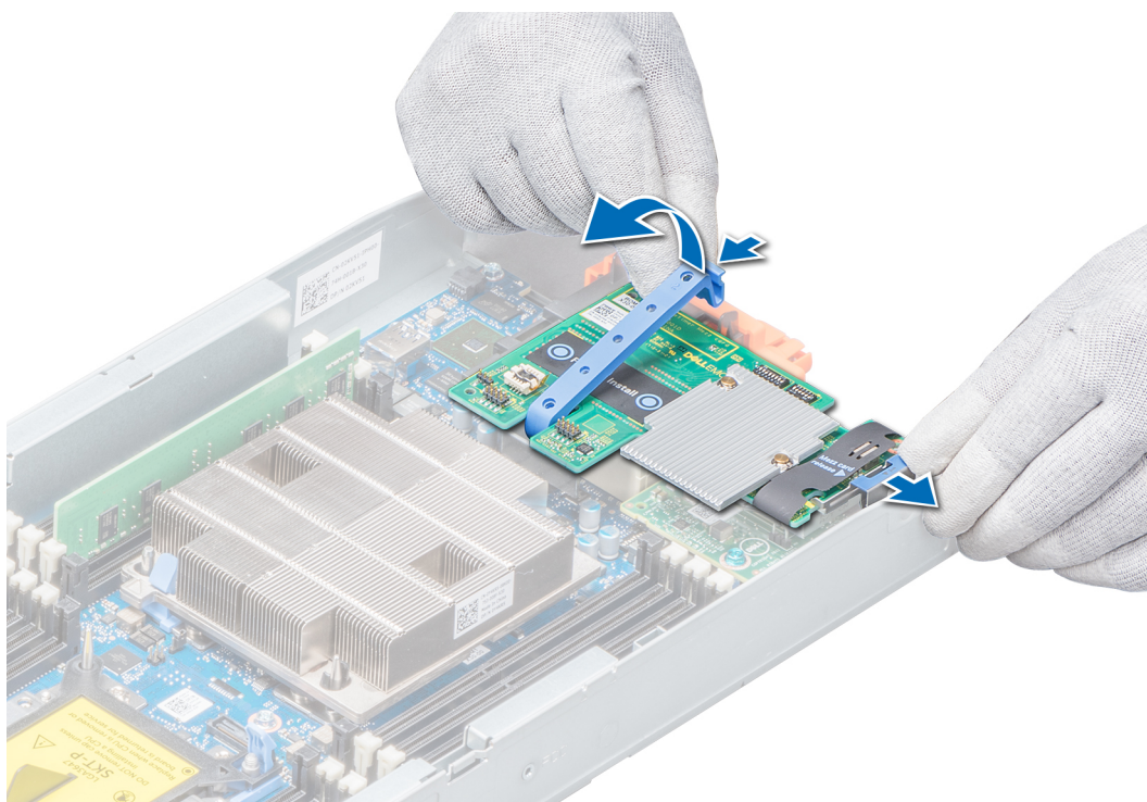
图 40: 卸下 PCIe 夹层卡
