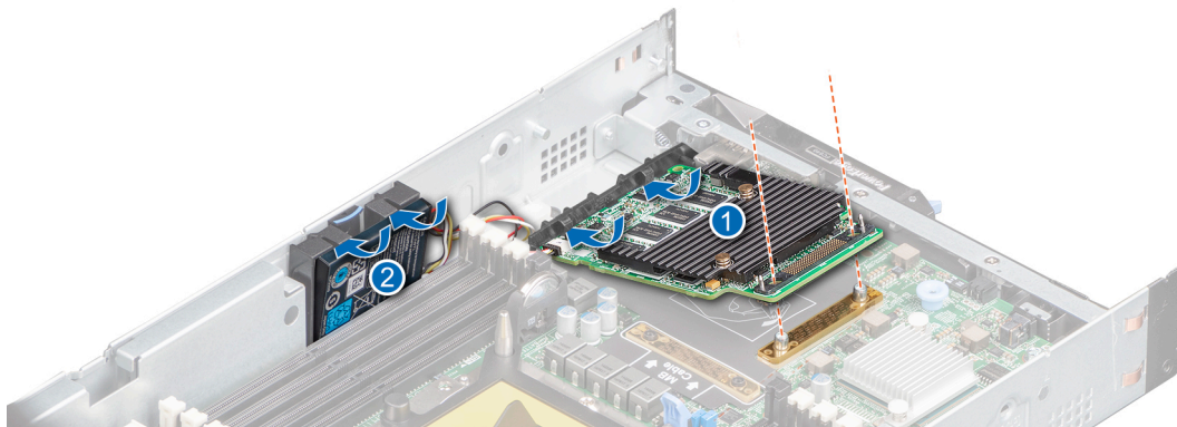
图 46: 安装 RAID 控制器电池
