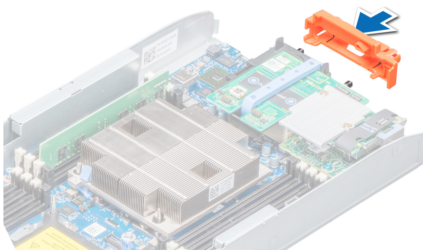
图 8: 安装 I/O 连接器护盖
