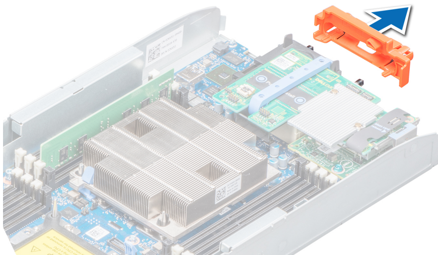
图 9: 卸下 I/O 连接器护盖
