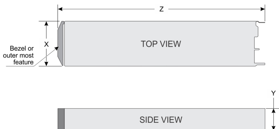
图 6: 系统尺寸
