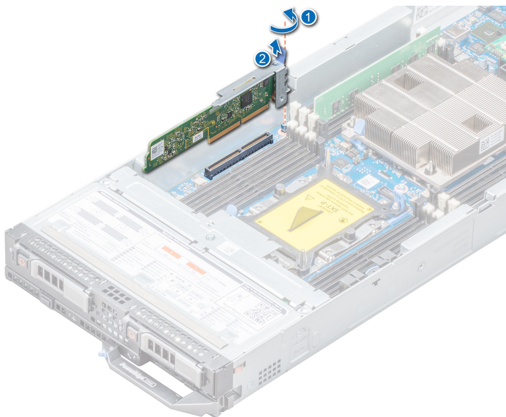
图 54: 卸下可选的 IDSDM 模块
