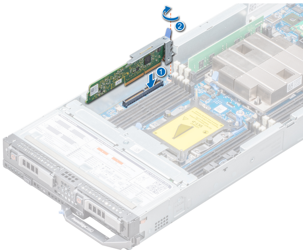
图 55: 安装可选的 IDSDM 模块
