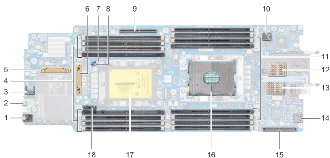
图 62: 系统板连接器
