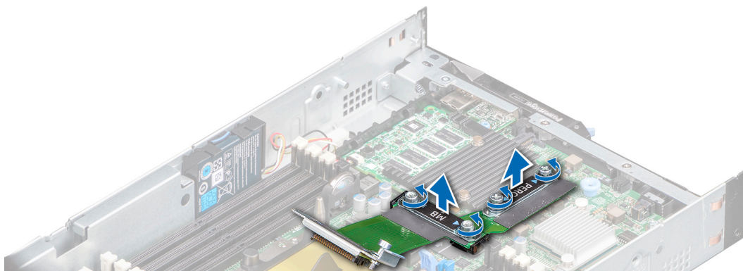
图 44: 卸下驱动器线缆连接器
