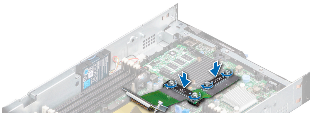
图 47: 安装驱动器线缆连接器
