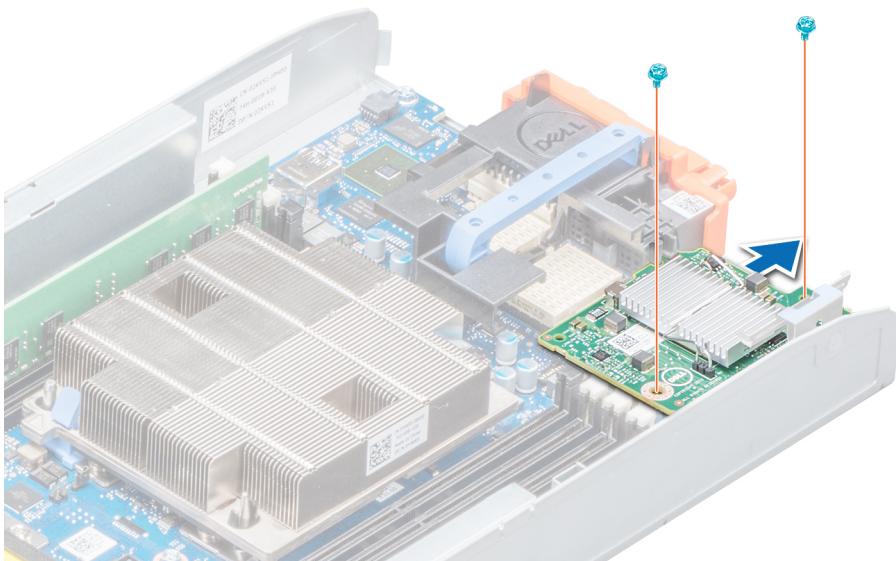
图 38: 卸下网络子卡
