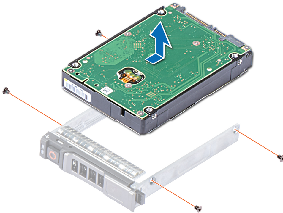
图 18: 从驱动器托盘中卸下驱动器
