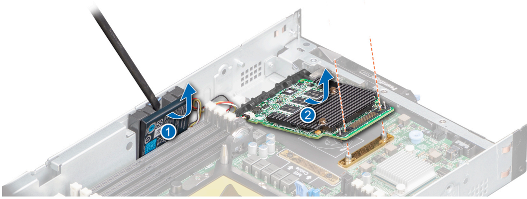
Rakam 45. RAID denetleyicisi pilini çıkarma
