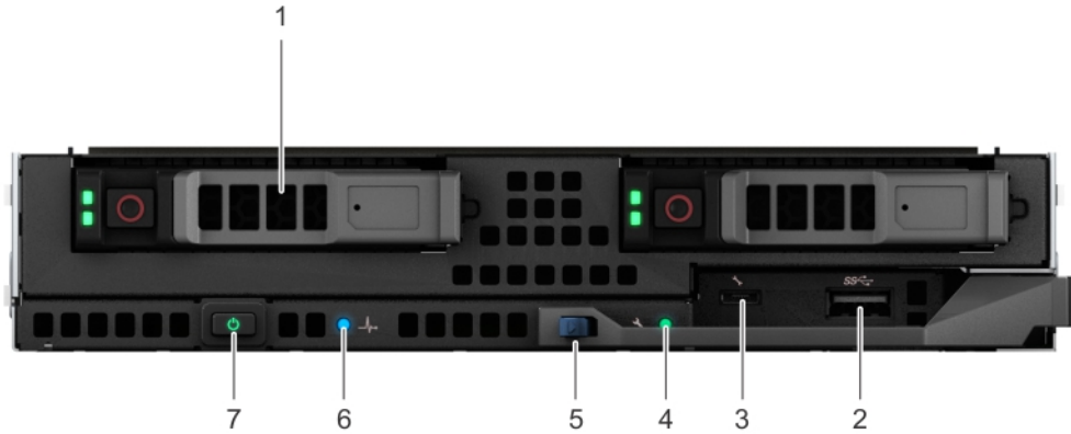
Rakam 1. Sistemin önden görünümü
