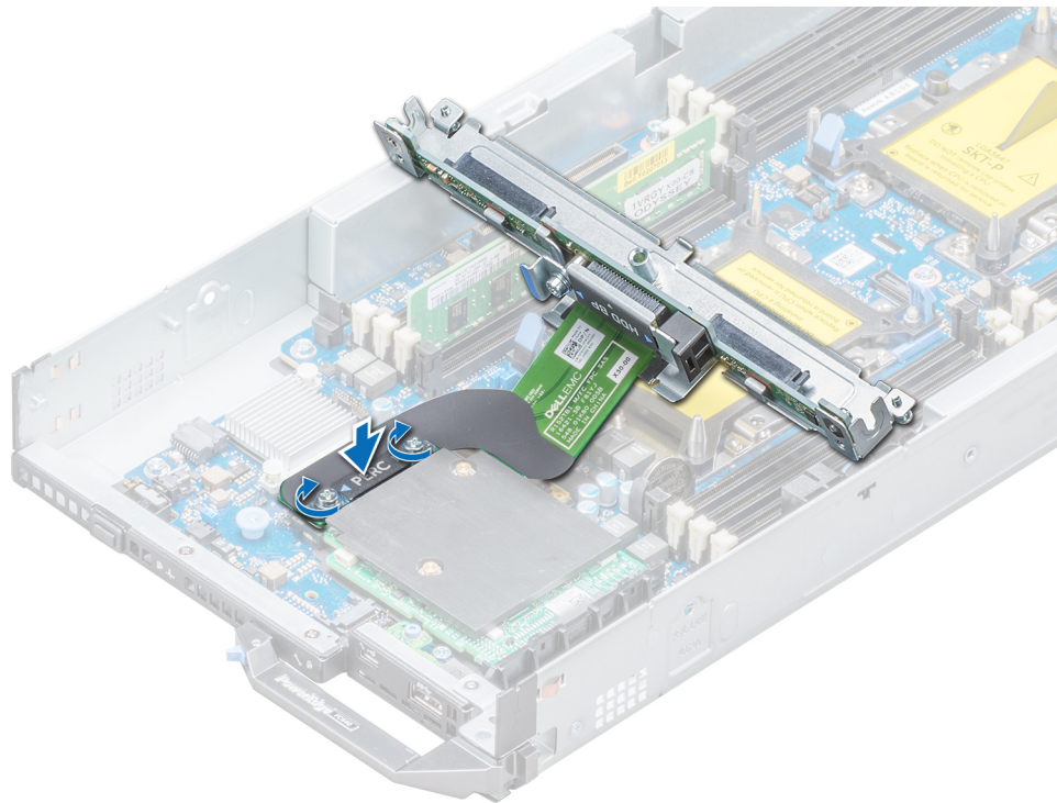
図 43. ストレージコントローラカードの取り付け
