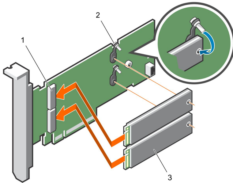
図 37. M.2 SSD モジュールの取り付け
