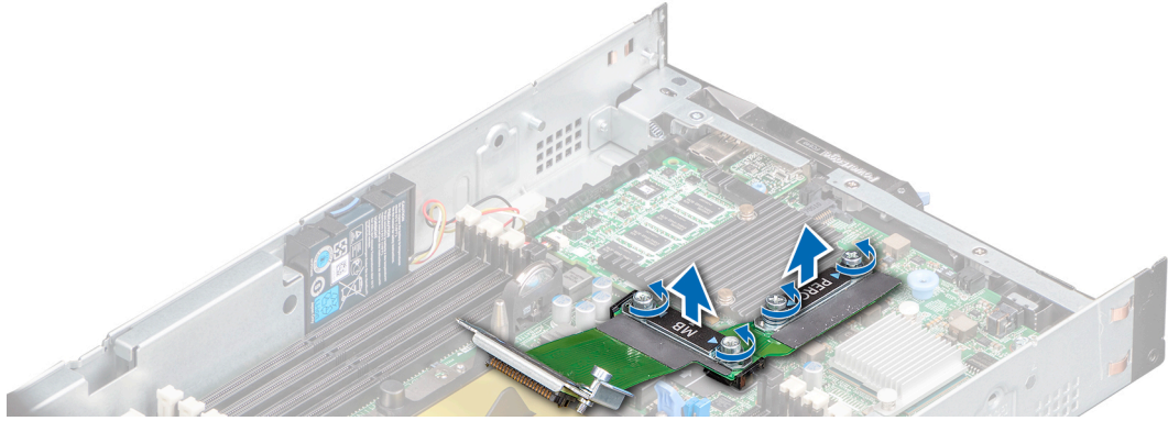
図 44. ドライブケーブル コネクタの取り外し
