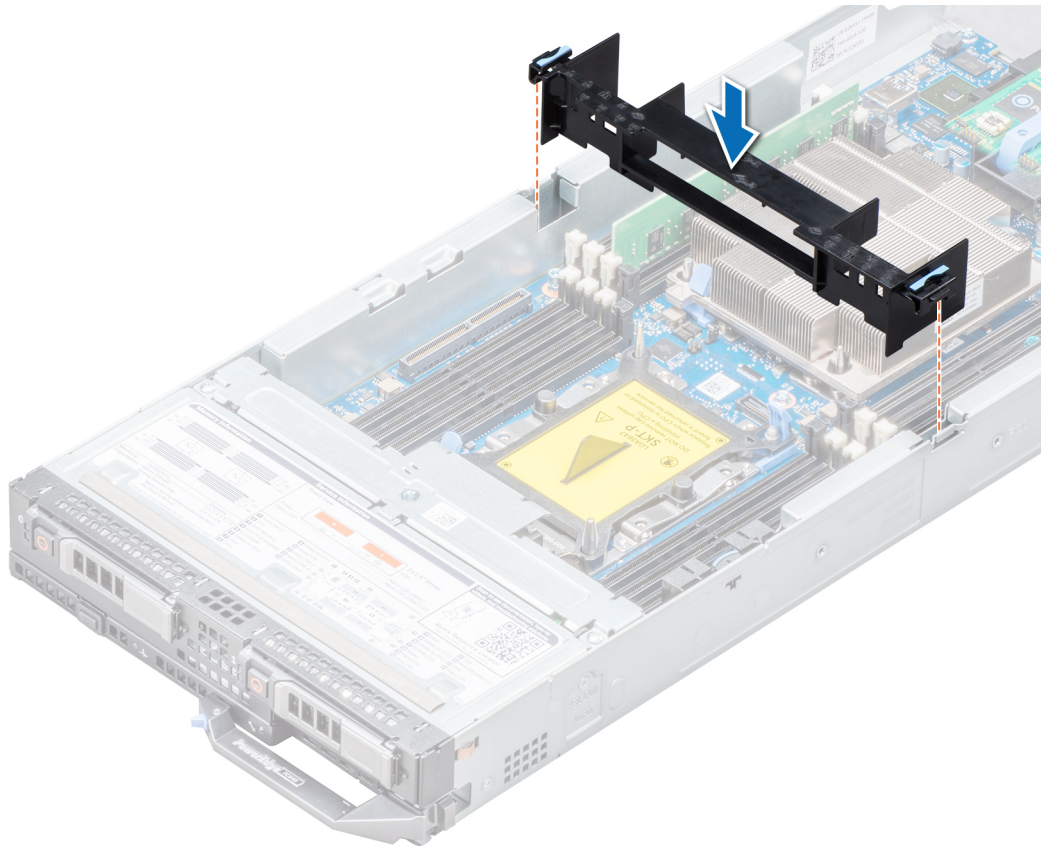
図 13. エアフローカバーの取り付け
