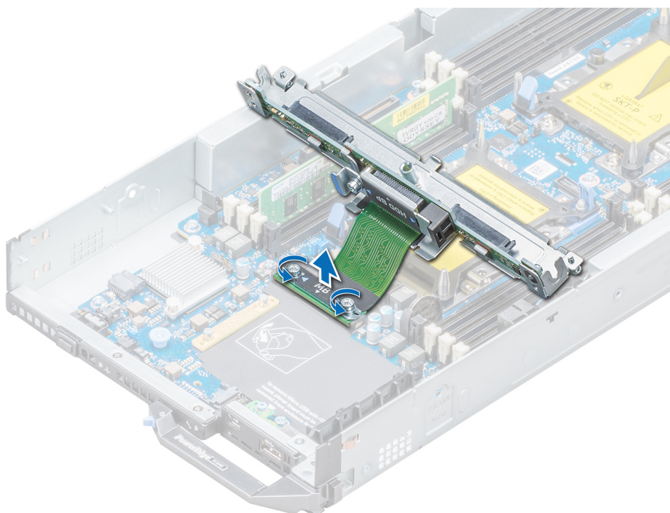
図 23. ドライブ バックプレーン ケーブルの取り外し
