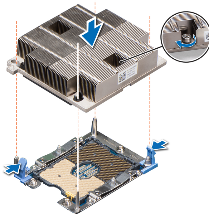
図 35. プロセッサ/ヒートシンク モジュールの取り付け
