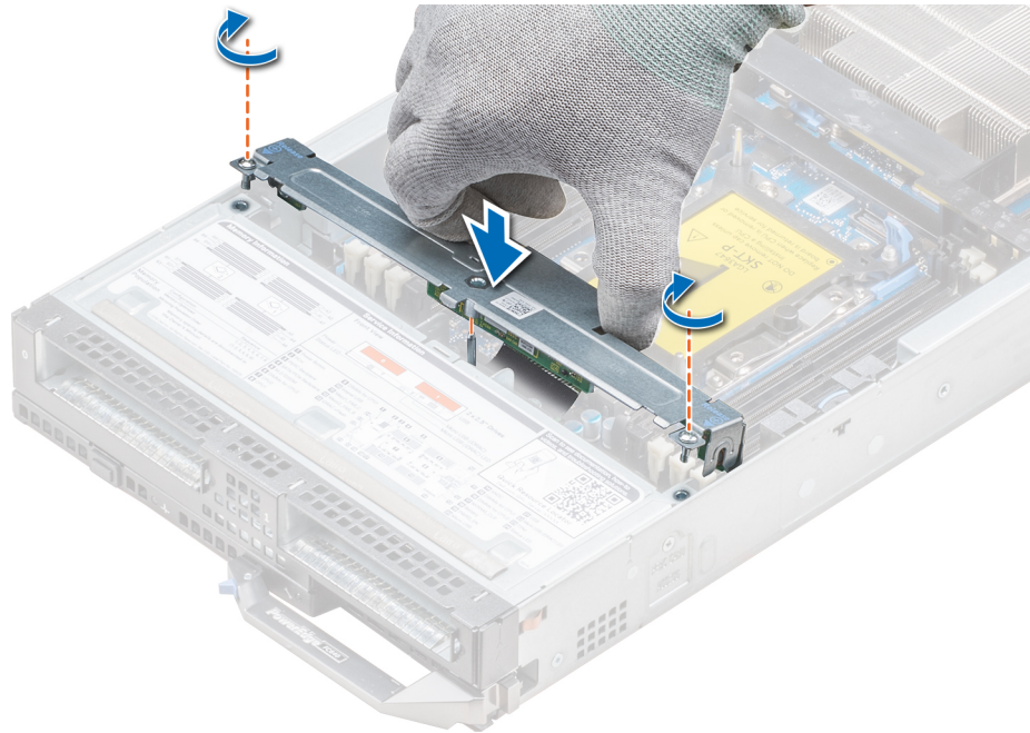
図 25. ドライブ バックプレーンの取り付け
