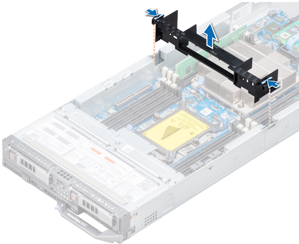
図 12. エアフローカバーの取り外し
