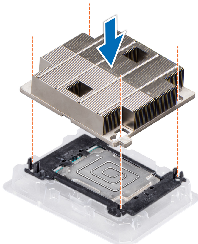
図 34. ヒートシンクをプロセッサに取り付けます。
