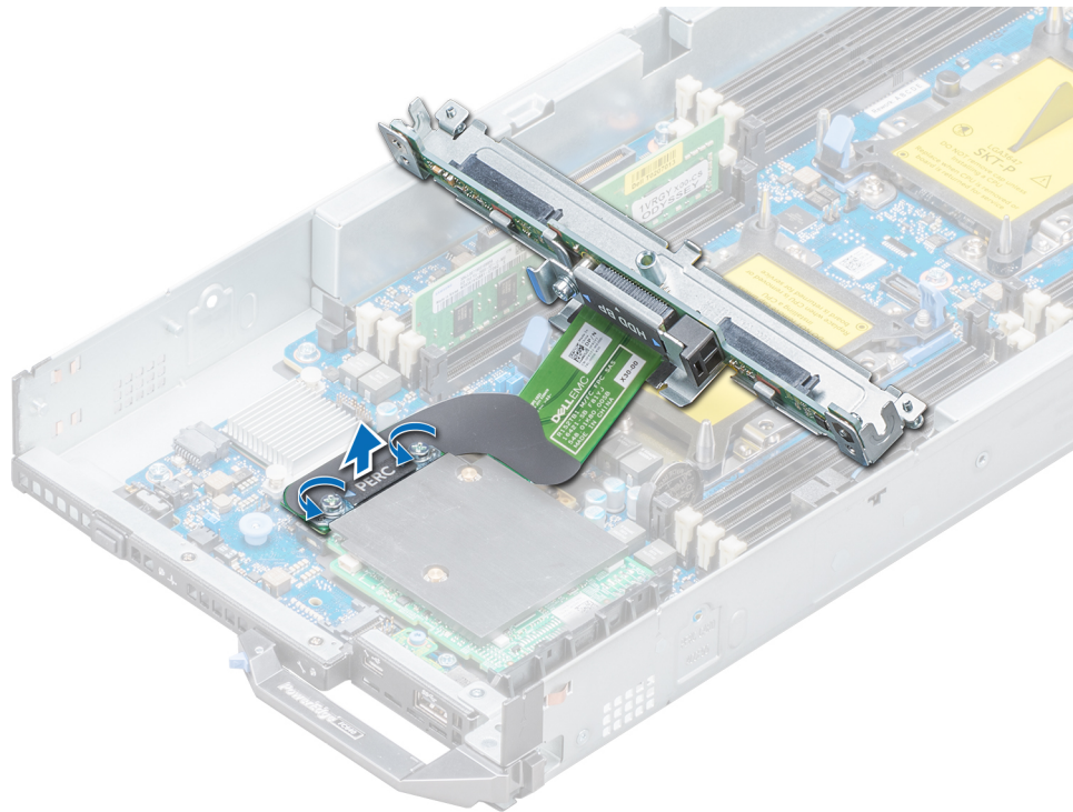
図 42. ストレージコントローラカードの取り外し
