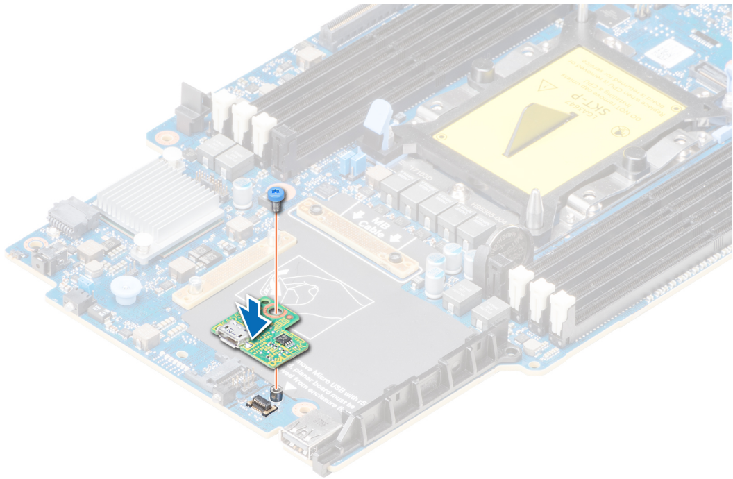
図 61. rSPI カードの取り付け
