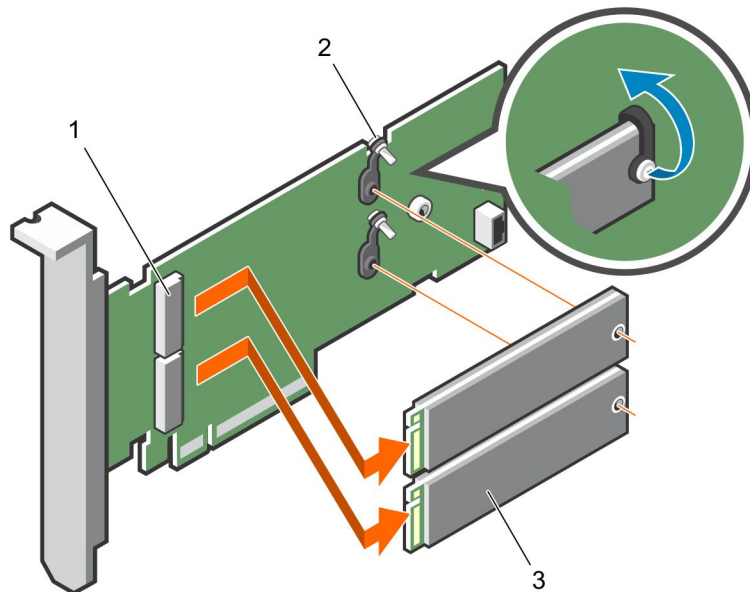
図 36. M.2 SSD モジュールの取り外し
