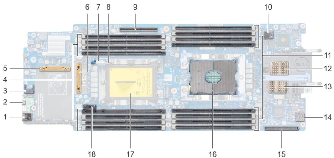
図 62. システム基板のコネクタ
