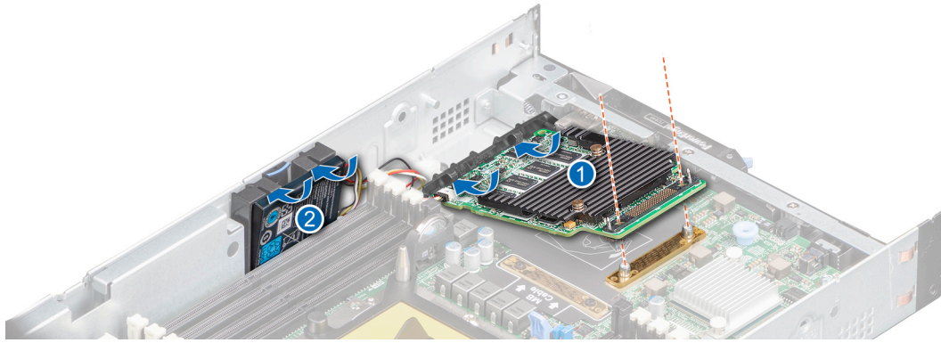
図 46. RAID コントローラー バッテリーの取り付け
