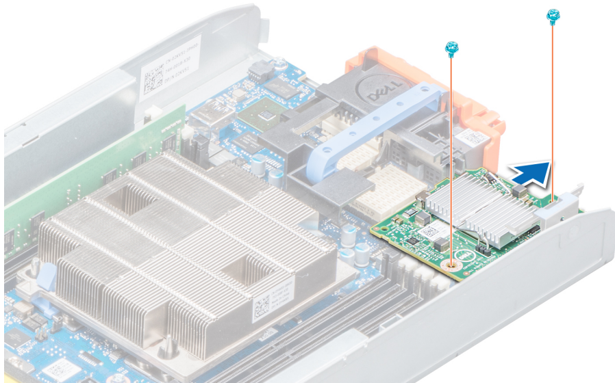
図 38. ネットワークドーターカードの取り外し
