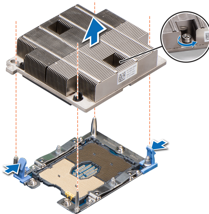
図 29. プロセッサとヒートシンクモジュールの取り外し
