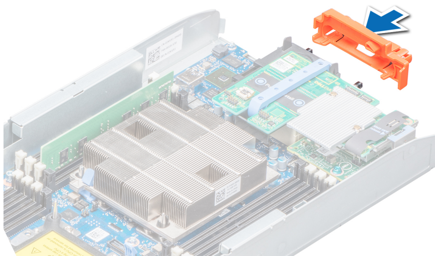
図 8. I/O コネクタカバーの取り付け
