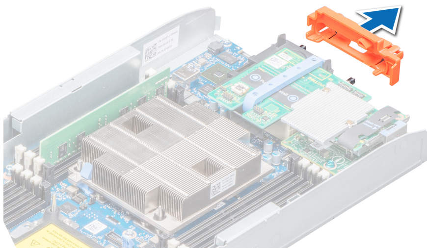
図 9. I/O コネクタカバーを取り外します。
