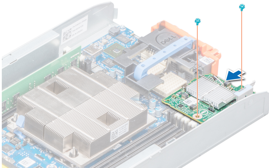
図 39. ネットワーク daughter カードの取り付け
