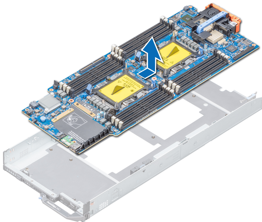
図 57. システム基板の取り外し
