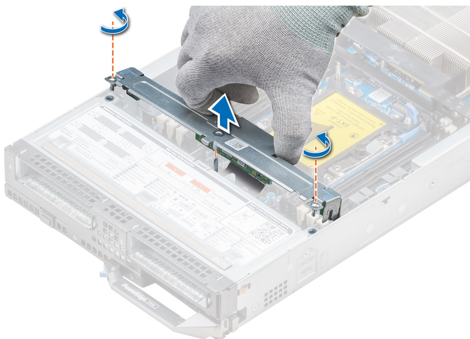
図 22. ドライブ バックプレーンの取り外し
