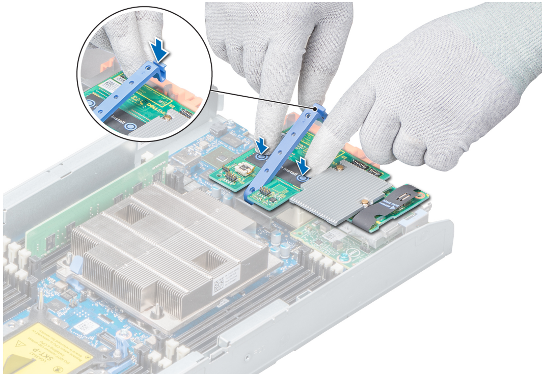
図 41. PCIe メザニンカードの取り付け
