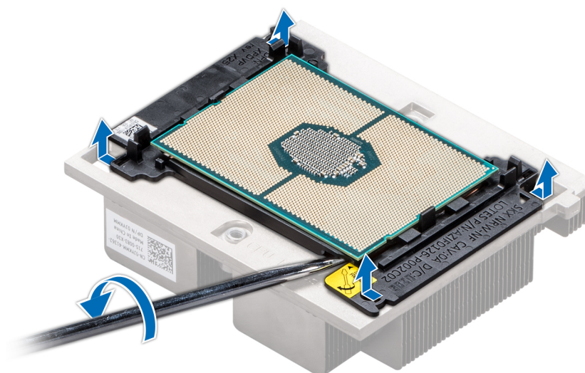
図 30. プロセッサブラケットを緩める
