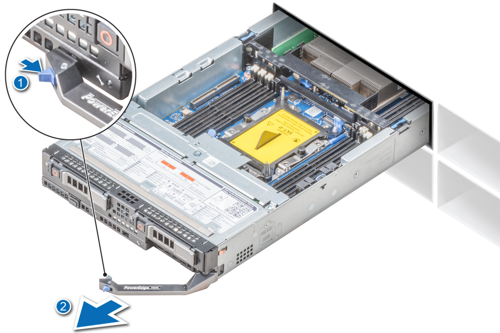
図 7. エンクロージャからのシステムの取り外し
