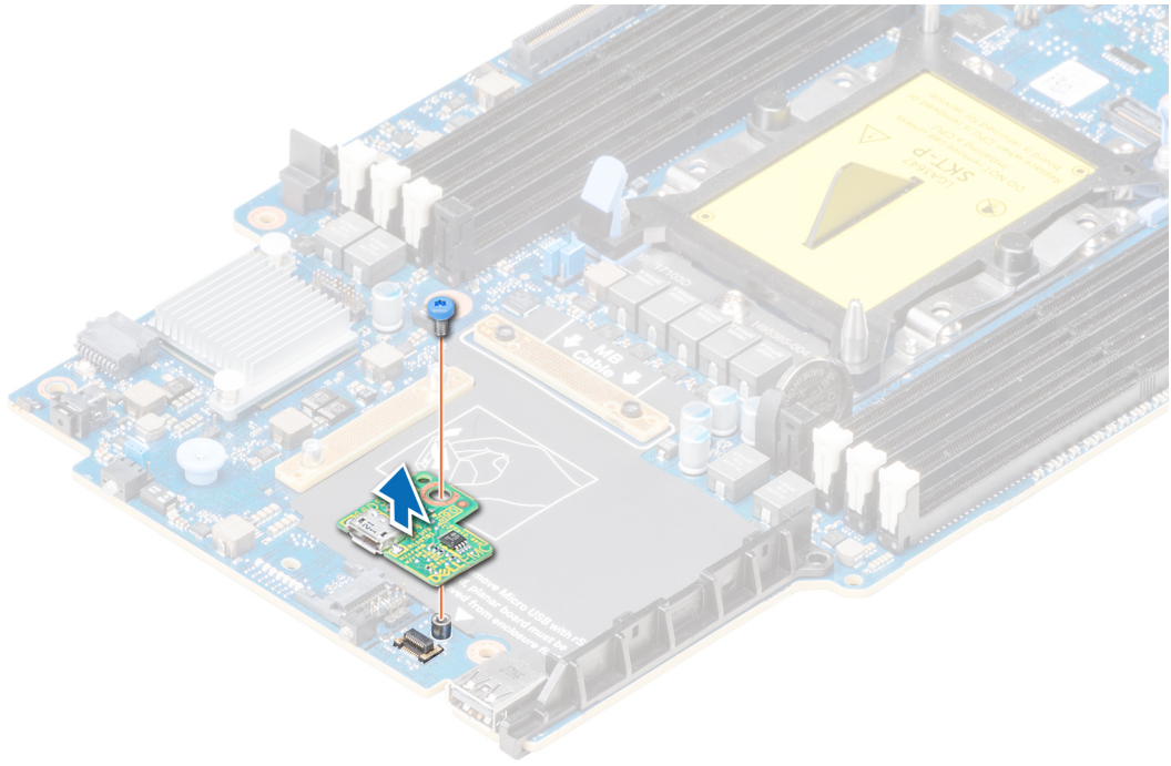
図 60. rSPI カードの取り外し
