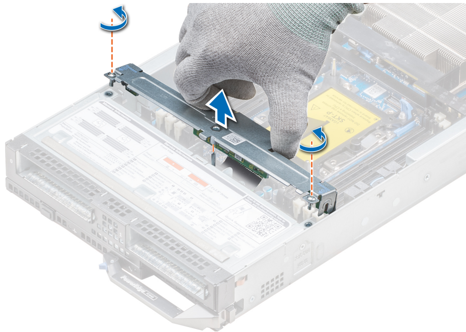
Figure 22. Retrait du fond de panier de disque
