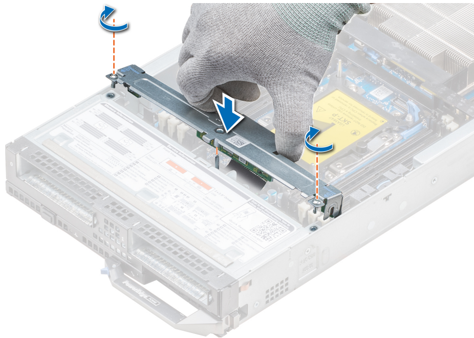
Figure 25. Installation du fond de panier de disque
