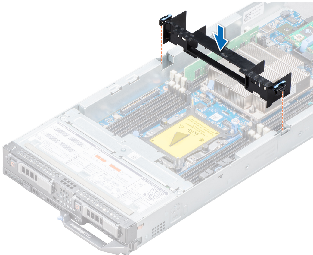
Figure 13. Installation du carénage d'aération
