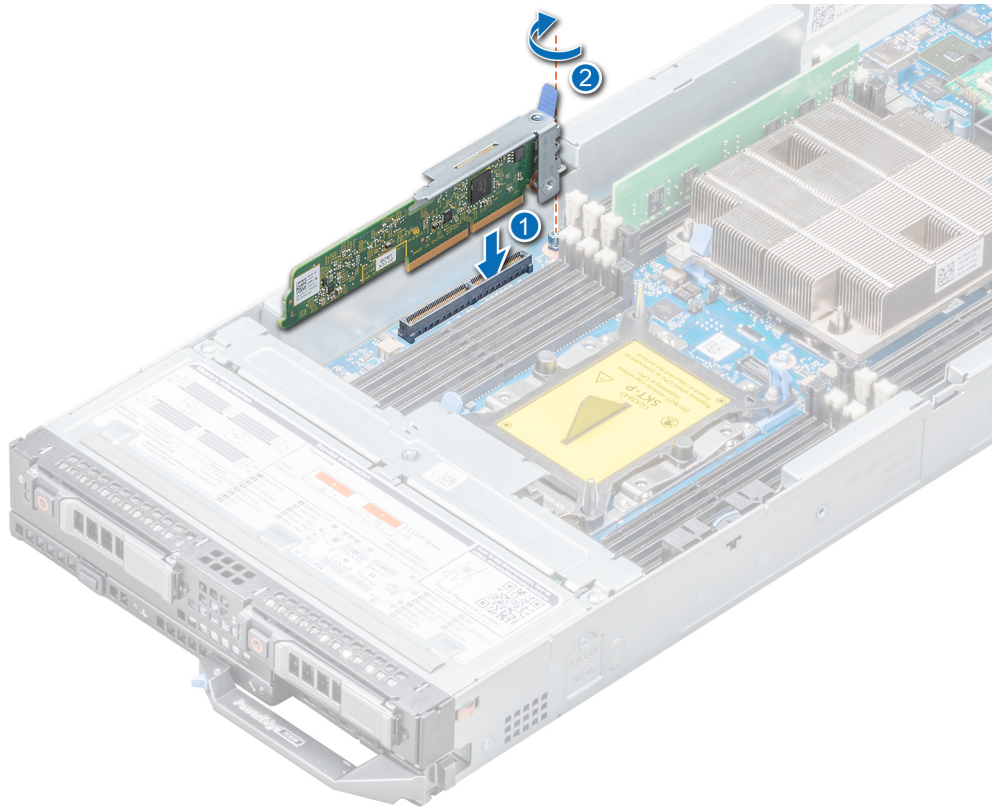
Figure 55. Installation du module IDSDM optionnel
