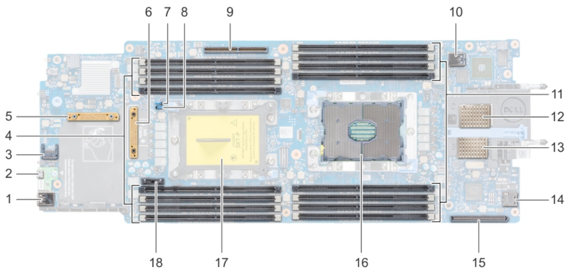
Figure 62. Connecteurs de carte système
