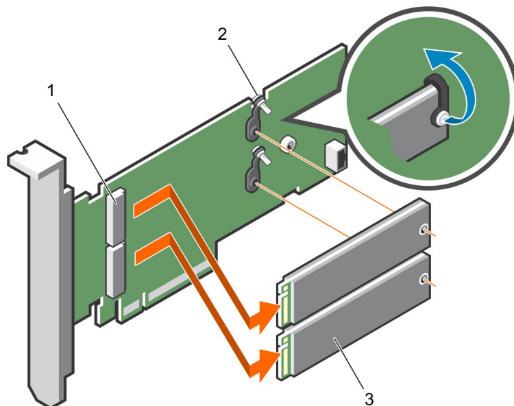
Figure 36. Retrait du module SSD M.2
