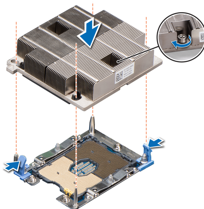
Figure 35. Installation d'un module de processeur et de dissipateur de chaleur
