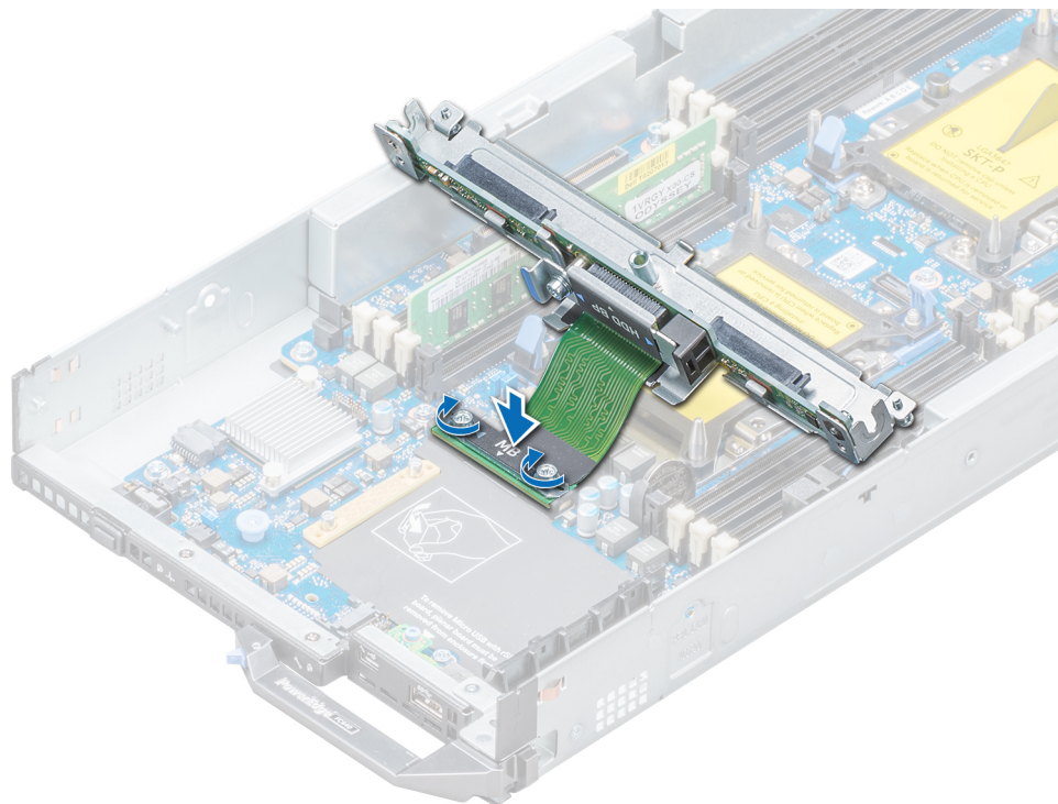
Figure 24. Fixation du câble du fond de panier
