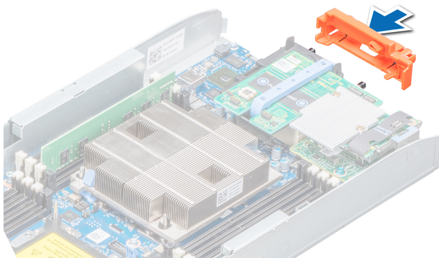
Figure 8. Installation du cache de connecteur d'E/S.
