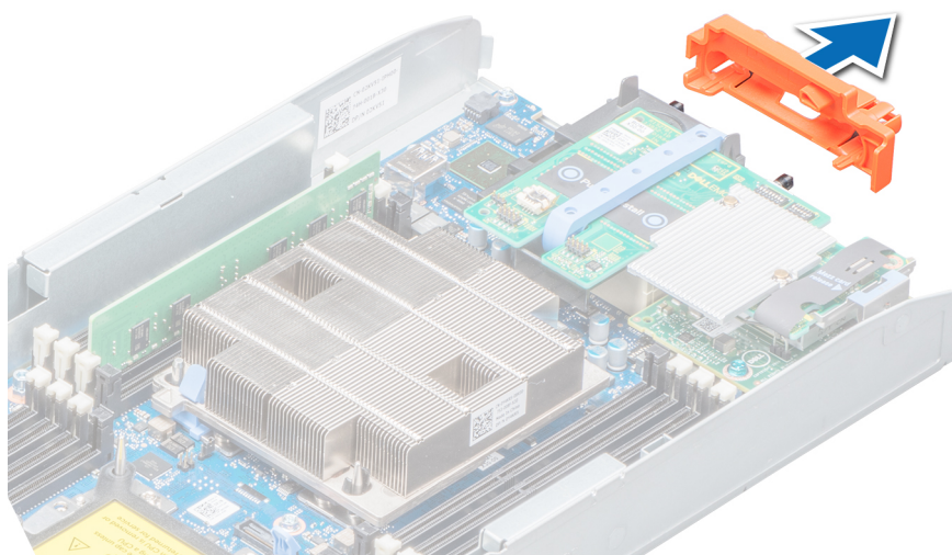
Figure 9. Retrait du cache de connecteur d'E/S.
