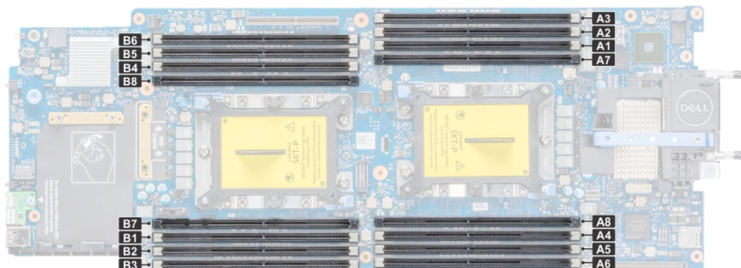
Figure 26. Vue du dessus du système
