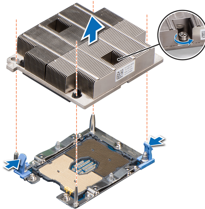
Figure 29. Retrait du module du processeur et du dissipateur de chaleur
