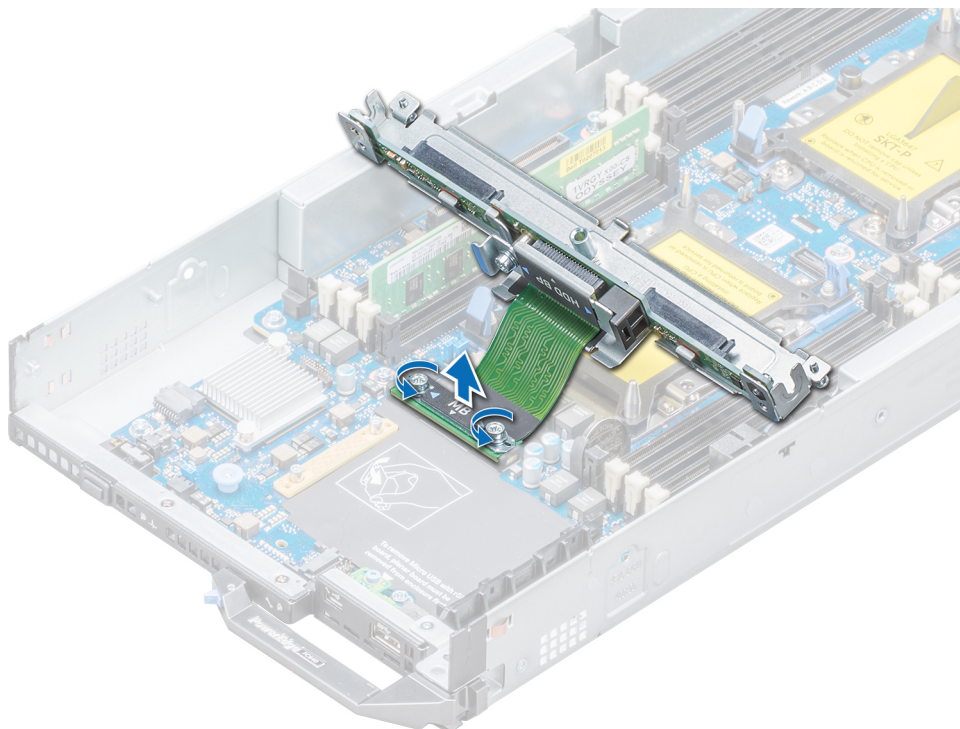
Figure 23. Retrait du câble du fond de panier de disque
