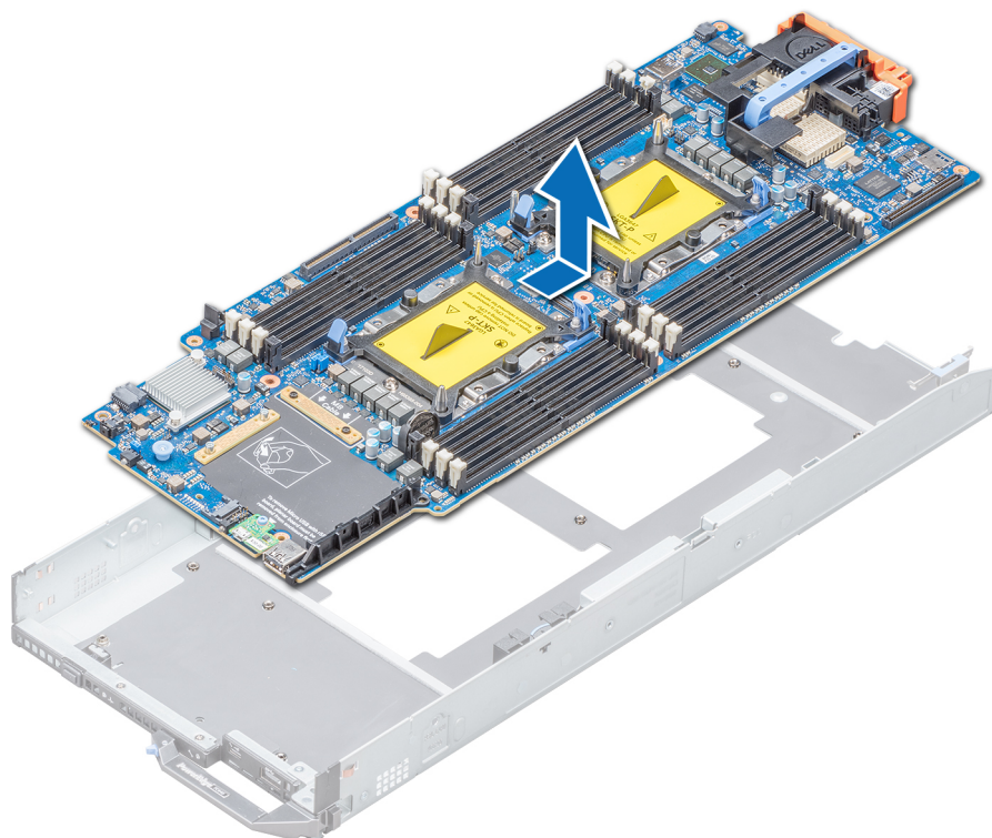
Figure 57. Retrait de la carte système
