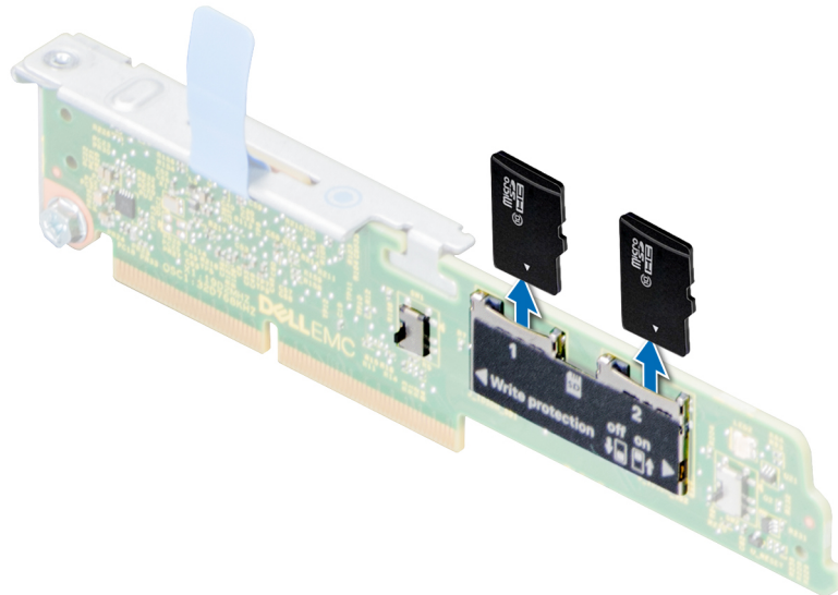
Figure 52. Retrait de la carte micro SD interne
