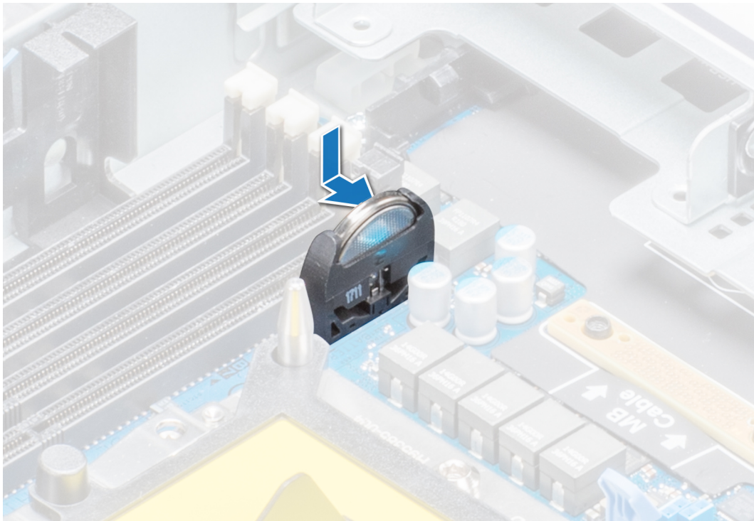
Figure 49. Installation de la pile du système
