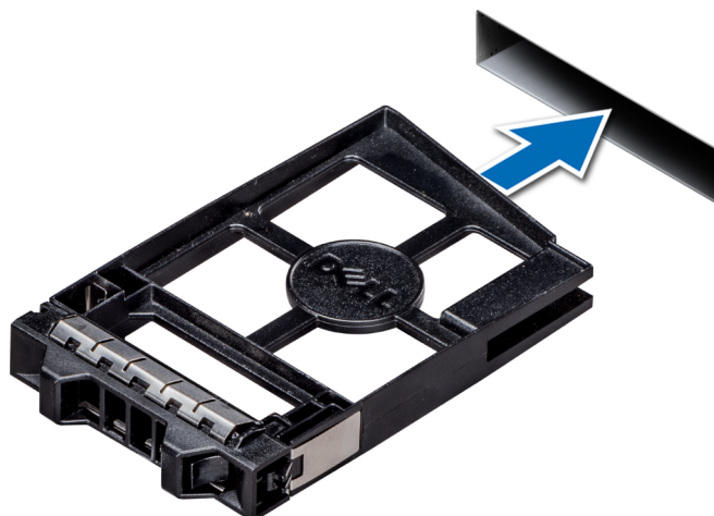
Ilustración 15. Instalación de una unidad de relleno
