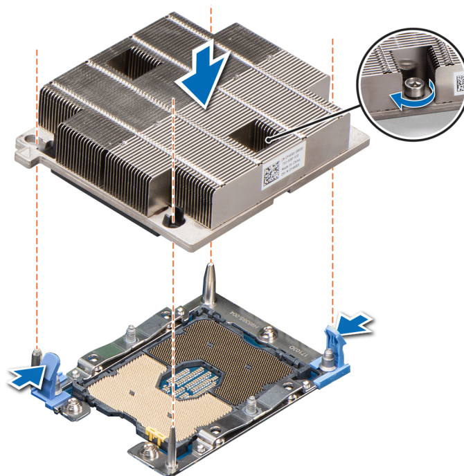
Ilustración 35. Instalación del módulo del procesador y el disipador de calor
