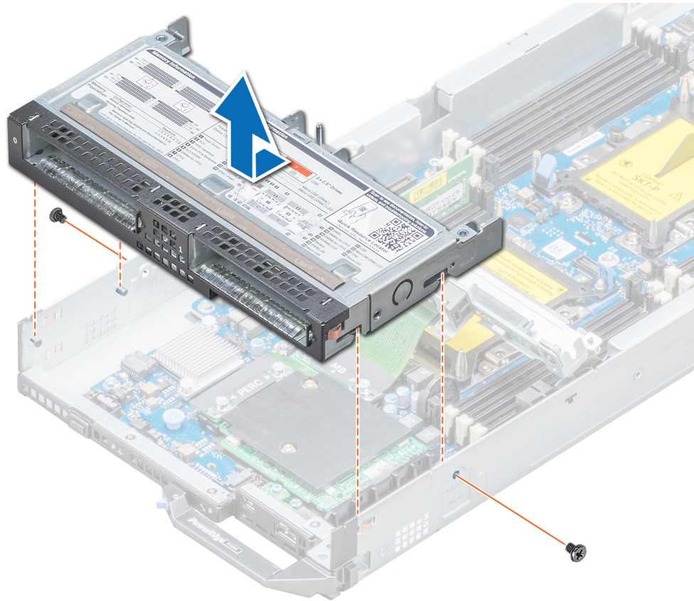
Ilustración 20. Extracción de la caja de la unidad
