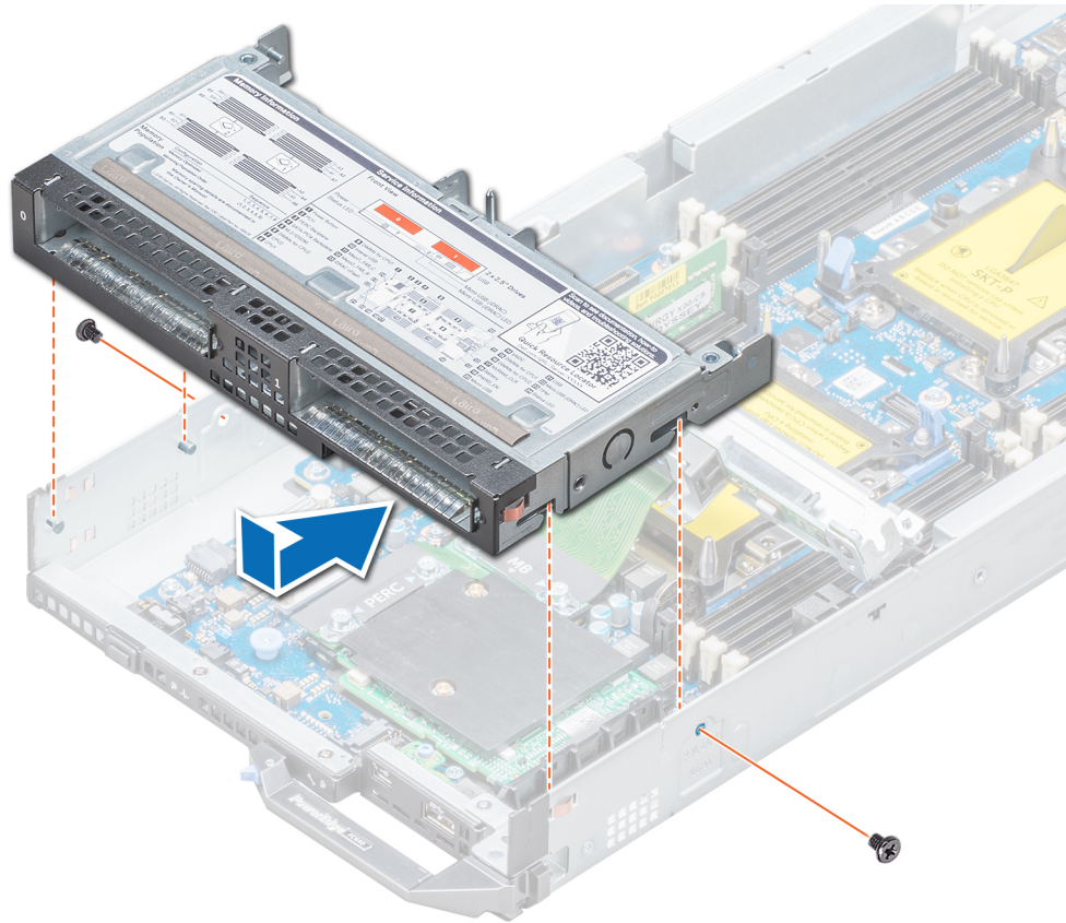
Ilustración 21. Instalación de la caja de la unidad de disco duro.
