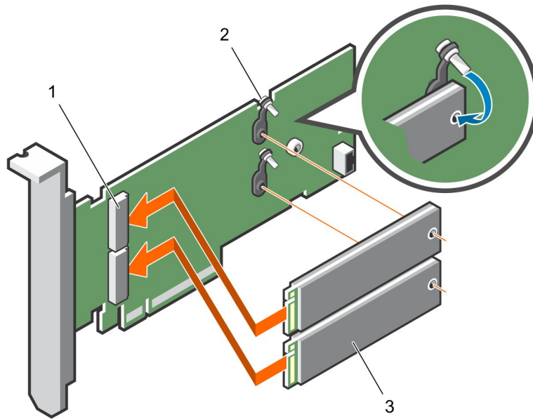
Ilustración 37. Instalación del módulo de SSD M.2
