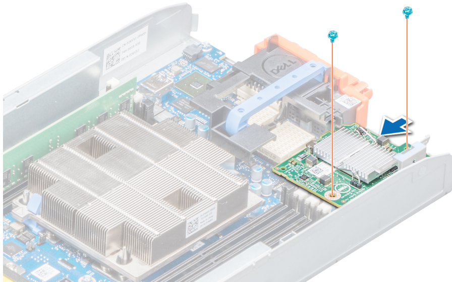
Ilustración 39. Instalación de la tarjeta secundaria de red
