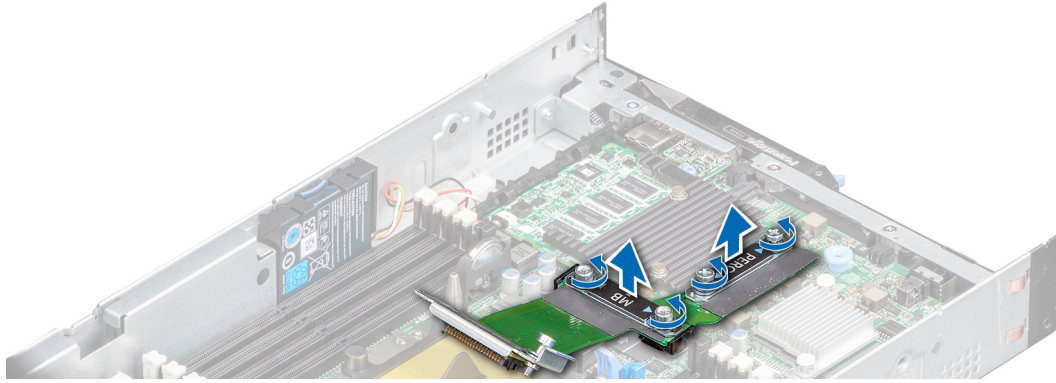
Ilustración 44. Extracción del conector del cable de la unidad
