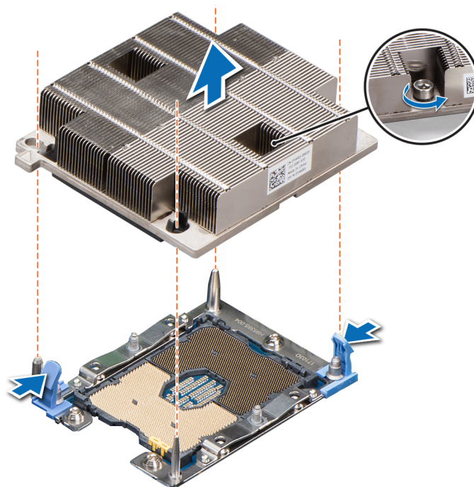
Ilustración 29. Extracción del módulo del procesador y el disipador de calor
