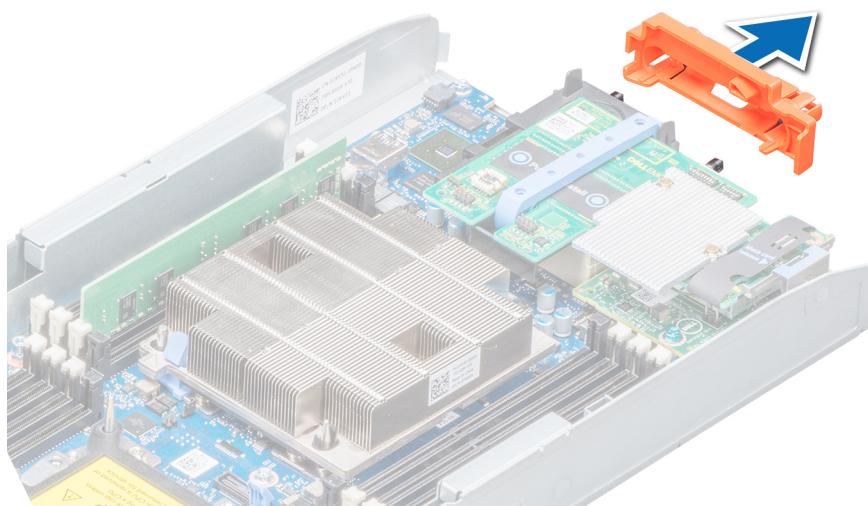
Ilustración 9. Extracción de la cubierta del conector de E/S.
