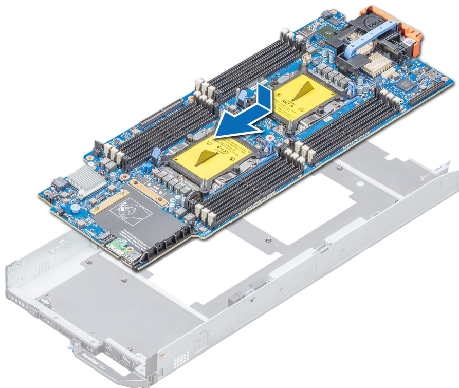
Ilustración 58. Instalación de la placa base
