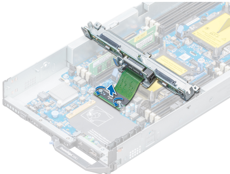
Ilustración 23. Extracción del cable del plano posterior de la unidad de disco duro
