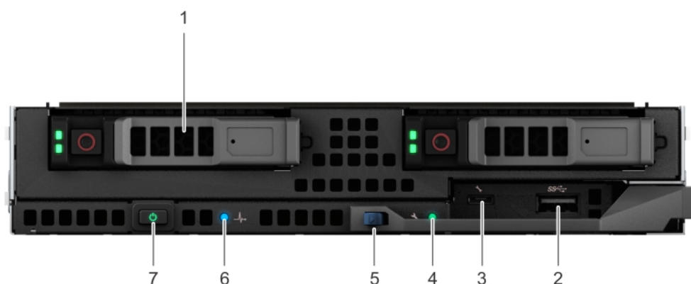
Ilustración 1. Vista frontal del sistema
