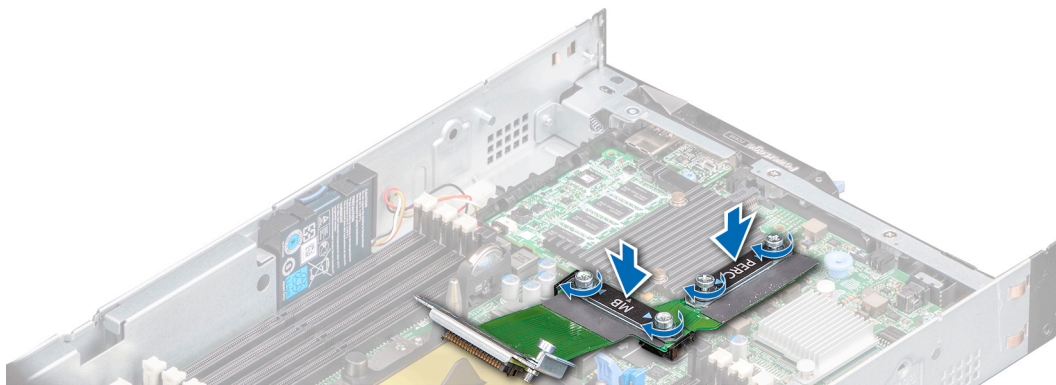
Ilustración 47. Instalación del conector del cable de la unidad
