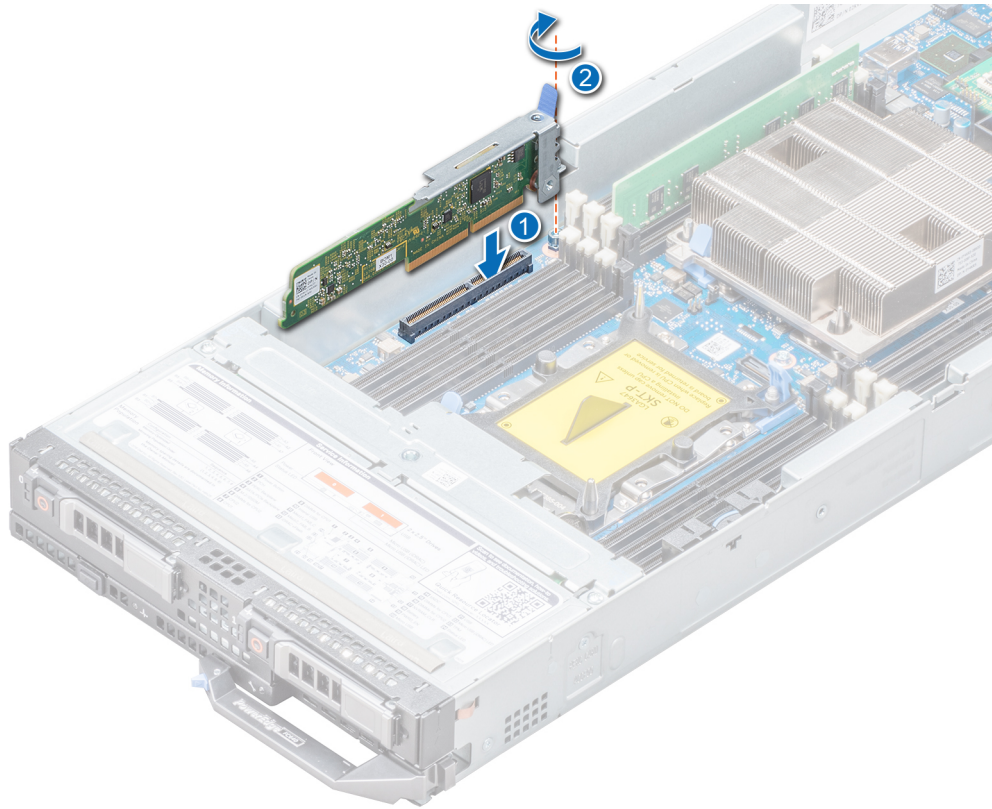
Ilustración 55. Instalación del módulo IDSDM opcional
