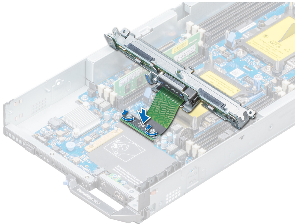
Ilustración 24. Fijación del cable del plano posterior
