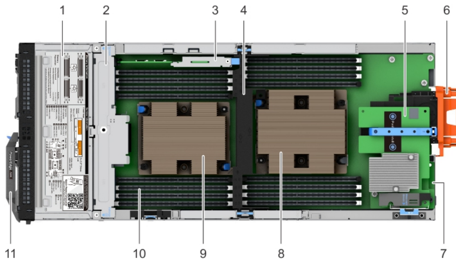
Ilustración 11. Interior del sistema
