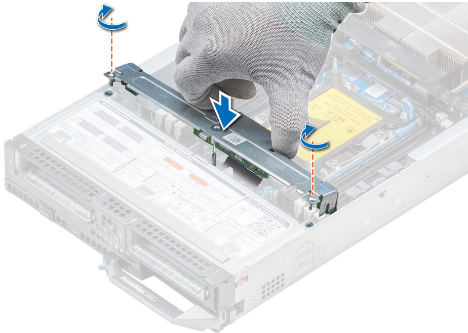
Ilustración 25. Instalación del plano posterior de la unidad de disco duro
