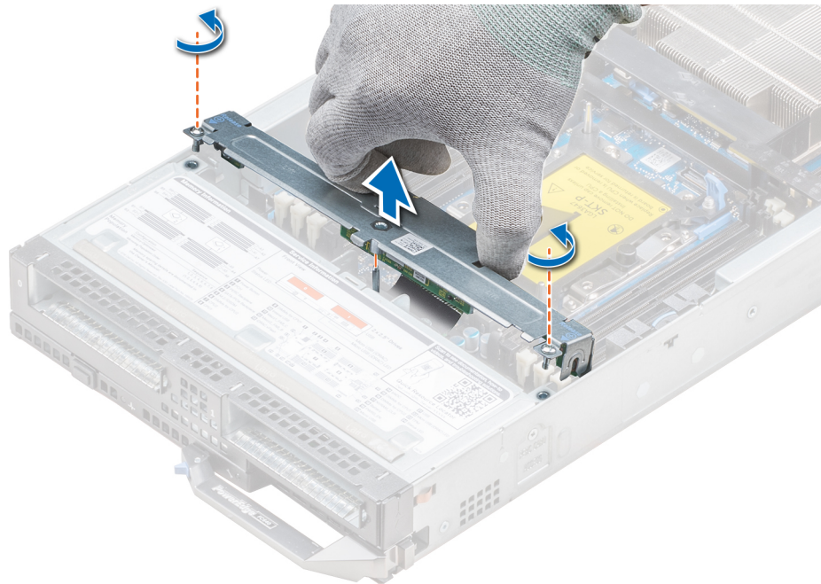
Ilustración 22. Extracción del plano posterior de la unidad de disco duro
