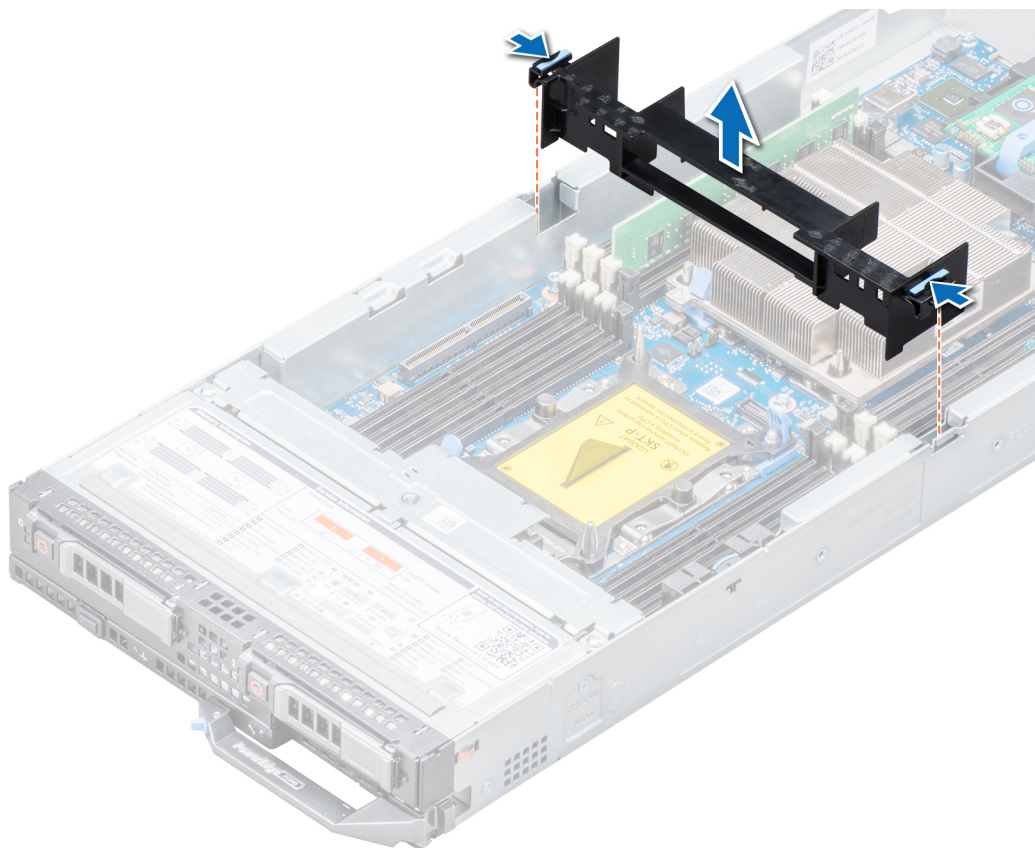
Ilustración 12. Extracción de la cubierta para flujo de aire
