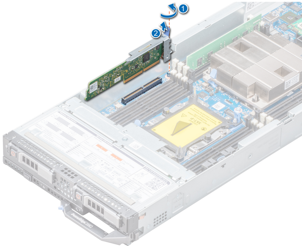
Ilustración 54. Extracción del módulo IDSDM opcional
