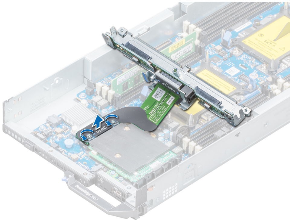
Ilustración 42. Extracción de la tarjeta controladora de almacenamiento
