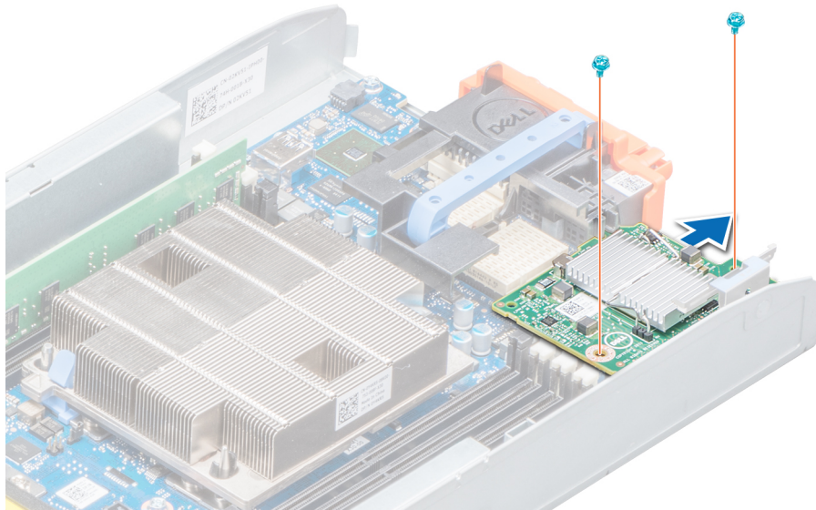
Ilustración 38. Extracción de la tarjeta secundaria de red
