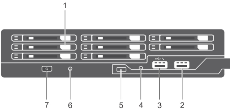
图 3: 前面板功能部件 — 1.8 英寸 SSD 系统
