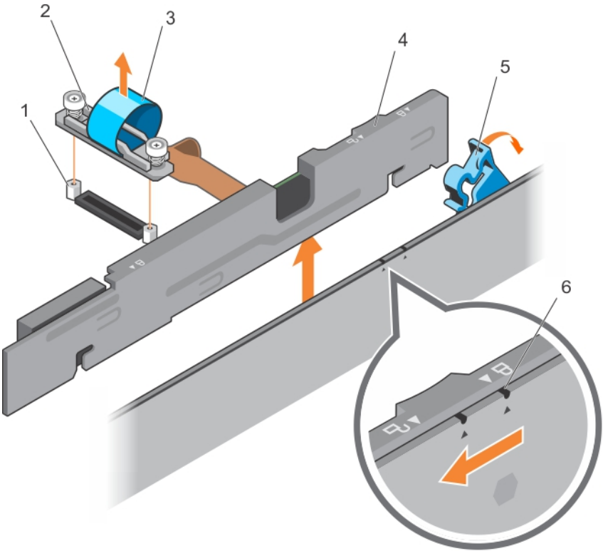
图 54: 卸下 PERC H730P 纤薄型卡
