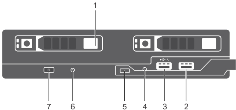
图 2: 前面板功能部件 — 2.5 英寸硬盘驱动器或 SSD 系统
