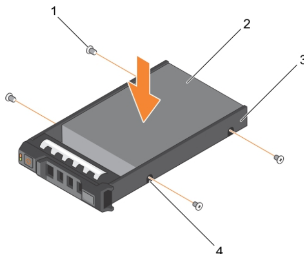
图 47: 在 2.5 英寸硬盘驱动器或 SSD 托盘中安装 2.5 英寸硬盘驱动器或 SSD
