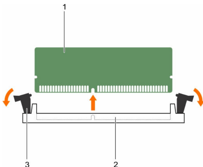
图 16: 卸下内存模块
