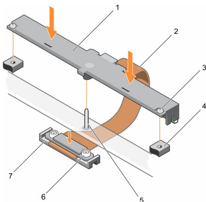
图 53: 安装硬盘驱动器或 SSD 背板
