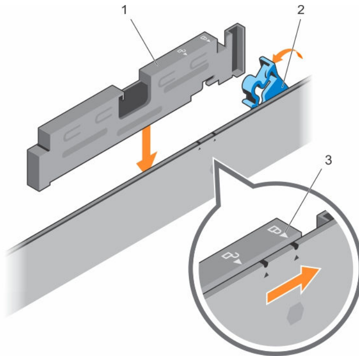
图 55: 安装 PERC H730P 纤薄型卡
