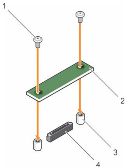
图 26: 安装可选 rSPI 卡
