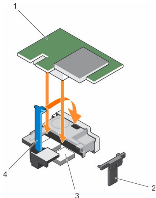
图 19: 安装 PCIe 夹层卡
