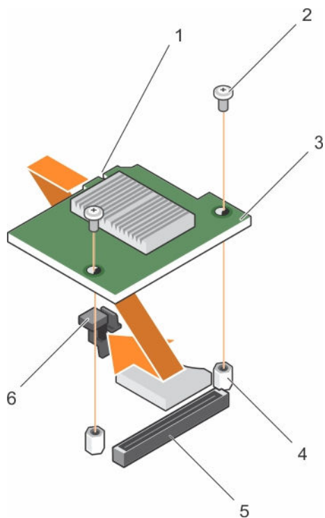
图 30: 安装 NDC
