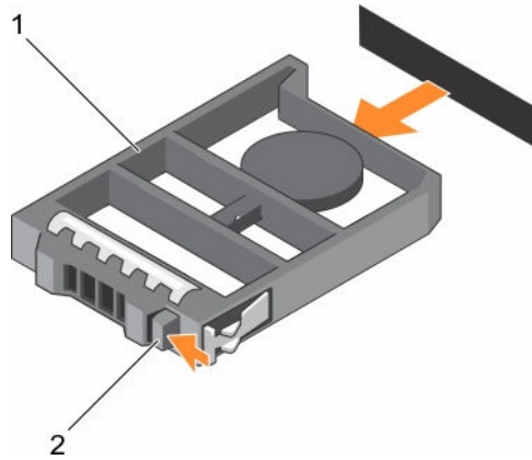
图 42: 卸下 2.5 英寸硬盘驱动器
