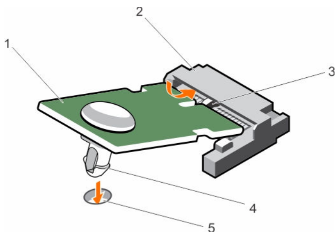
图 62: 安装 TPM
