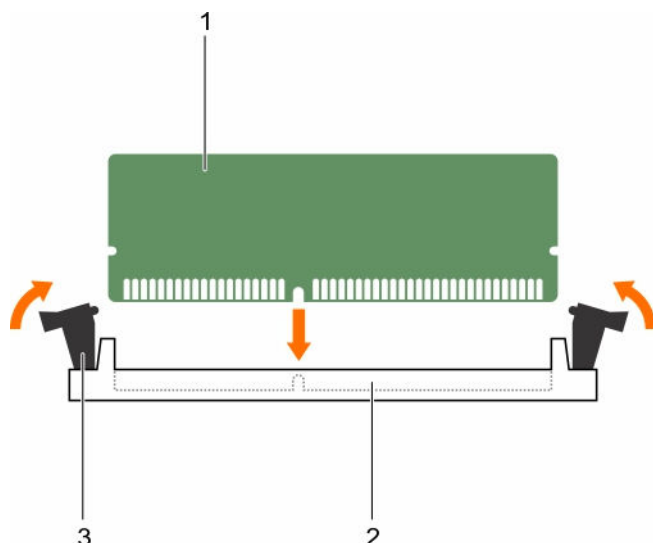
图 17: 安装内存模块
