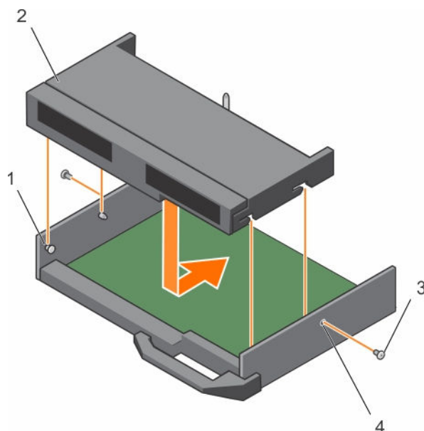
图 51: 安装硬盘驱动器或 SSD 固定框架
