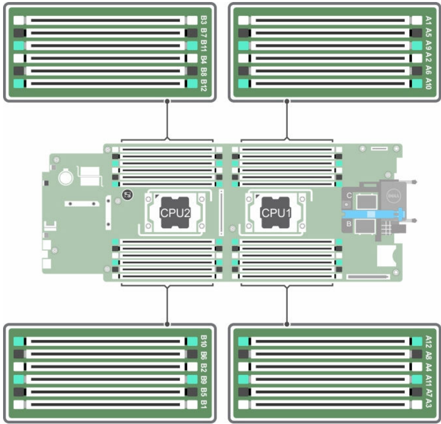
图 15: 内存插槽位置
