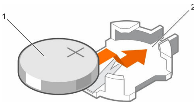
图 59: 安装 NVRAM 备用电池
