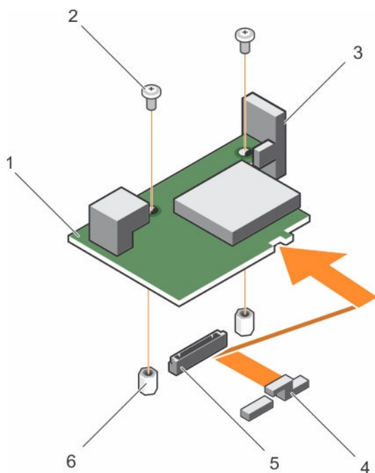
图 23: 卸下可选 IDSDM 卡
