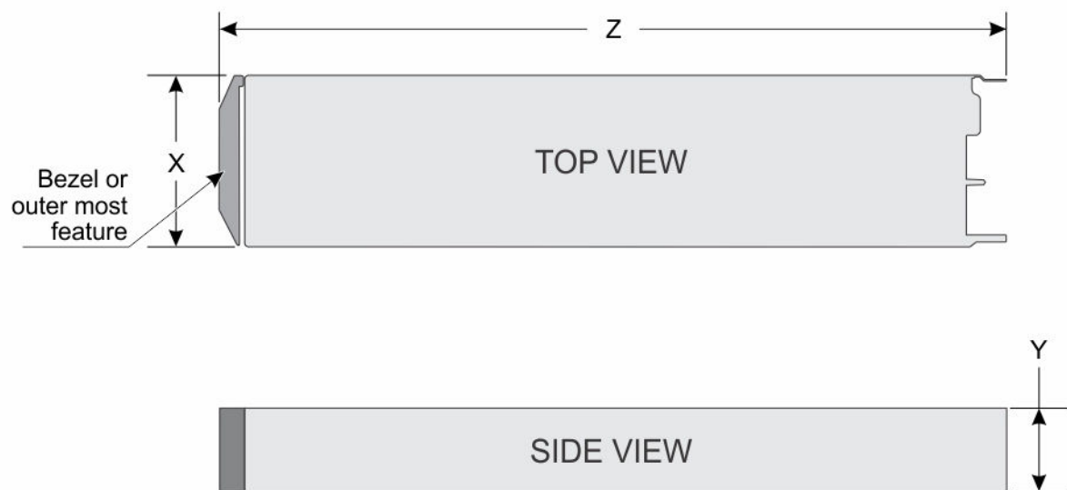
图 6: 机箱尺寸
