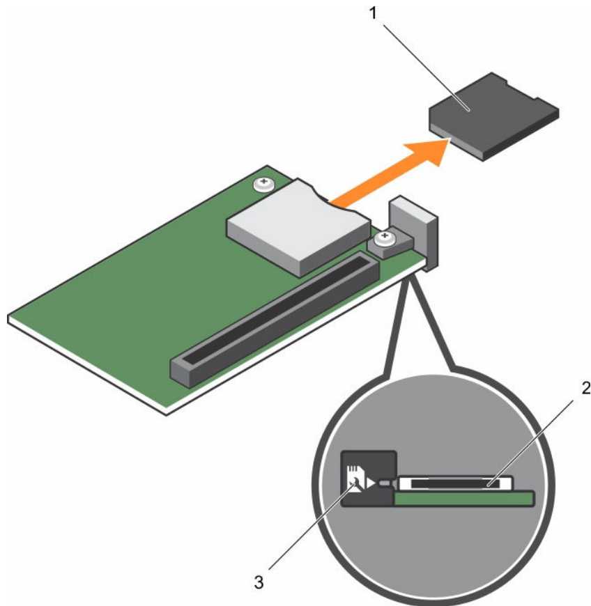
图 27: 装回 SD vFlash 卡
