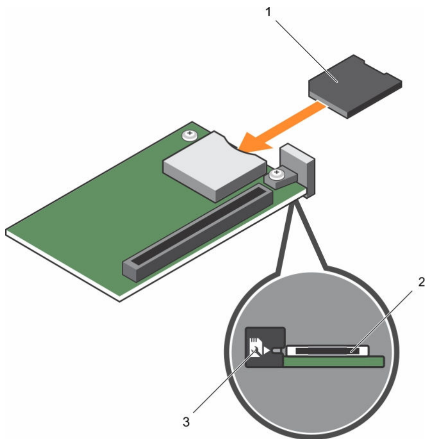
图 28: 安装 SD vFlash 卡
