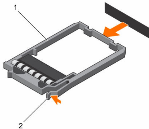
图 43: 卸下 1.8 英寸 SSD 挡片
