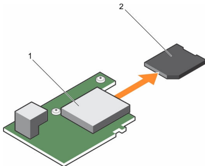
图 20: 装回 SD 卡
