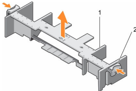
图 11: 卸下冷却导流罩
