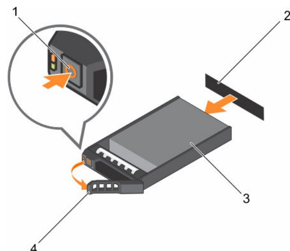
图 38: 卸下硬盘驱动器
