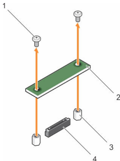
图 25: 卸下可选 rSPI 卡
