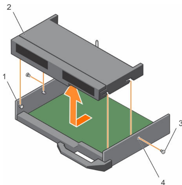
图 50: 卸下硬盘驱动器或 SSD 固定框架
