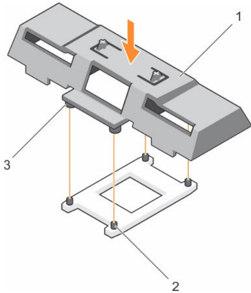
图 14: 安装处理器/DIMM 挡片
