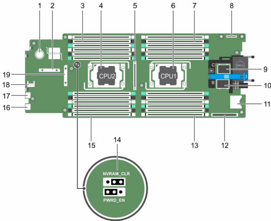
图 63: 系统板连接器
