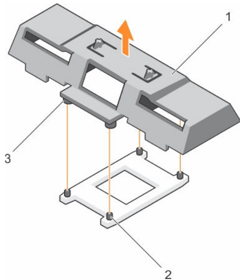
图 13: 卸下处理器或 DIMM 挡片
