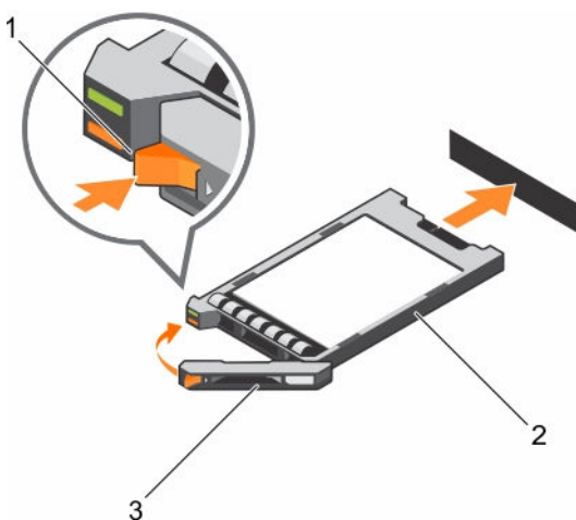
图 41: 安装 SSD
