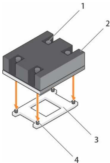
图 34: 安装散热器
