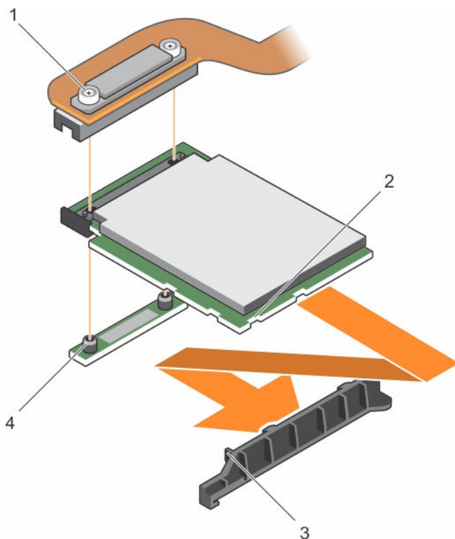
图 57: 安装 PCIe 扩展卡或存储控制器卡
