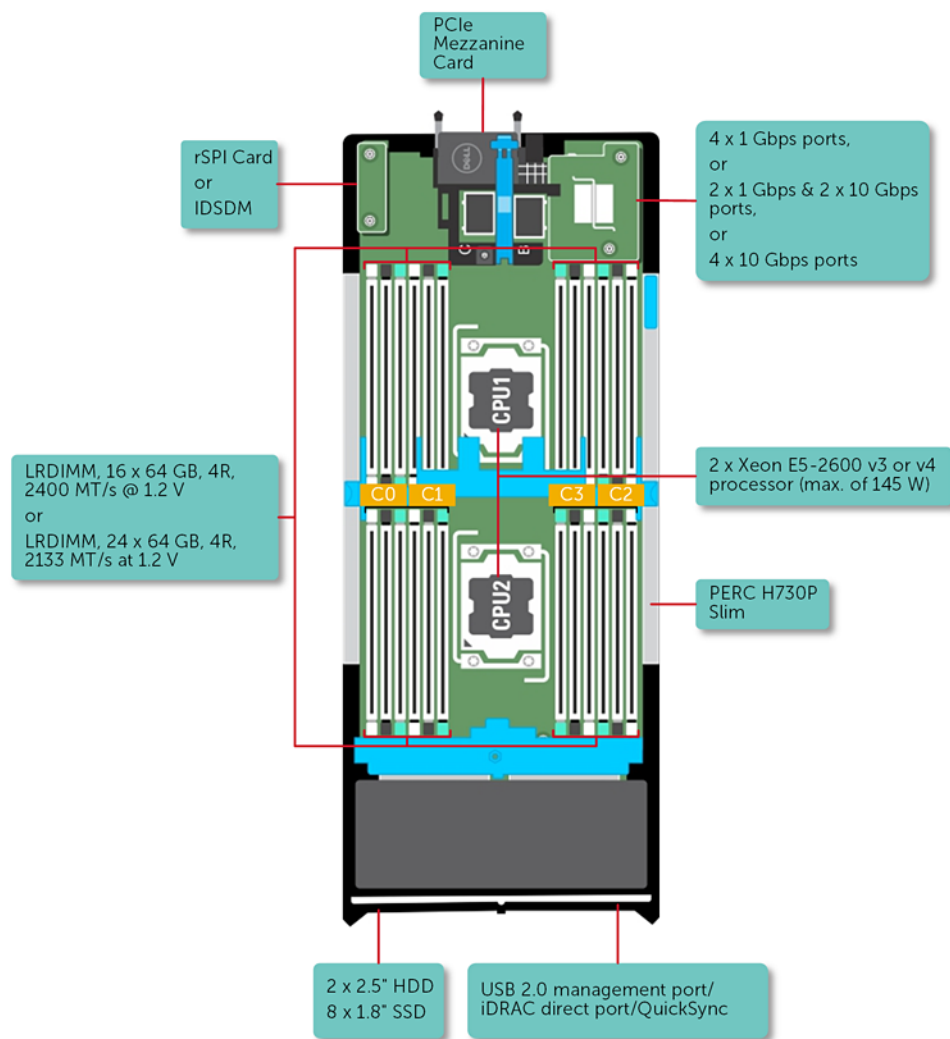
图 1: FC630 配置概览
