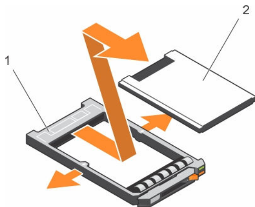
图 48: 从 1.8 英寸 SSD 托盘卸下 1.8 英寸 SSD
