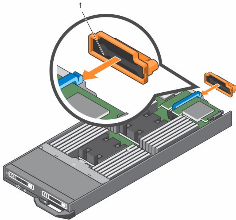
图 9: 安装底座
