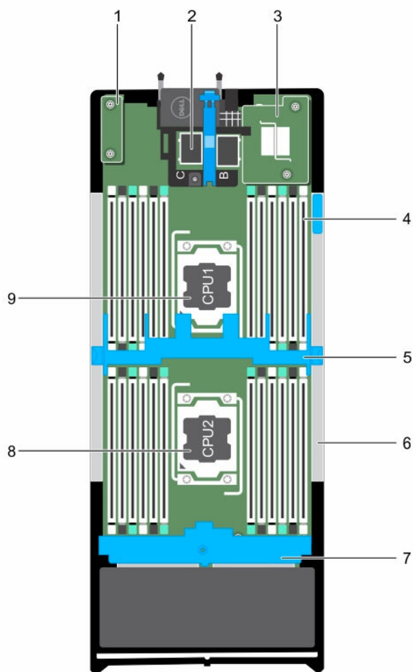
图 10: 底座内部组件
