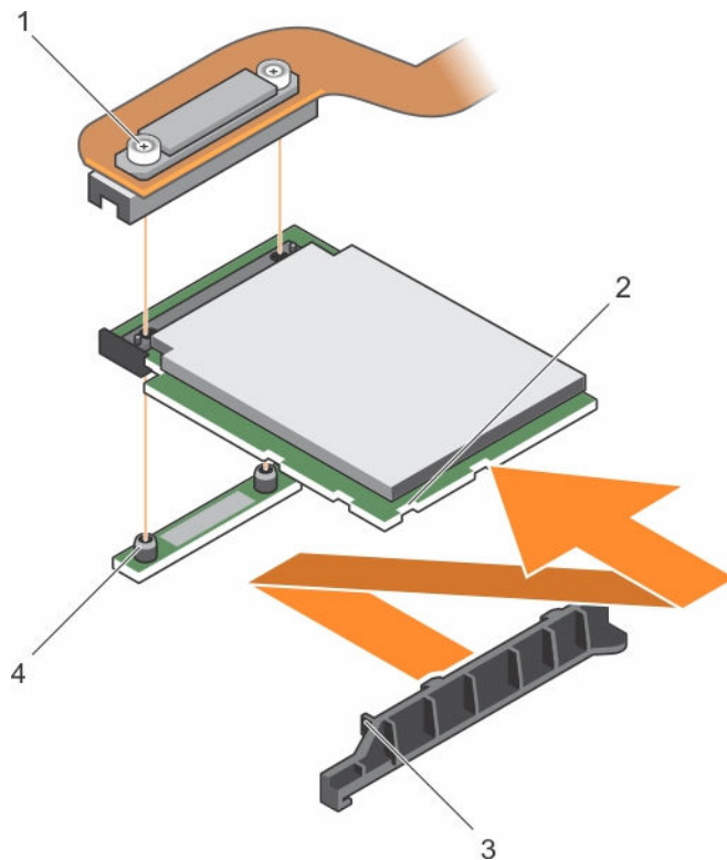
图 56: 卸下 PCIe 扩展卡或存储控制器卡
