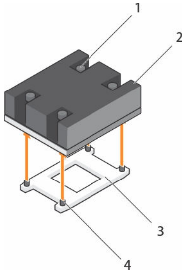
图 31: 卸下散热器
