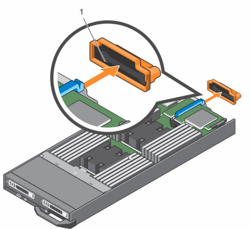
图 7: 卸下 I/O 连接器护盖
