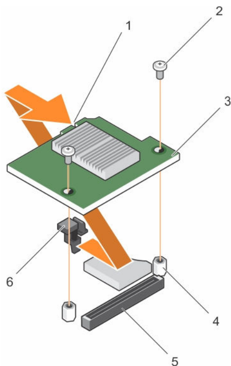
图 29: 卸下 NDC
