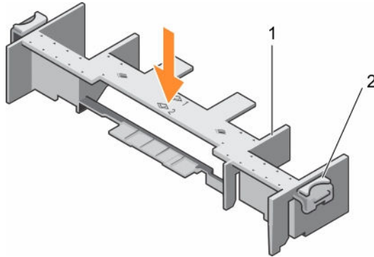
图 12: 安装冷却导流罩
