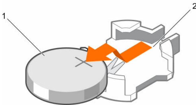
图 58: 卸下 NVRAM 备用电池
