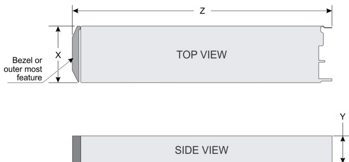
図 5. PowerEdge FC430 システムのシャーシ寸法
