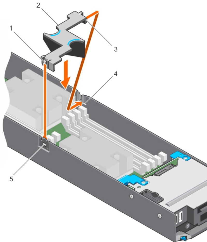
図 10. 冷却用エアフローカバーの取り付け
