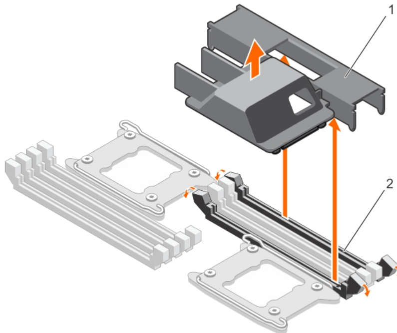
図 30. プロセッサダミー と DIMM ダミーの取り外し
