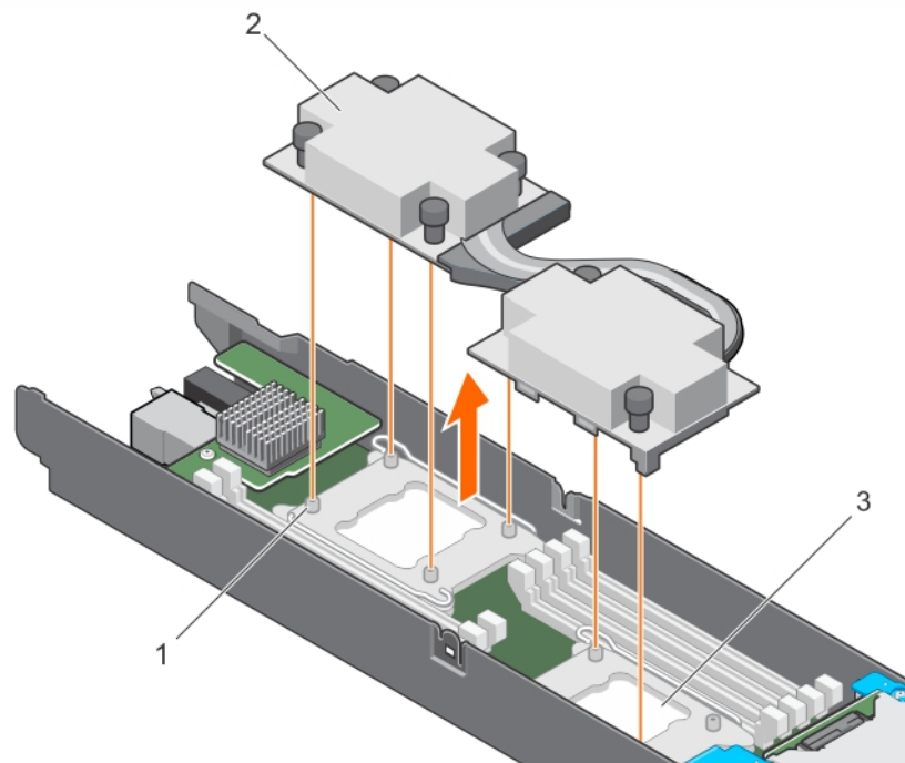
図 26. 140 W ヒートシンクの取り外し
