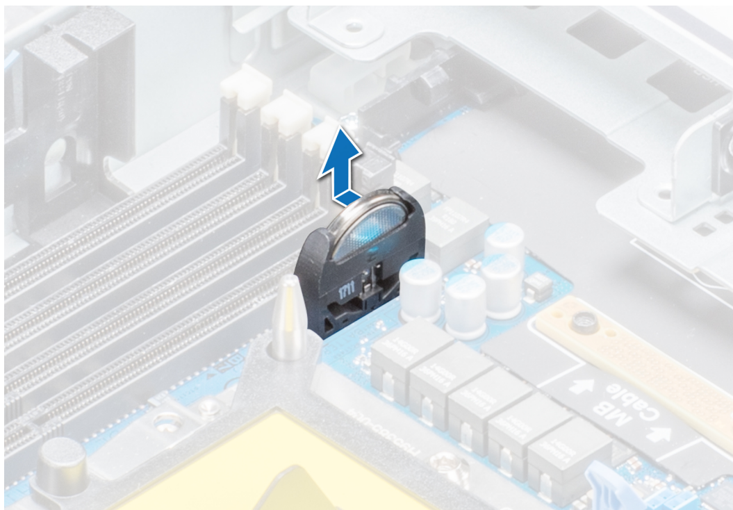
Figure 46. Retrait de la pile du système
