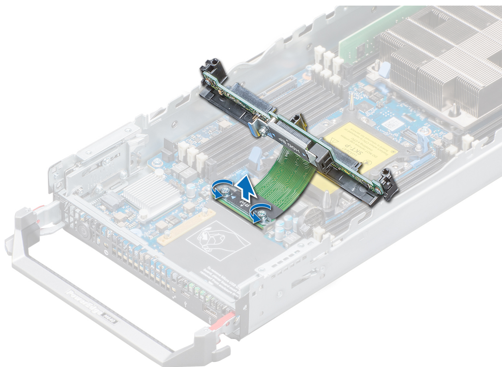
Figure 25. Retrait du câble de fond de panier
