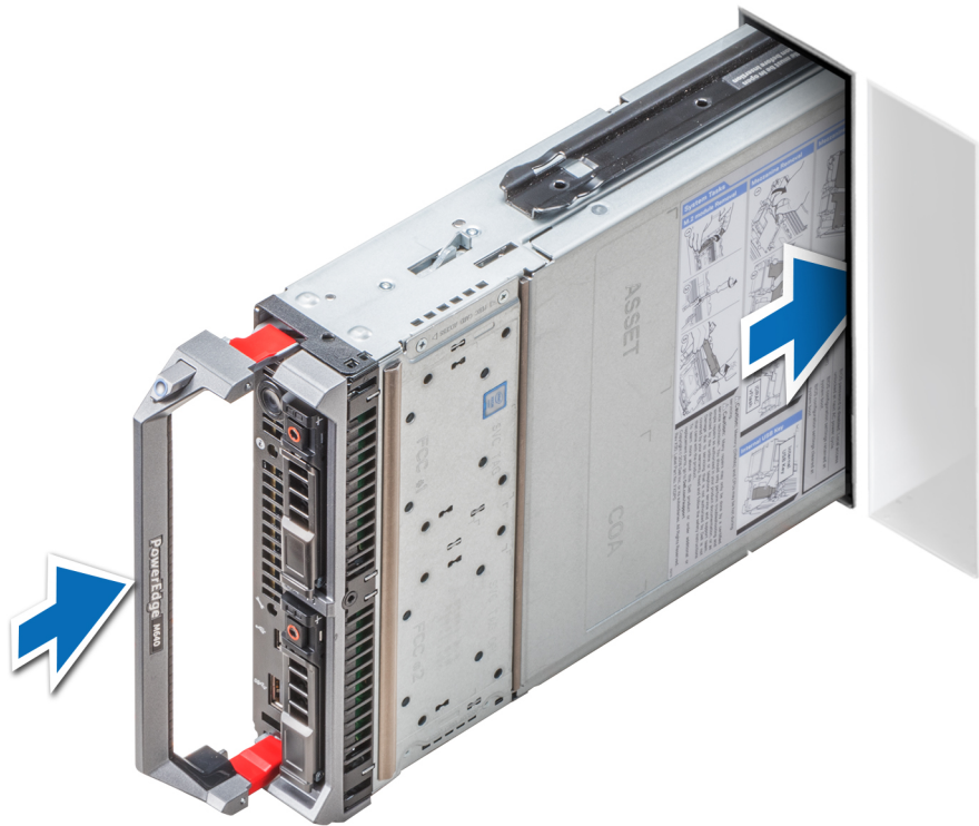
Figure 10. Installation du système dans le châssis
