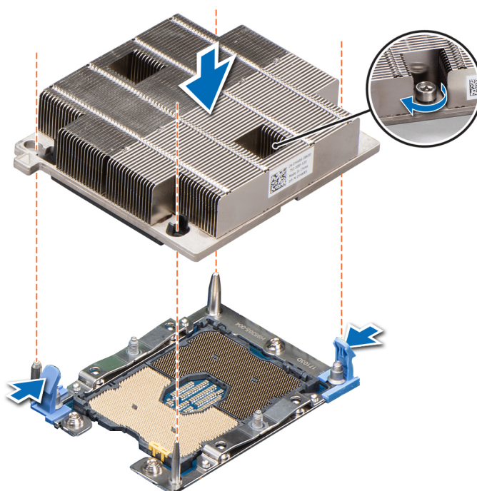
Figure 37. Installation d'un module de processeur et de dissipateur de chaleur
