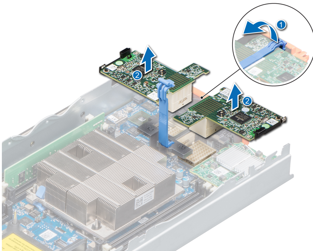
Figure 42. Retrait de la carte mezzanine PCIe
