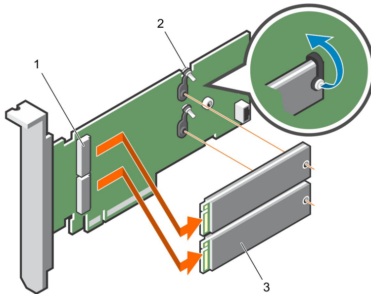
Figure 38. Retrait du module SSD M.2
