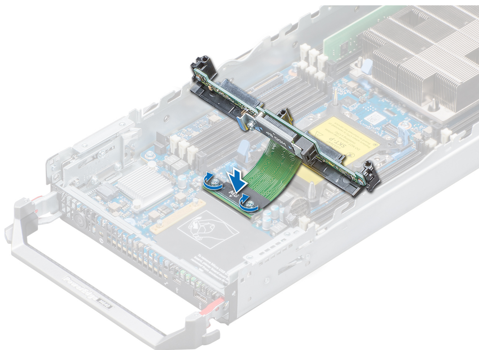
Figure 26. Installation du câble de fond de panier de disque
