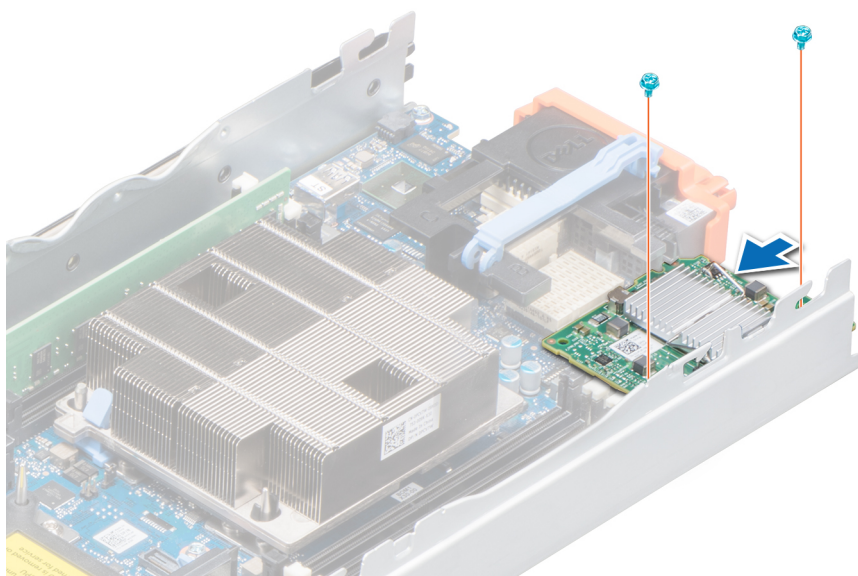
Figure 41. Installation de la carte fille réseau
