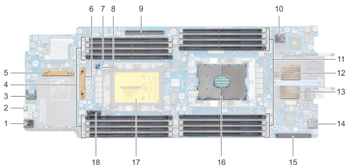
Figure 60. Connecteurs de carte système
