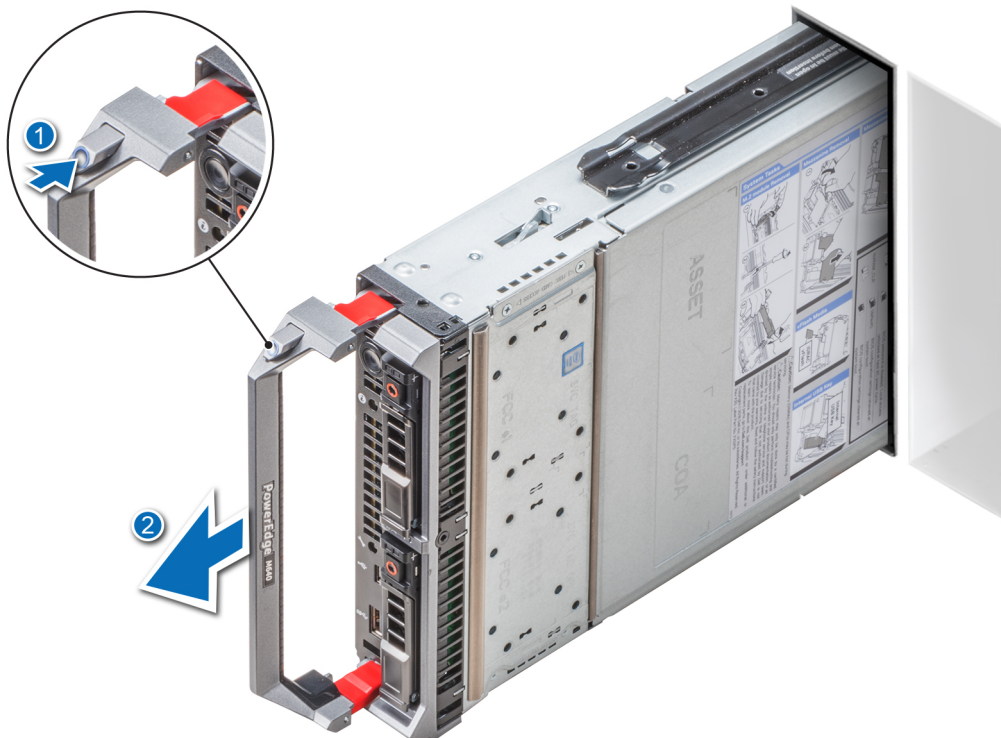
Figure 7. Retrait du système hors du châssis
