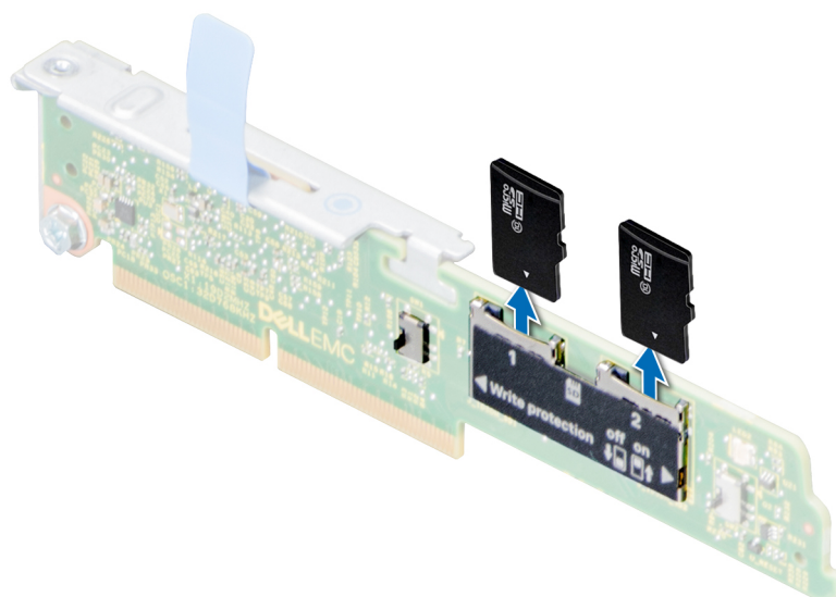
Figure 50. Retrait de la carte micro SD interne
