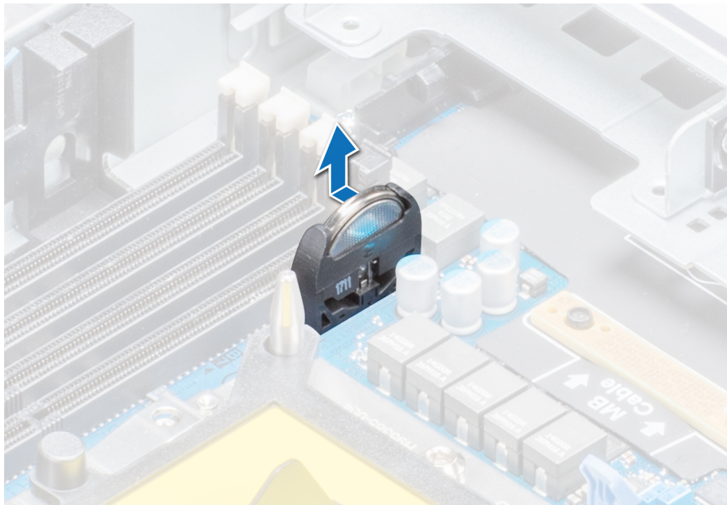
Ilustración 46. Extracción de la batería del sistema
