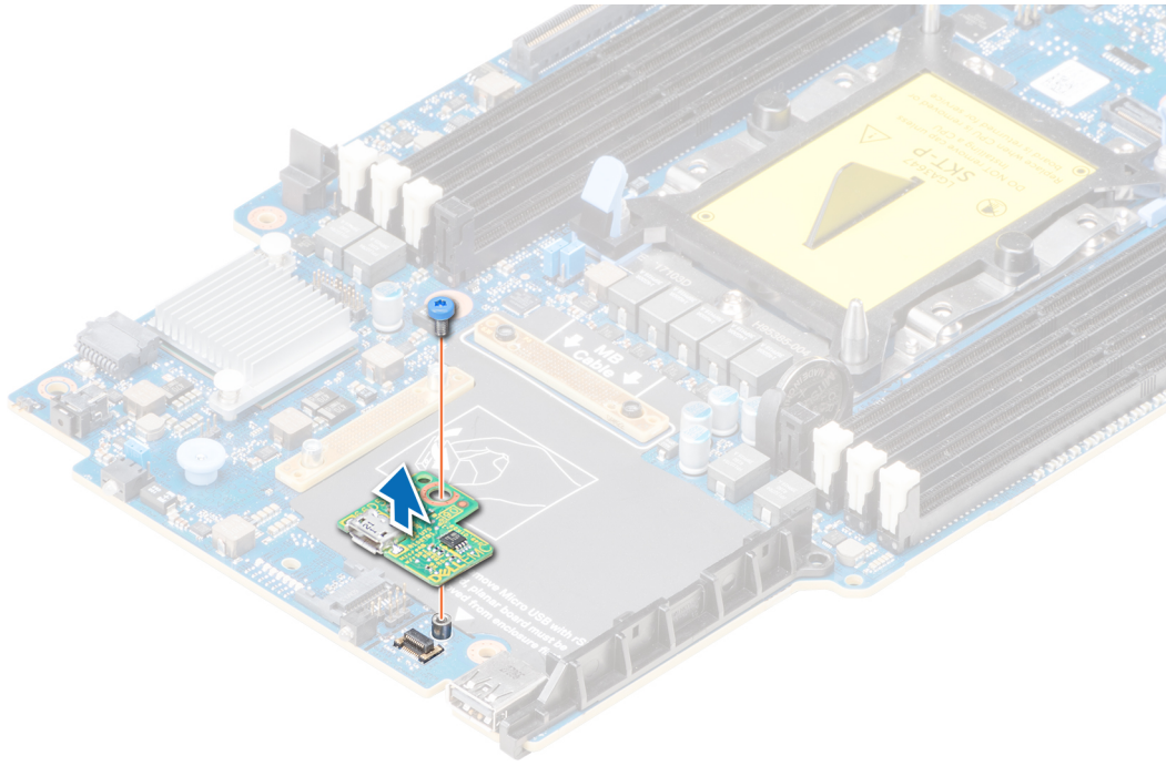
Ilustración 58. Extracción de la tarjeta rSPI
