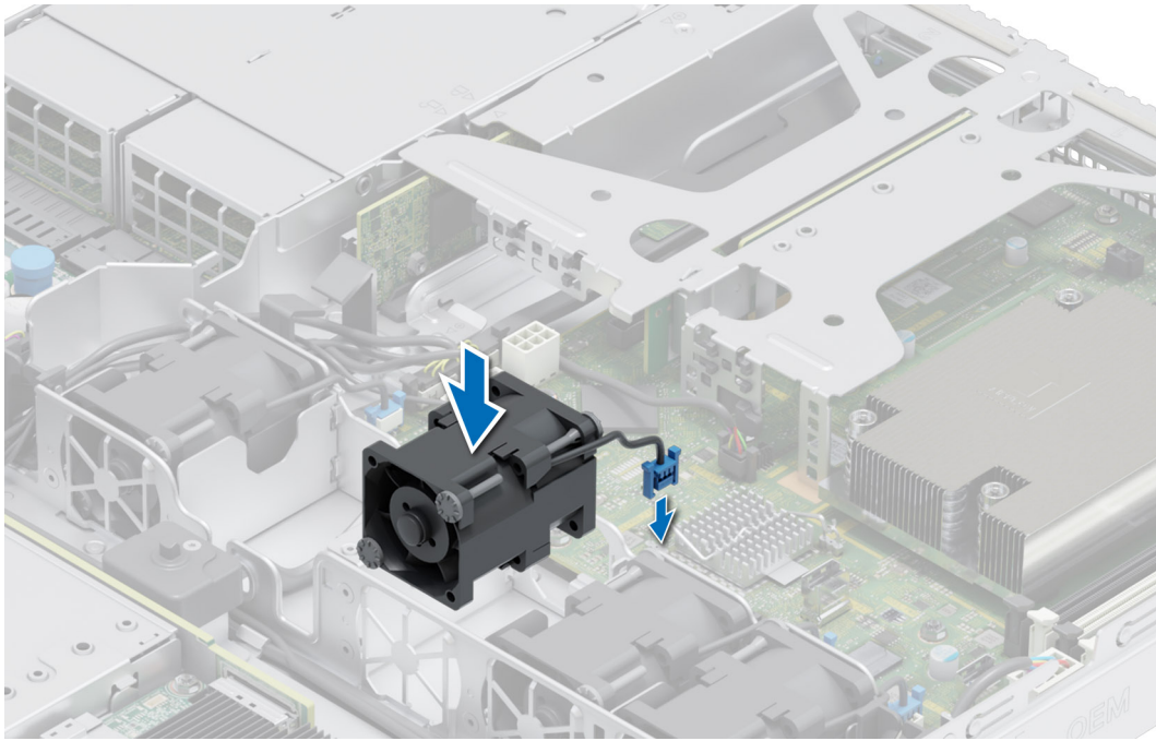
Figure 16. Installation d'un ventilateur
