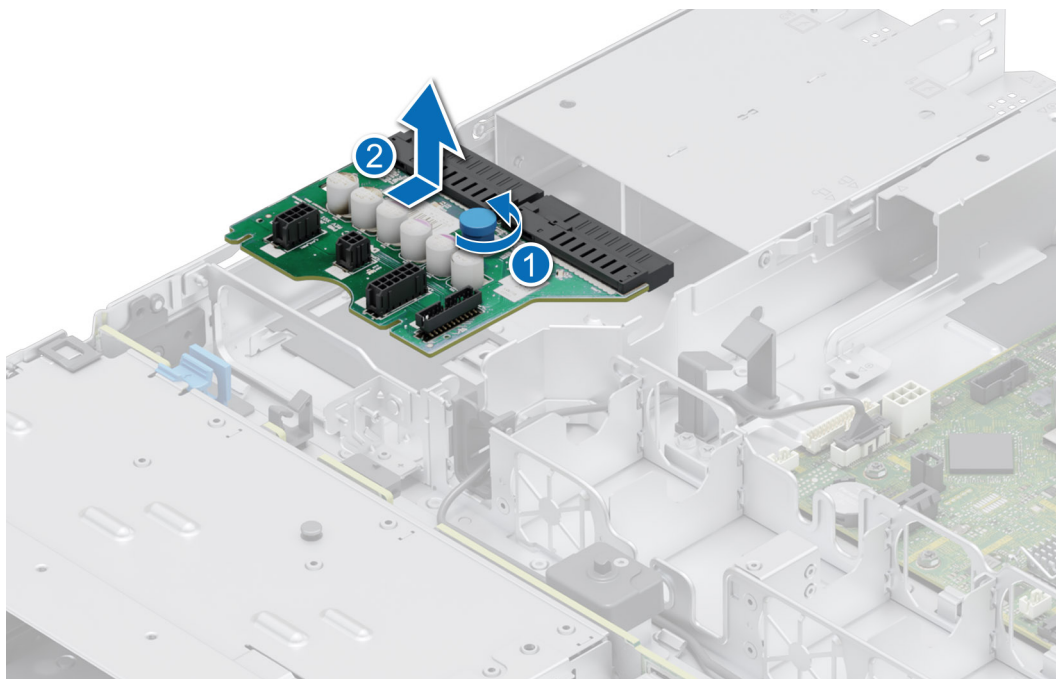
Figure 71. Retrait de la carte intercalaire d'alimentation
