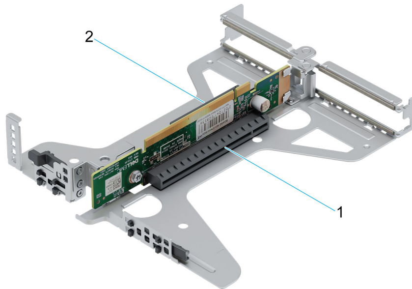
Figure 46. Carte de montage papillon
