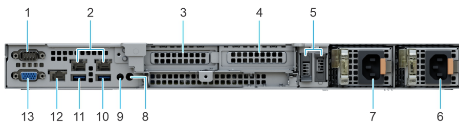
Figure 3. Vue arrière du système
