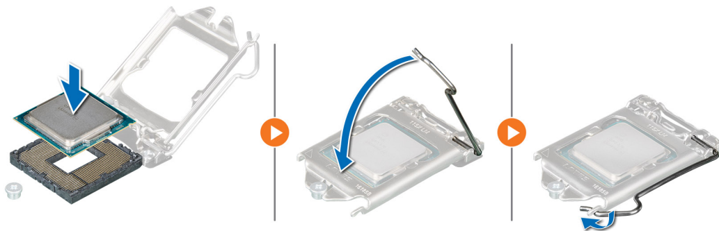
Figure 44. Installation du processeur
