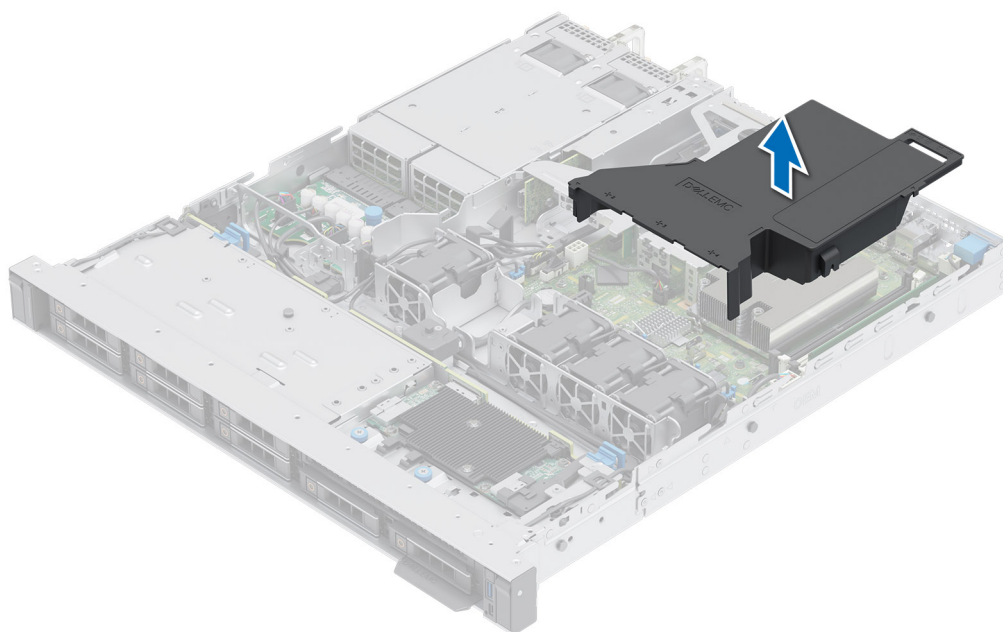
Figure 13. Retrait du carénage d'aération
