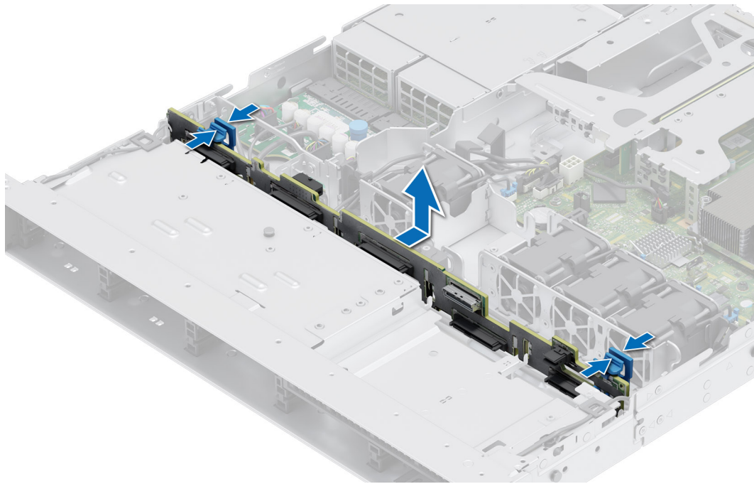
Figure 21. Retrait du fond de panier
