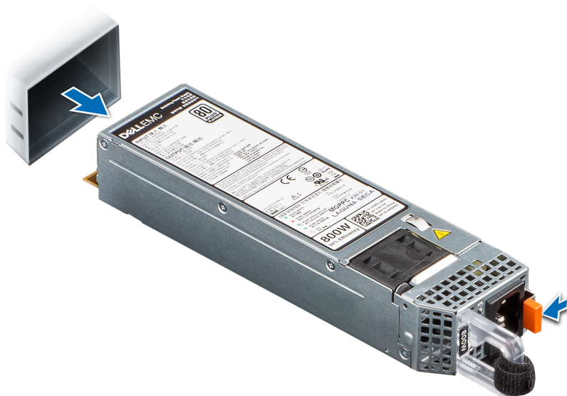
Figure 67. Retrait d'un bloc d'alimentation
