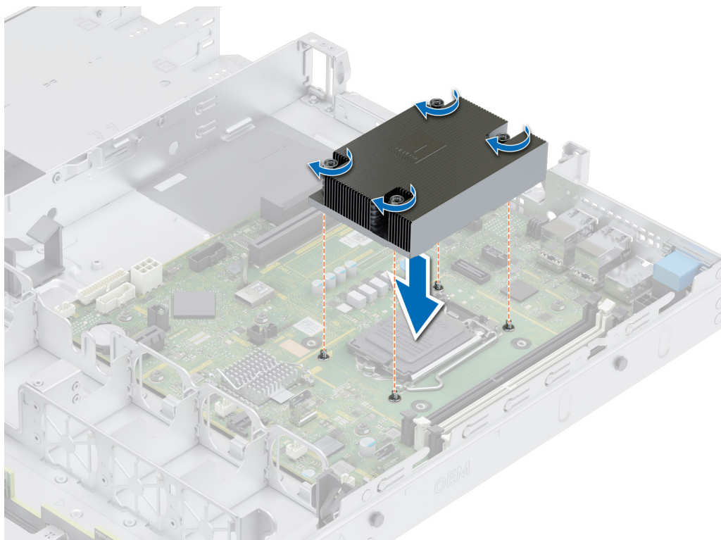
Figure 42. Installation du dissipateur de chaleur
