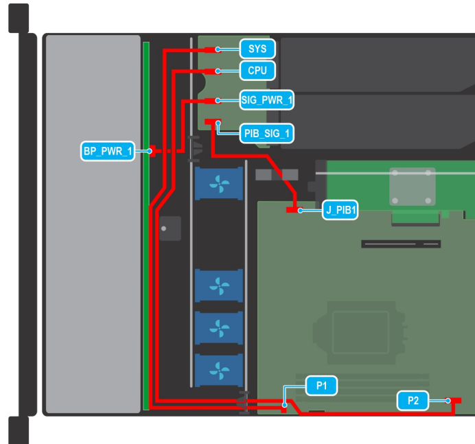
Figure 27. Acheminement des câbles : fond de panier pour 8 disques SAS ou SATA de 2,5 pouces avec PIB
