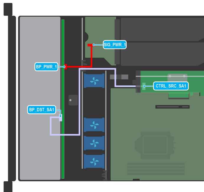
Figure 26. Acheminement des câbles : fond de panier pour 8 disques SATA de 2,5 pouces avec carte PERC interne
