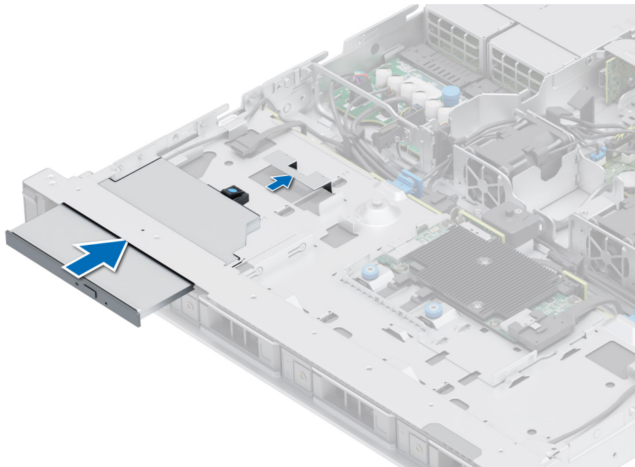
Figure 36. Installation du lecteur optique
