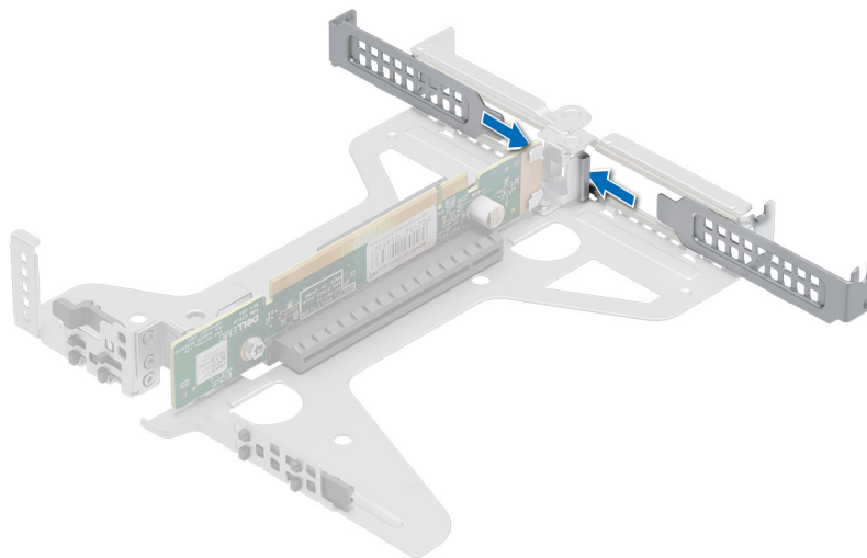
Figure 50. Installation de la plaque de recouvrement dans la carte de montage
