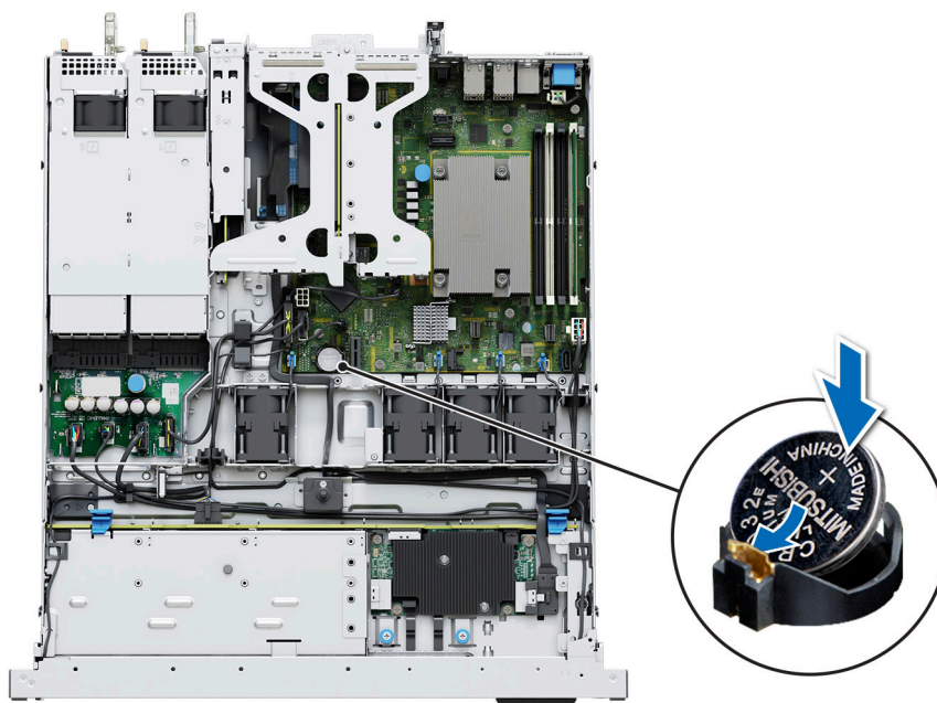
Figure 60. Installation de la pile du système
