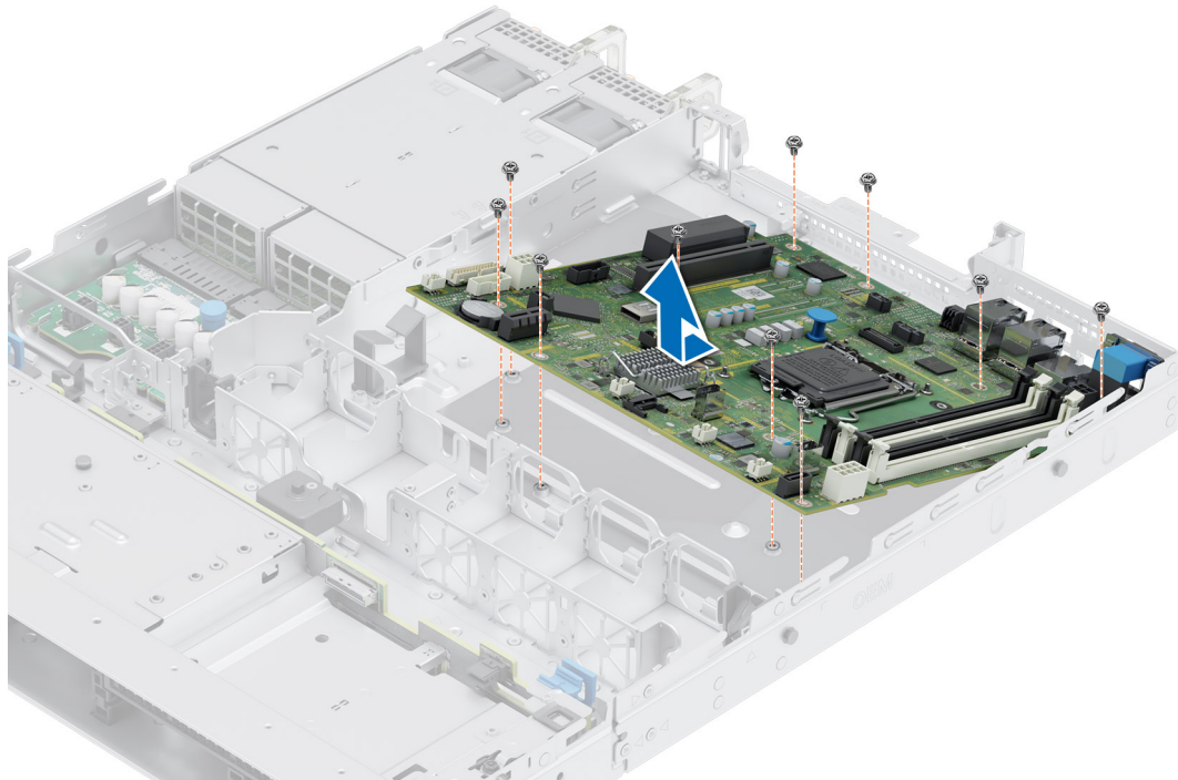
Figure 77. Retrait de la carte système
