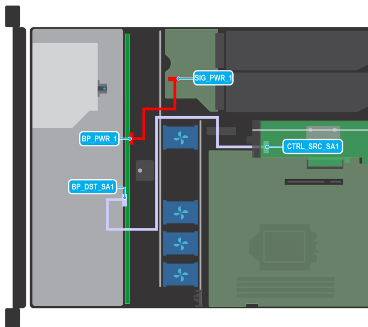
Figure 23. Acheminement des câbles : fond de panier pour 4 disques SAS ou SATA de 3,5 pouces
