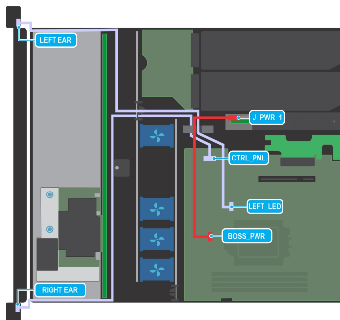
Figure 28. Acheminement des câbles : fond de panier pour 8 disques SAS ou SATA de 2,5 pouces avec panneau de configuration
