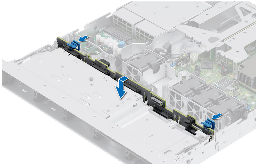
Figure 22. Installation du fond de panier de disque
