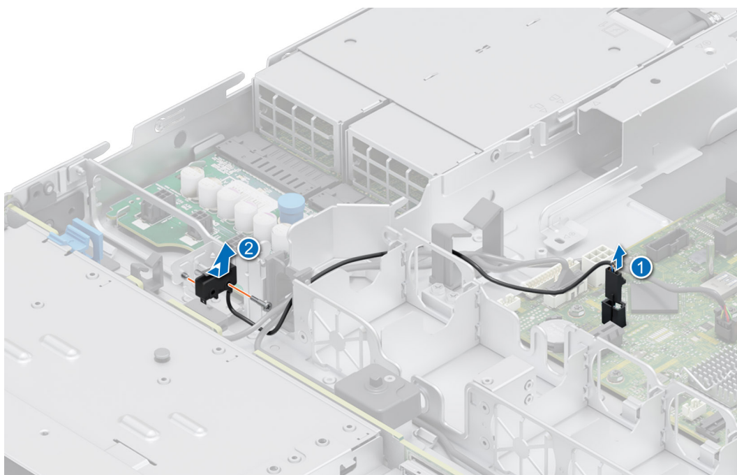
Figure 17. Retrait du module du commutateur d'intrusion
