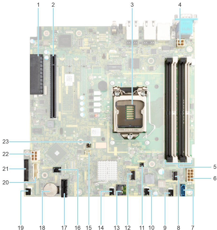
Figure 84. Connecteurs et cavaliers de la carte système
