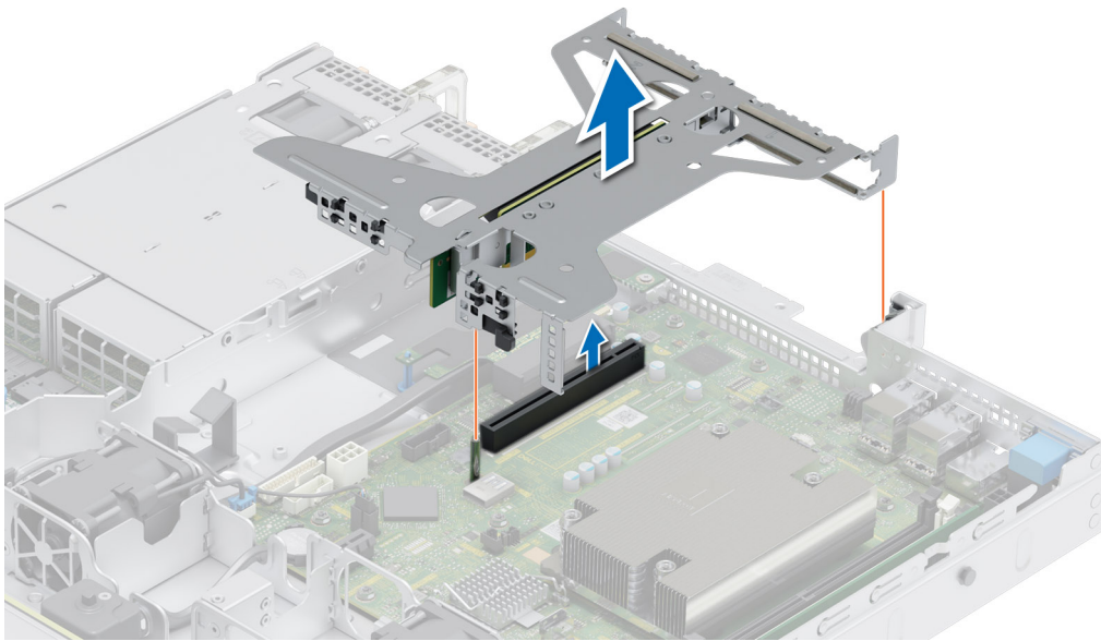
Figure 47. Retrait de la carte de montage papillon
