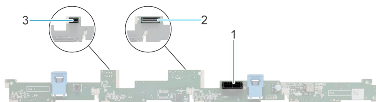
Figure 20. Fond de panier de 8 disques de 2,5 pouces
