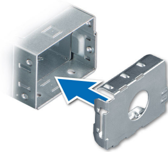
Figure 70. Installation du cache de bloc d'alimentation
