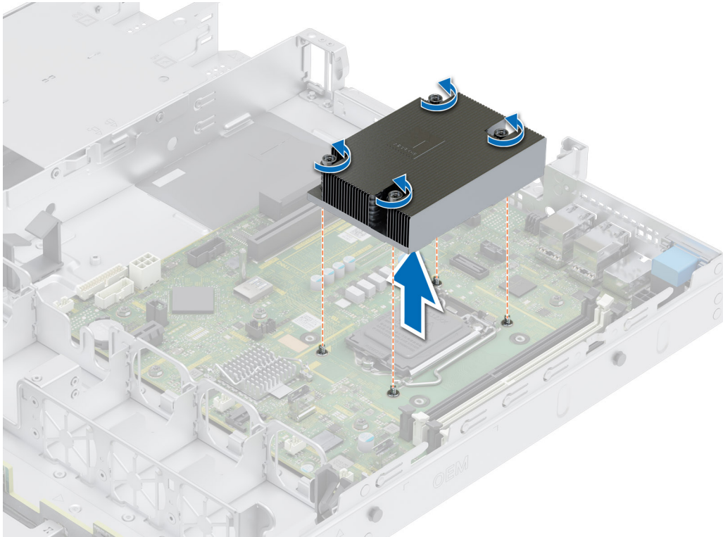
Figure 40. Retrait du dissipateur de chaleur
