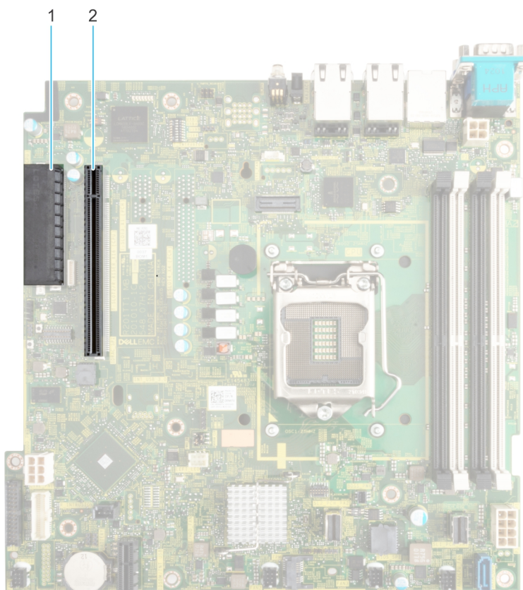
Figure 45. Connecteurs des logements de carte d'extension
