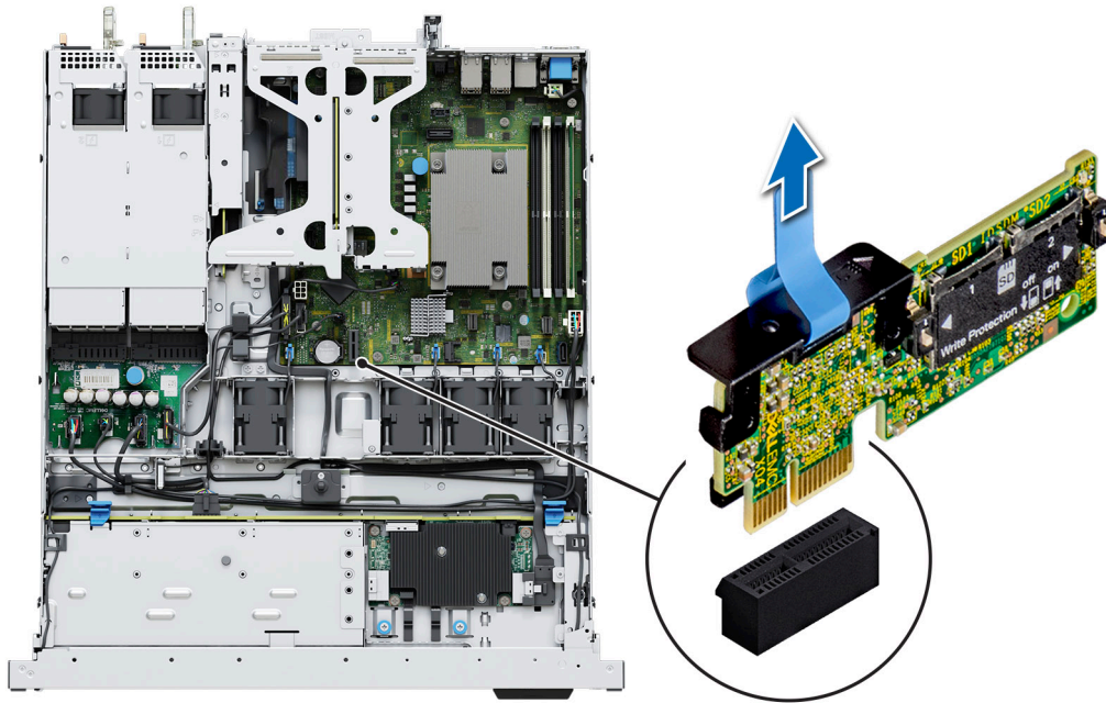
Figure 73. Retrait du module IDSDM
