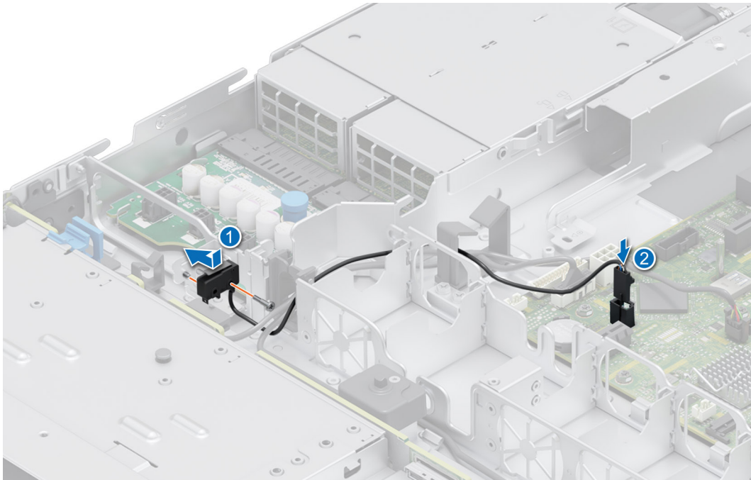
Figure 18. Installation du commutateur d'intrusion
