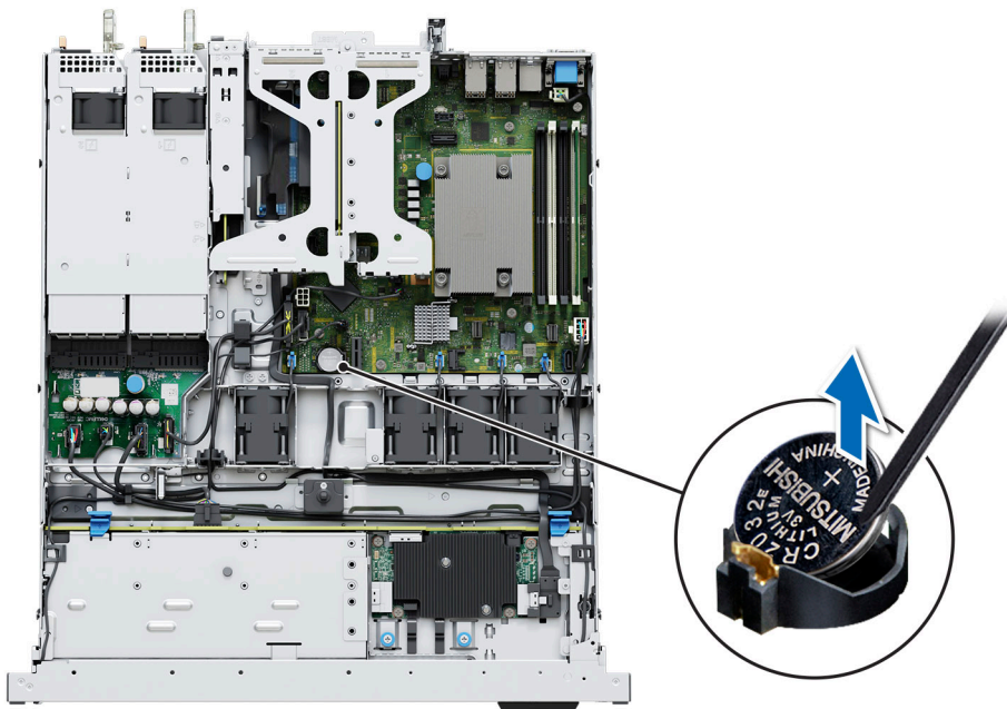
Figure 59. Retrait de la pile du système
