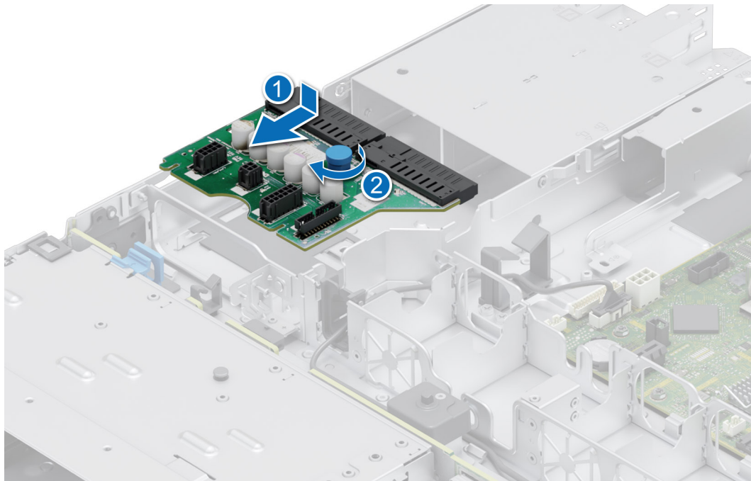
Figure 72. Installation de la carte intercalaire d'alimentation
