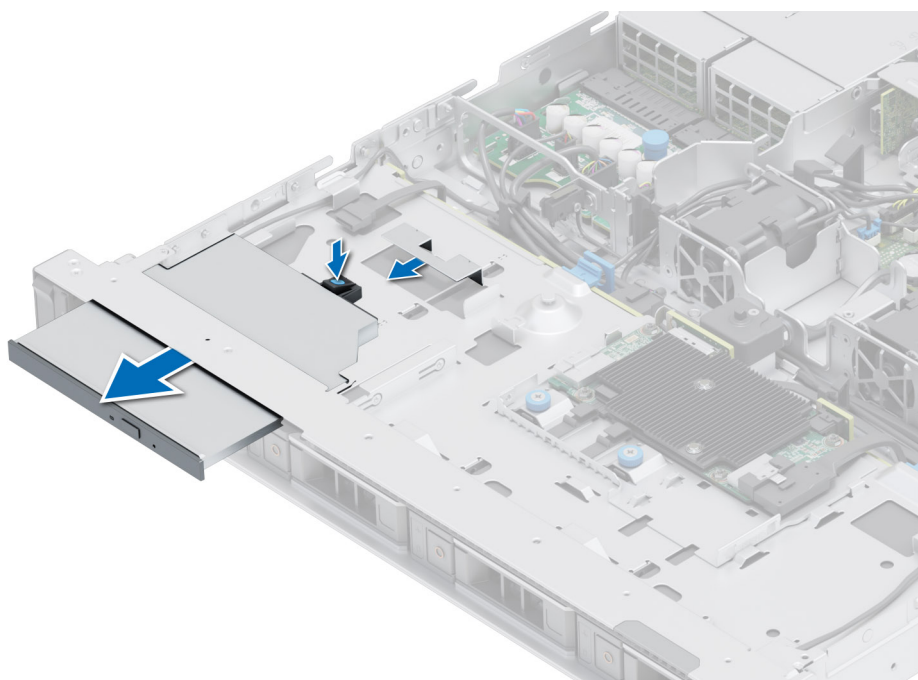
Figure 35. Retrait du lecteur optique
