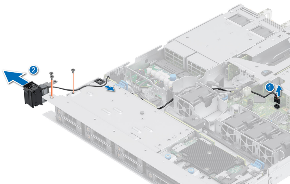
Figure 80. Retrait du panneau de configuration gauche
