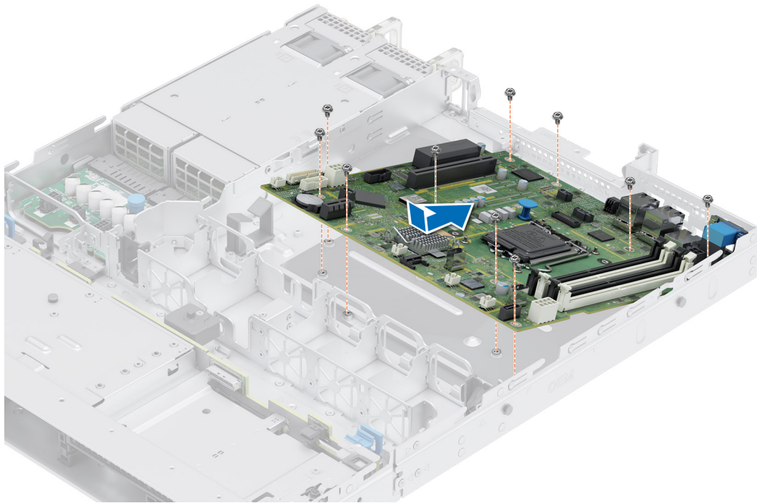
Figure 78. Installation de la carte système
