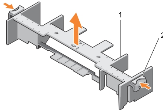
Ilustración 11. Extracción de la cubierta de refrigeración
