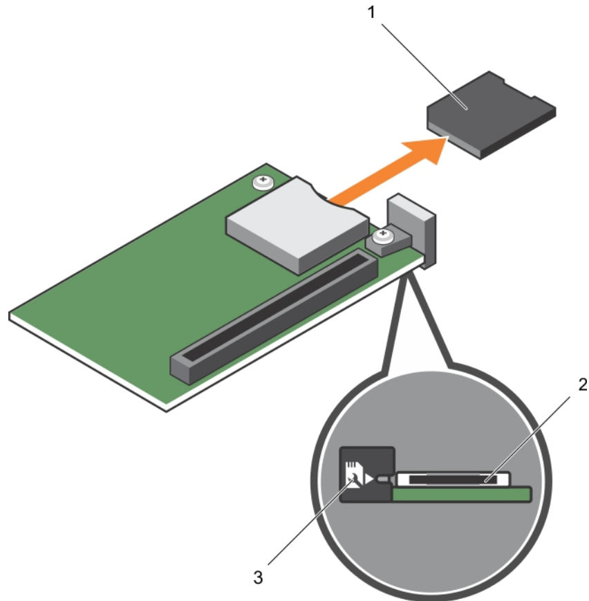
Ilustración 27. Sustitución de la tarjeta vFlash SD
