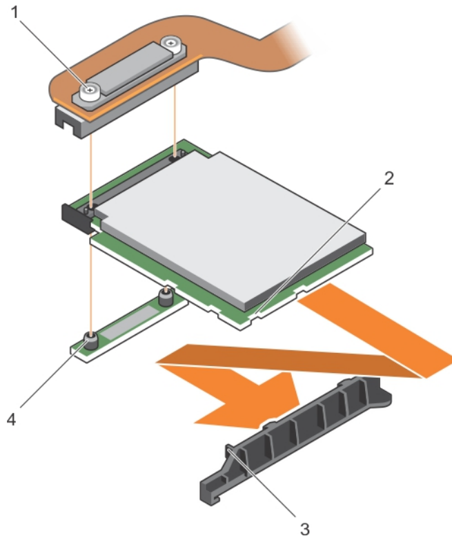
Ilustración 57. Instalación de la tarjeta extendida PCIe o de la controladora de almacenamiento
