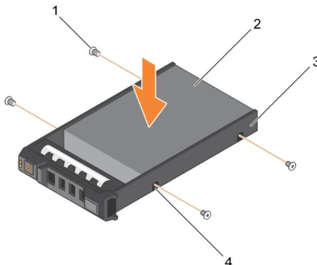
Ilustración 47. Instalación de una unidad de disco duro o SSD de 2,5 pulgadas en un portaunderidades de disco duro o SSD de 2,5 pulgadas
