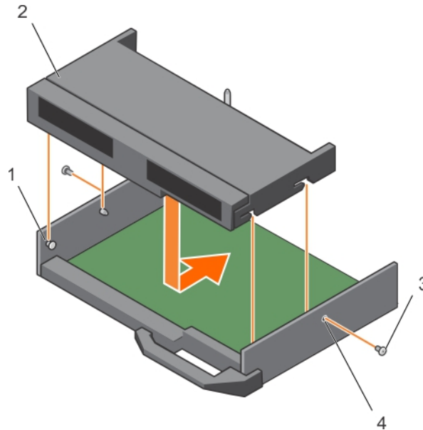
Ilustración 51. Instalación del compartimento de la unidad de disco duro o SSD
