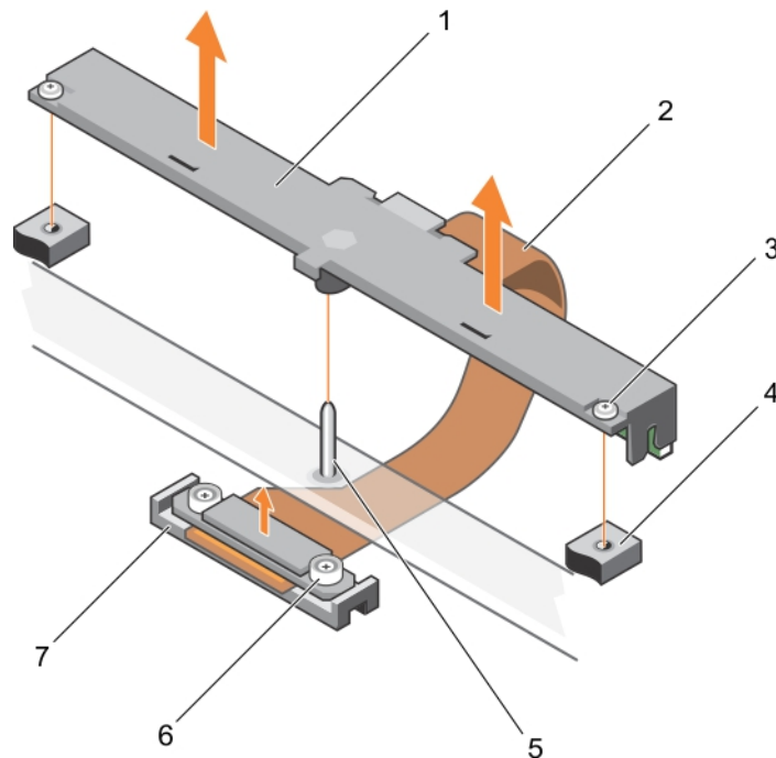
Ilustración 52. Extracción del plano posterior de la SSD o de la unidad de disco duro
