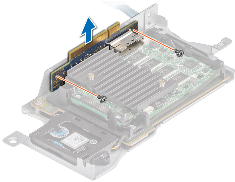
그림 77 . NVMe 브리지 커넥터 보드 제거
