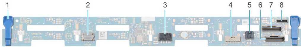
그림 92 . 2.5" 드라이브 NVME 백플레인
