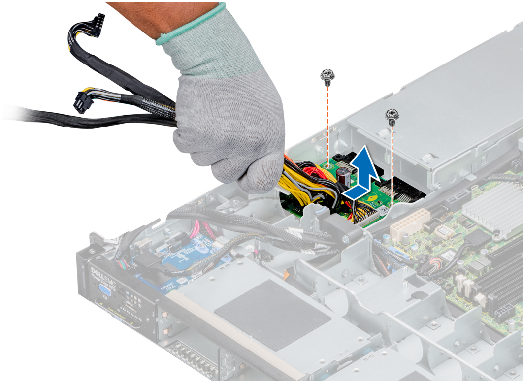
그림 103 . PIB 제거
