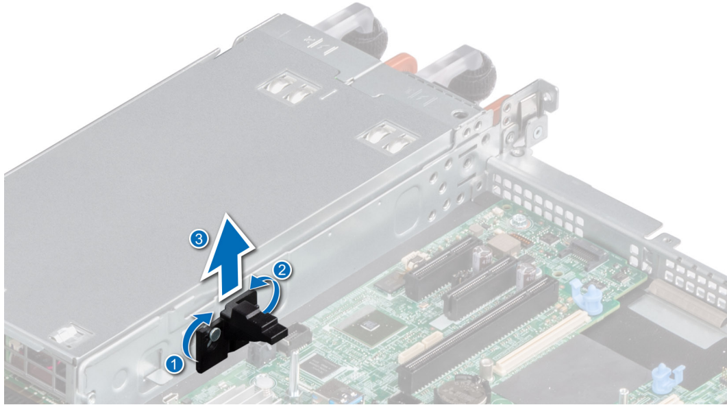
그림 109 . 라이저 2 지지 클립 제거
