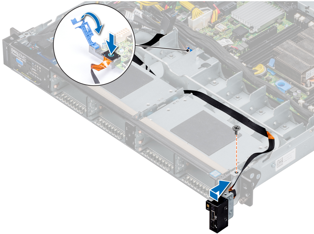
그림 108 . 오른쪽 제어판 설치
