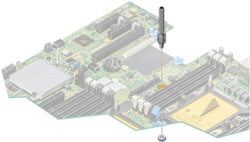
그림 115 . 시스템 보드에 901D 격리 애자 육각 스페이서 설치
