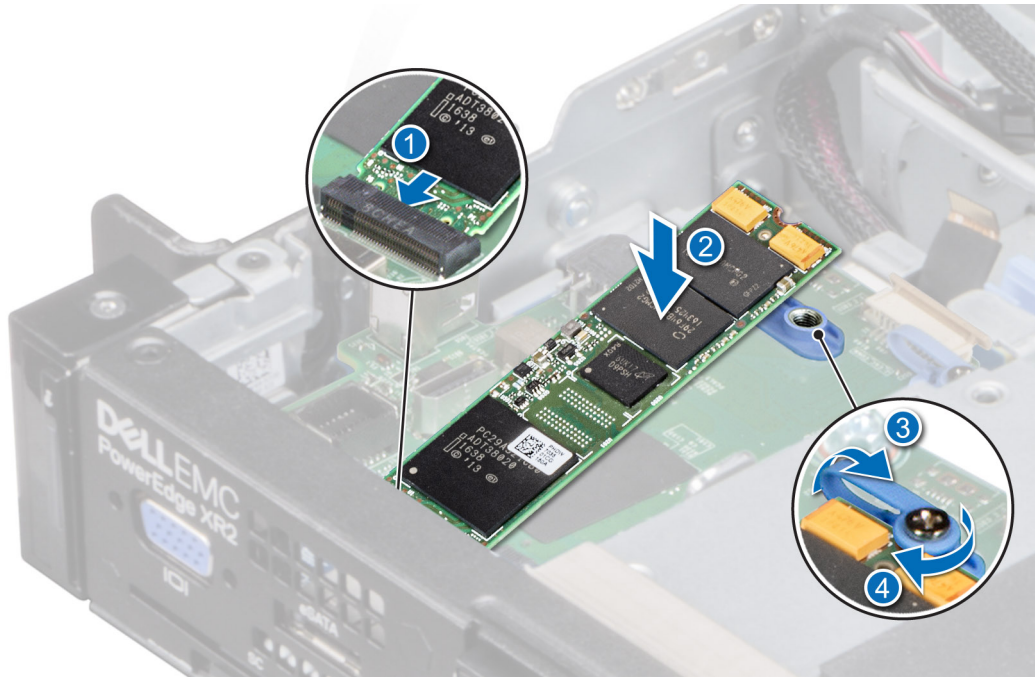
그림 36 . 내부 M.2 SSD 모듈 설치
