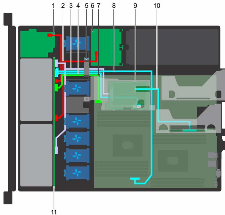
그림 97 . 케이블 라우팅 - NVMe miniPERC 라이저 및 2개의 프로세서가 장착된 8개의 2.5" NVMe 백플레인 포함
