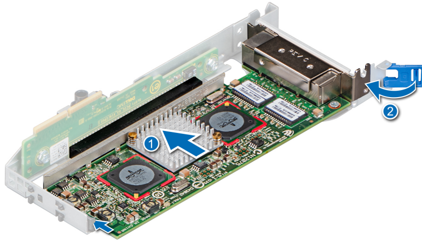
그림 118 . 901D 라이저에 PCI 카드 설치
