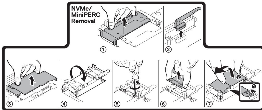
그림 16 . NVME/MiniPERC 제거
