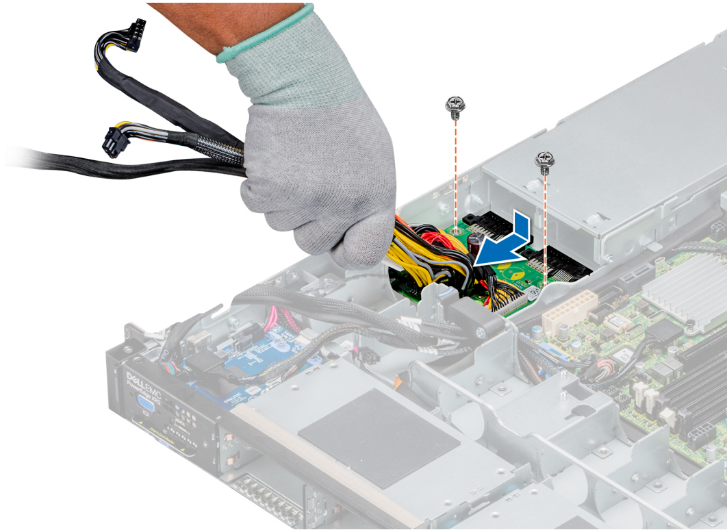
그림 104 . PIB 설치
