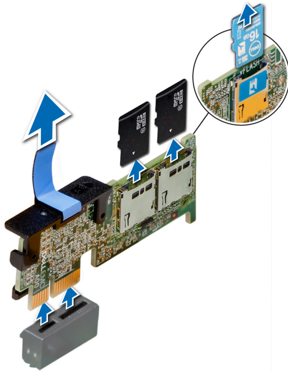
그림 87 . IDSDM/vFlash 카드(선택 사항) 제거
