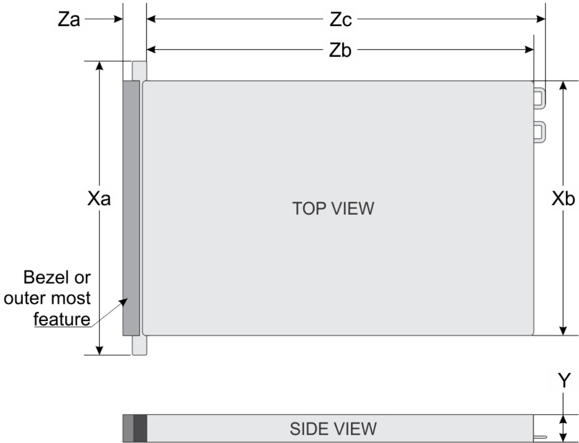
그림 17 . PowerEdge XR2 시스템의 크기
