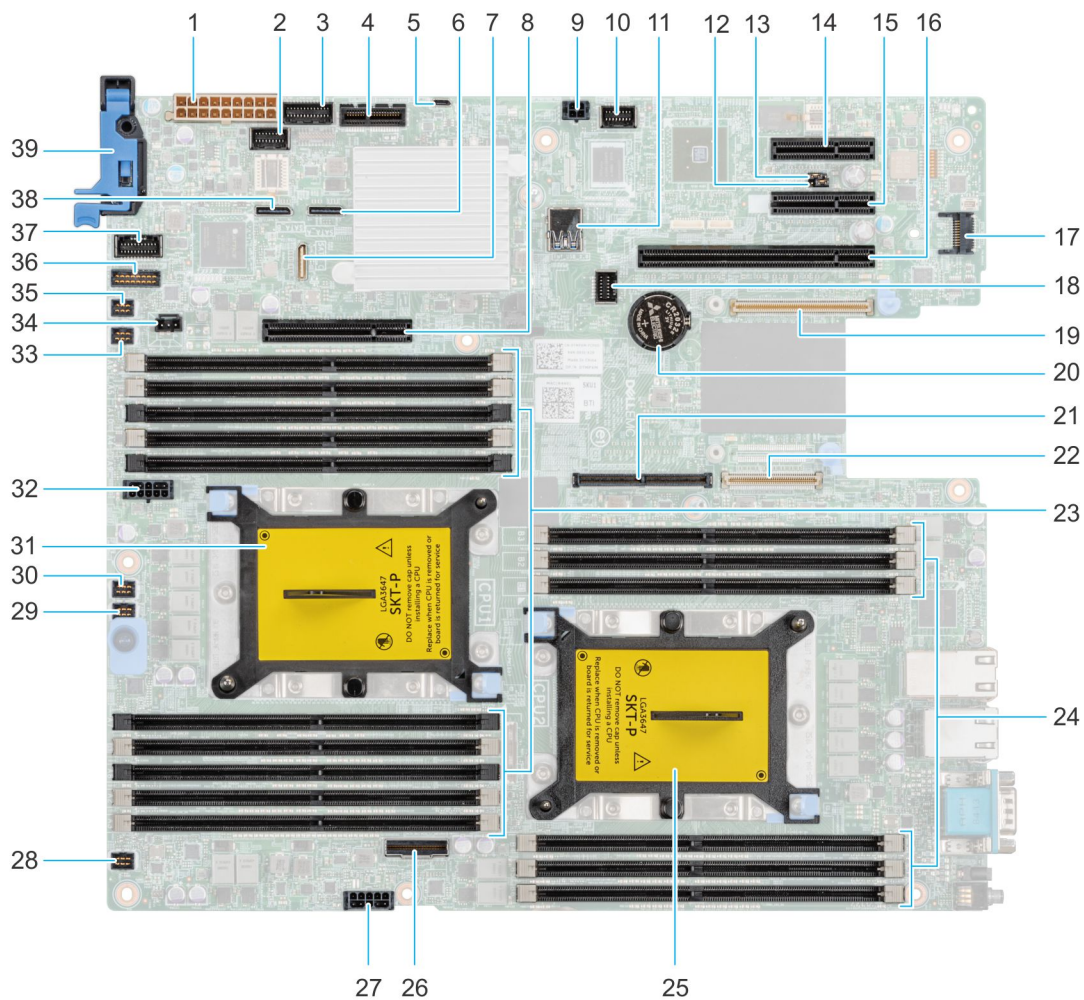
그림 126 . 시스템 보드 점퍼 및 커넥터
