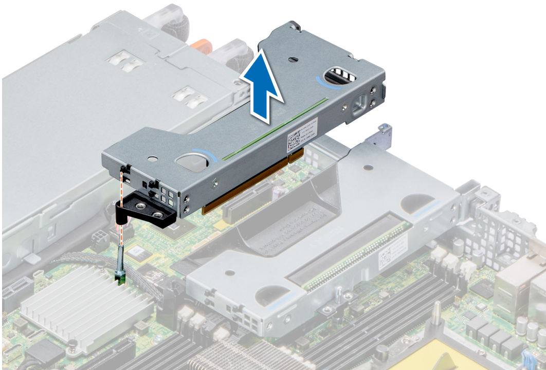
그림 64 . 로우 프로파일 라이저(라이저 2) 제거
