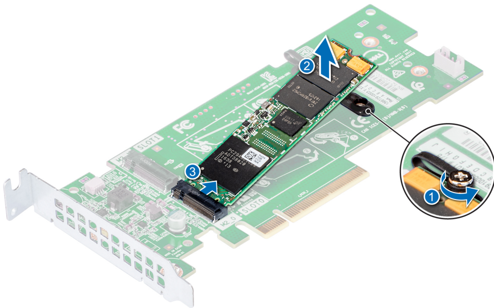
그림 85 . M.2 SSD 모듈 분리
