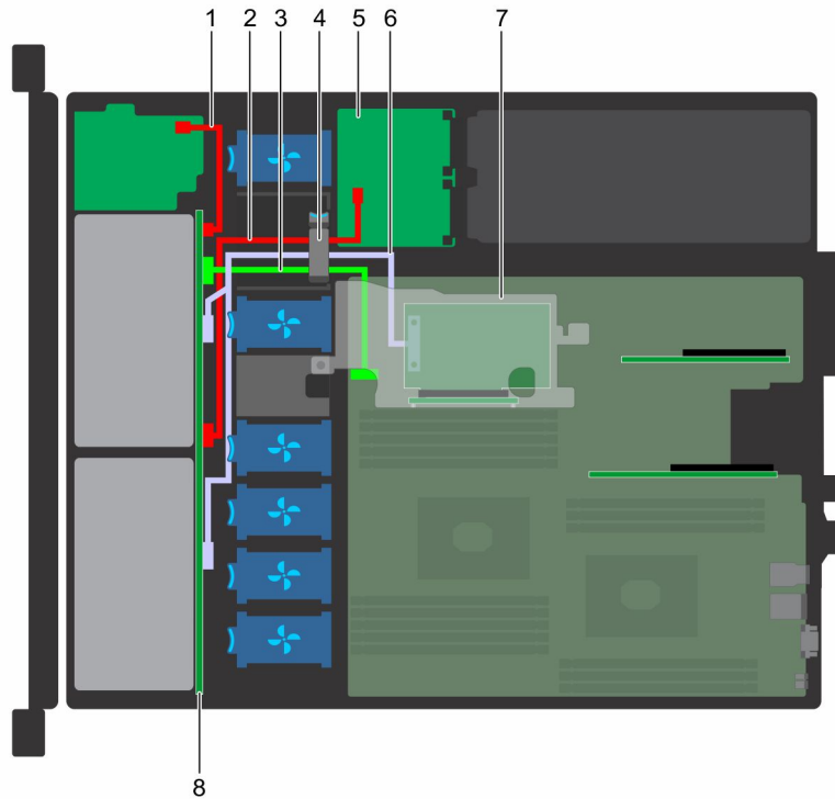
그림 95 . 케이블 라우팅 - miniPERC를 포함하는 8개의 2.5" 하드 드라이브 백플레인
