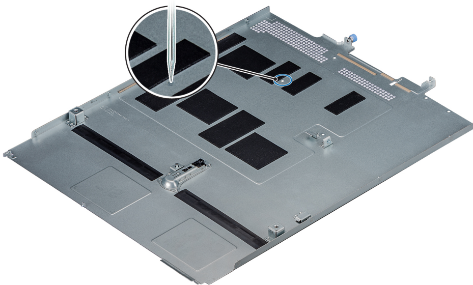
그림 121 . 격리 애자 육각 스페이스 나사 구멍 노출
