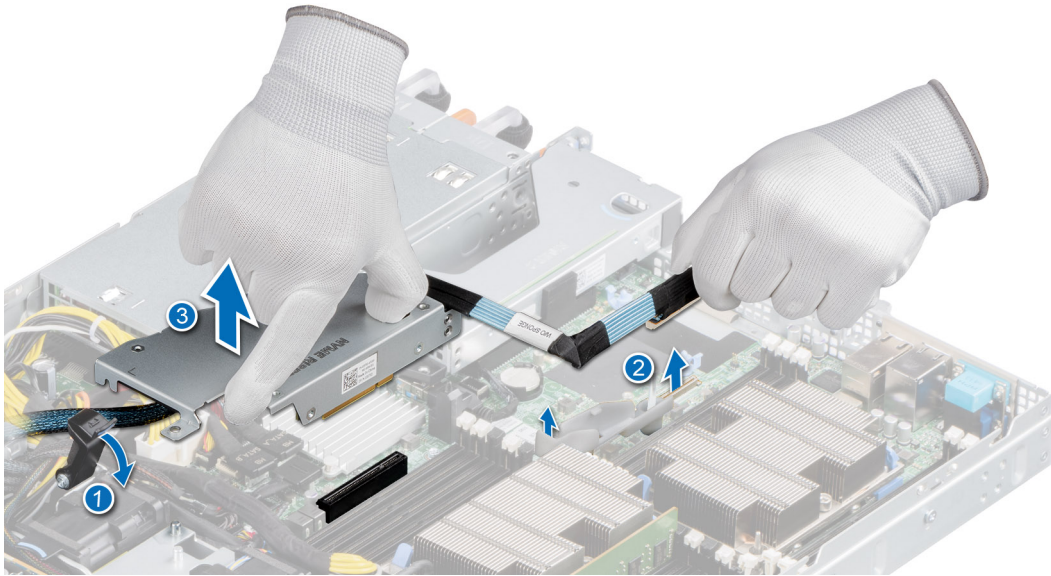
그림 75 . NVMe PERC 라이저 제거
