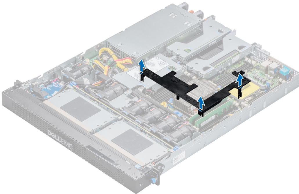
그림 29 . 공기 덮개 분리
