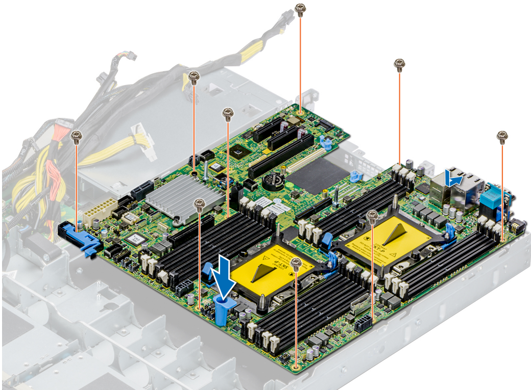
그림 112. 시스템 보드 설치
