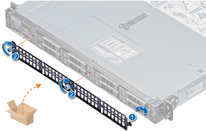
그림 124 . 드라이브 잠금 장치 설치
