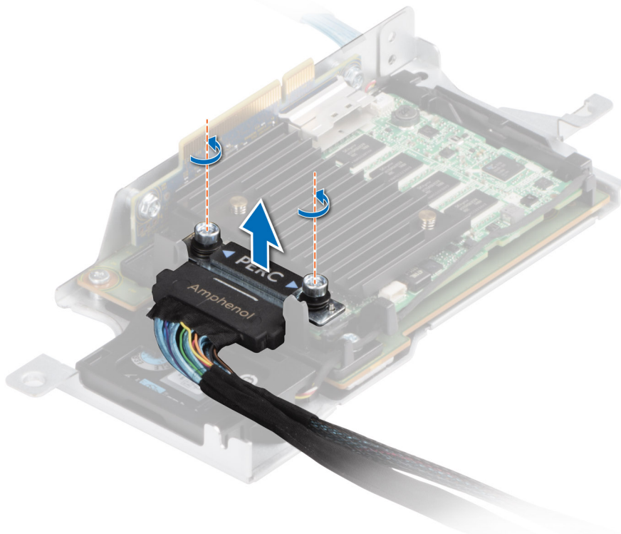
그림 78 . 라이저에서 miniPERC 케이블 제거
