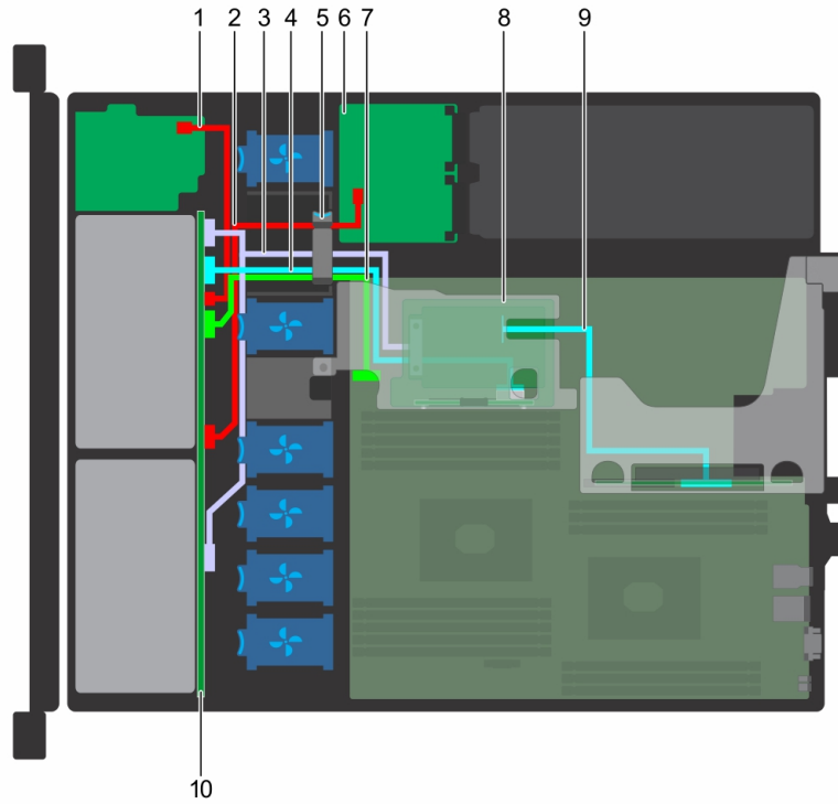
그림 98 . 케이블 라우팅 - NVMe MiniPERC 라이저 및 1개의 프로세서가 장착된 8개의 2.5" 하드 드라이브 NVMe 백플레인 포함
