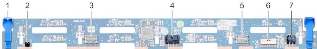
그림 91 . 8개의 2.5" 드라이브 백플레인
