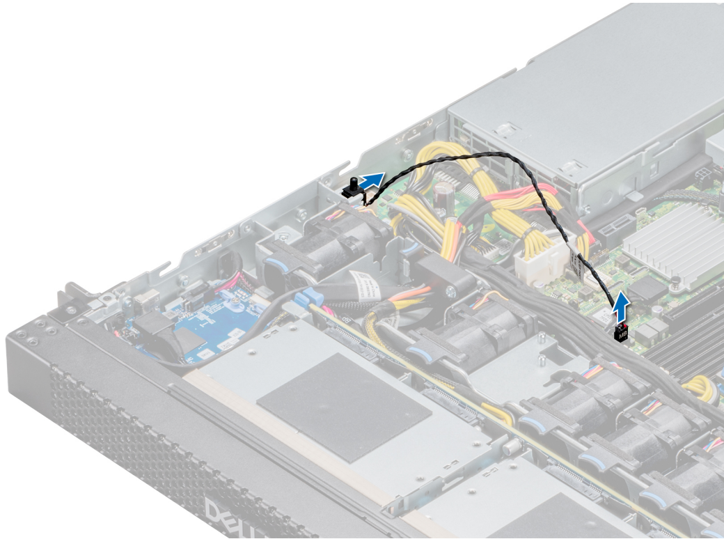
그림 41. 침입 스위치 제거
