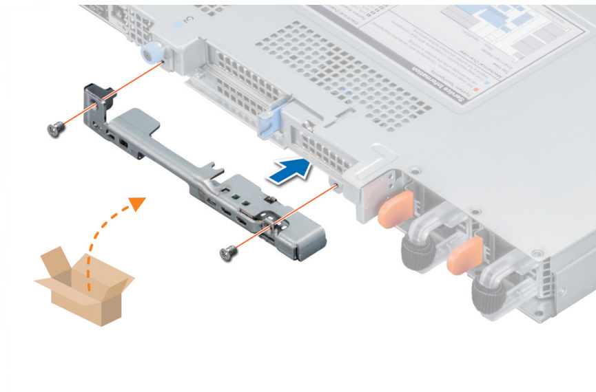
그림 125 . 901D PCI 견고한 브래킷 설치
