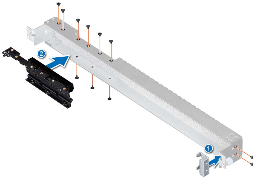
그림 24. LCD 베젤(옵션) 설치
