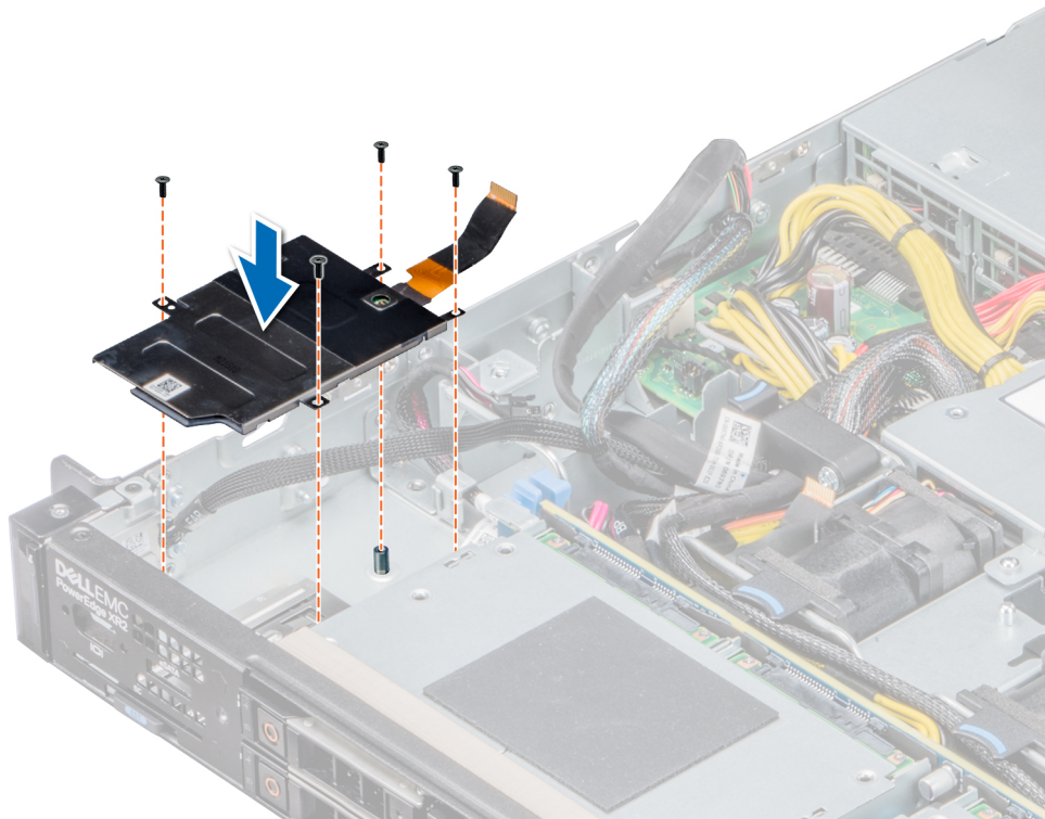
그림 39. 스마트 카드 판독기 장착
