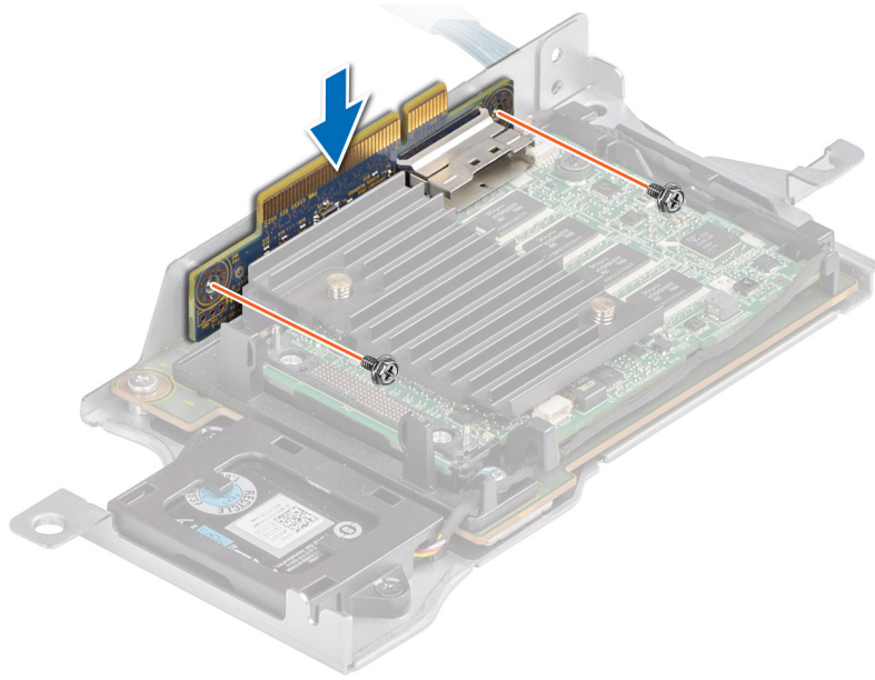
그림 83 . NVMe 브리지 커넥터 보드 설치
