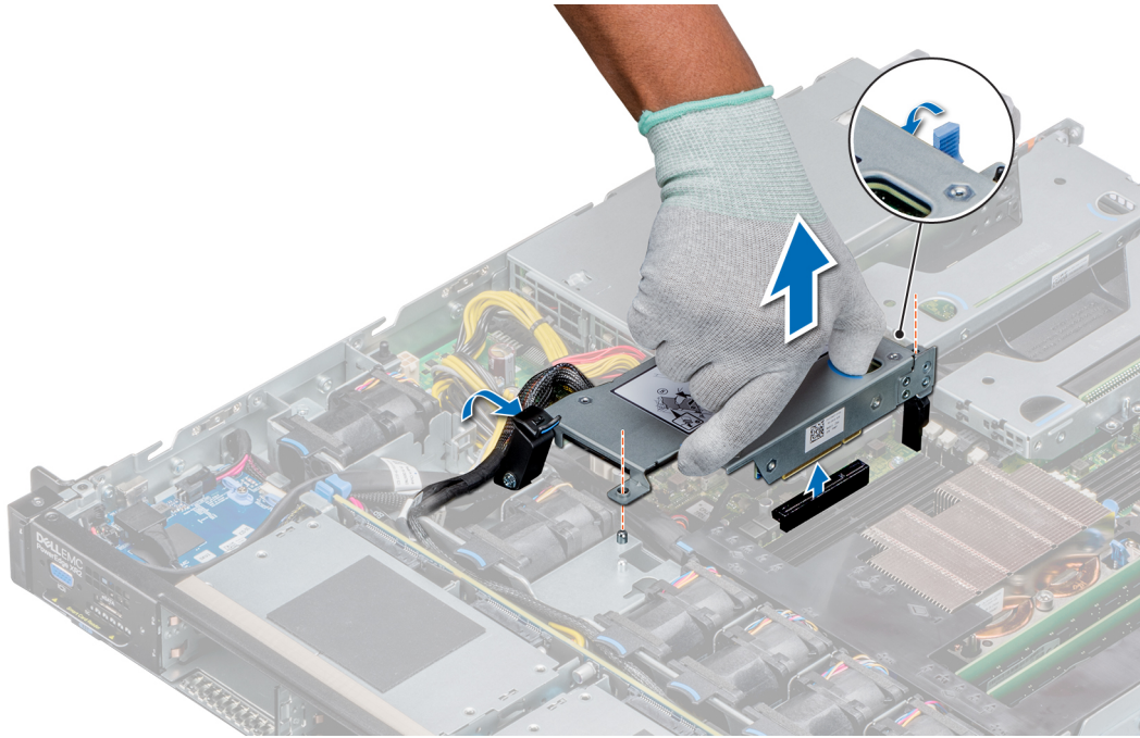
그림 59 . 내부 MiniPERC 라이저 제거
