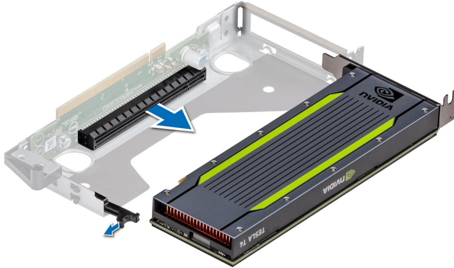
그림 71. 로우 프로파일 라이저에서 GPU 카드 제거
