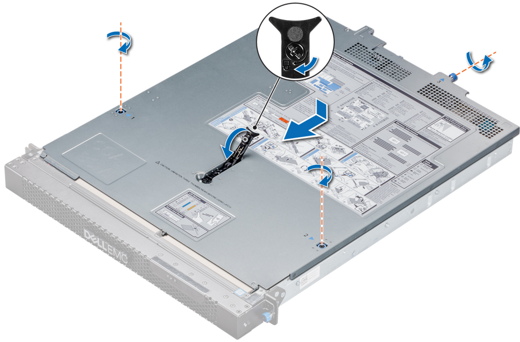
그림 27. 시스템 덮개 장착
