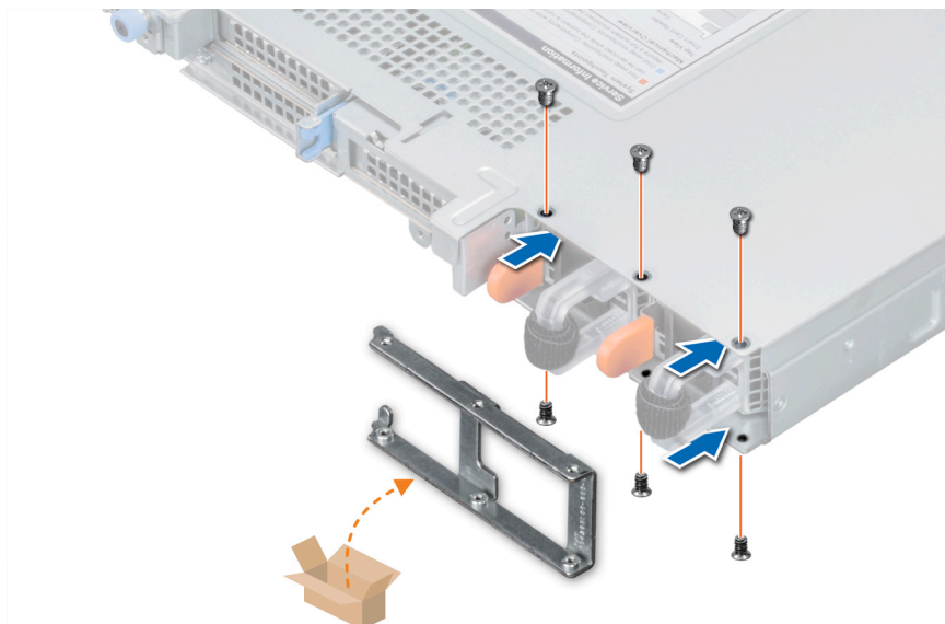
그림 123 . 901D 전원 공급 장치 견고한 브래킷 설치
