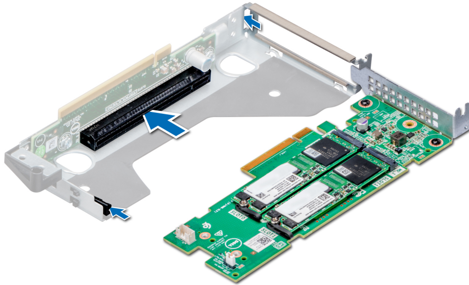
그림 70. 로우 프로파일 라이저에 확장 카드 설치
