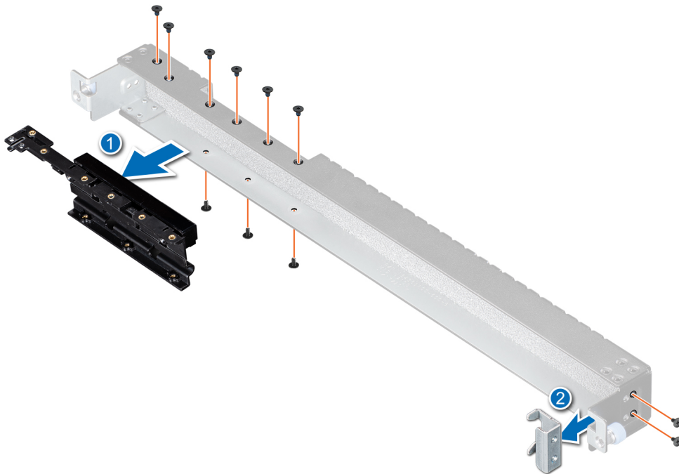
그림 21. LCD 베젤(옵션) 제거
