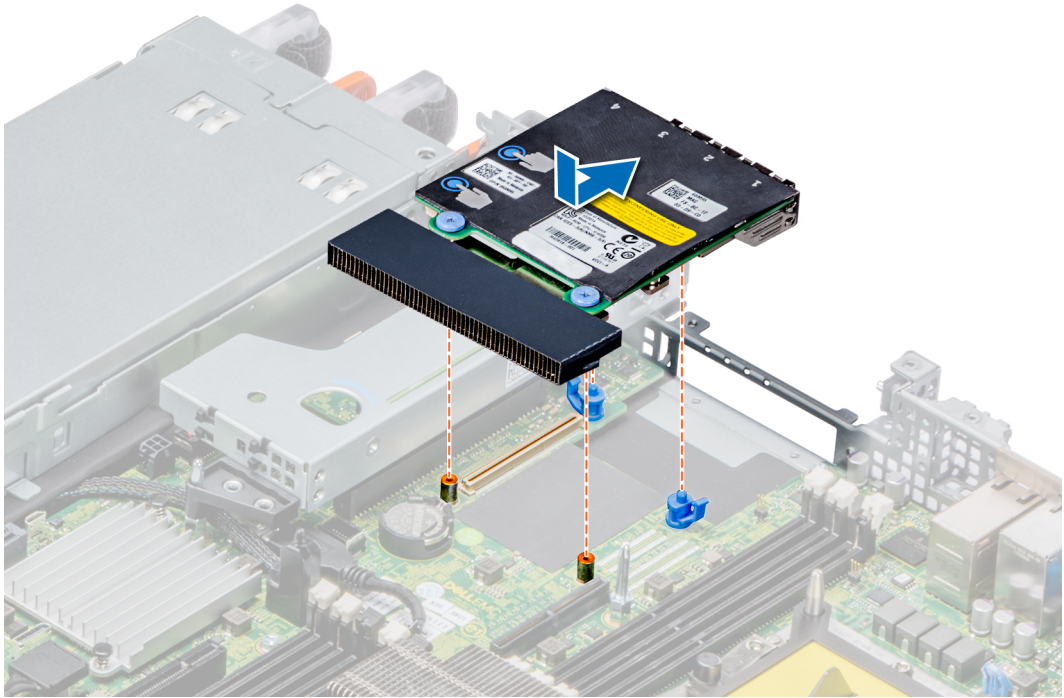
그림 90 . LOM 라이저 카드 설치
