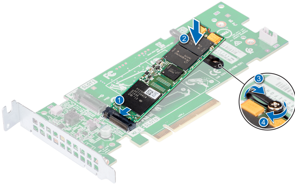
그림 86 . M.2 SSD 모듈 설치
