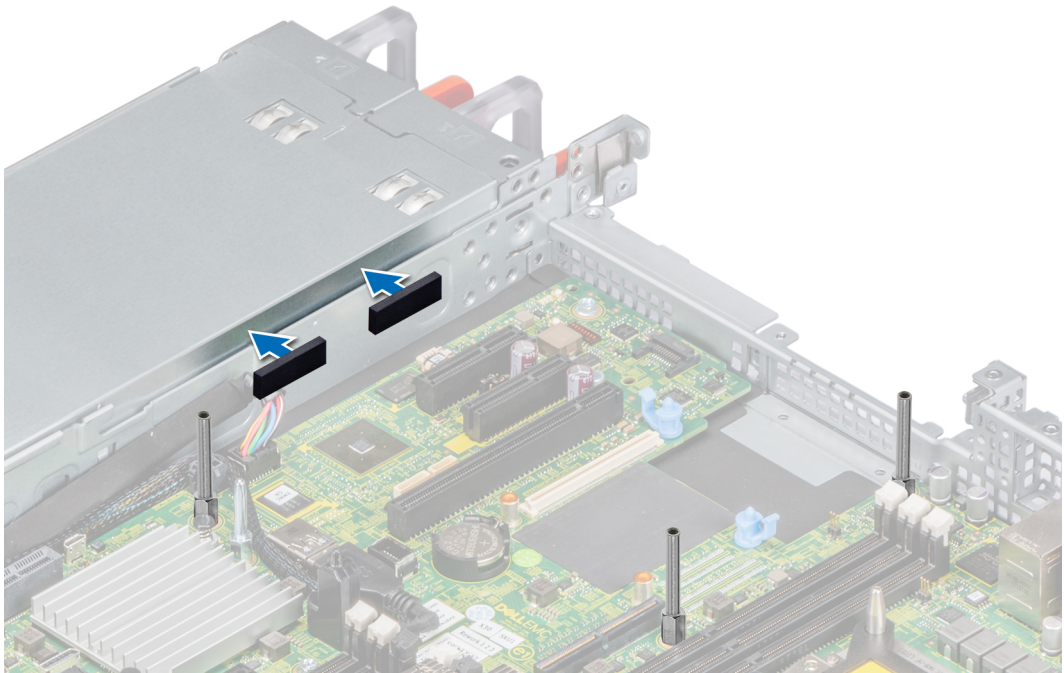
그림 117 . 마일라 폼 설치
