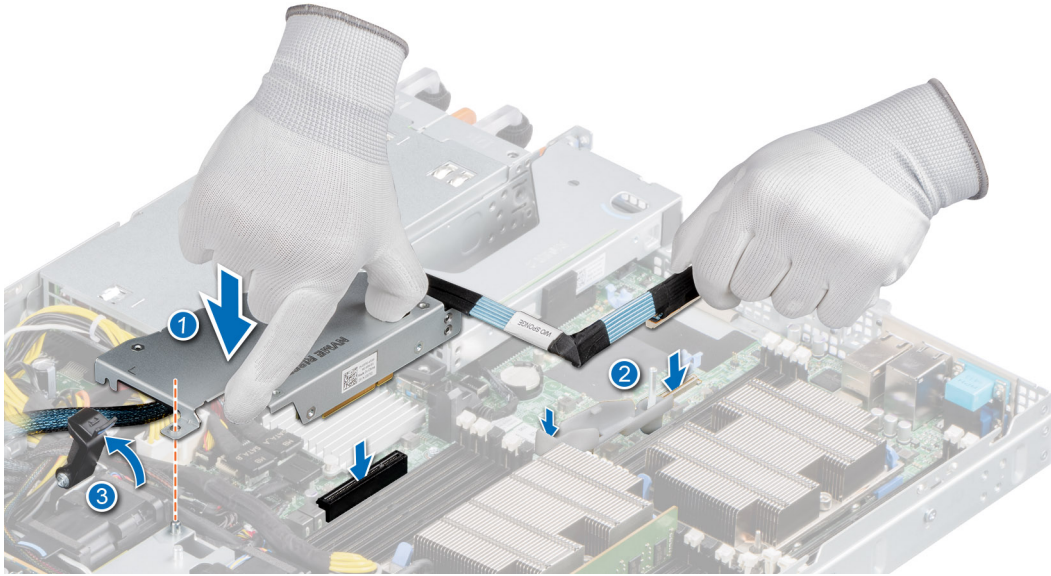
그림 76 . NVMe PERC 라이저 설치
