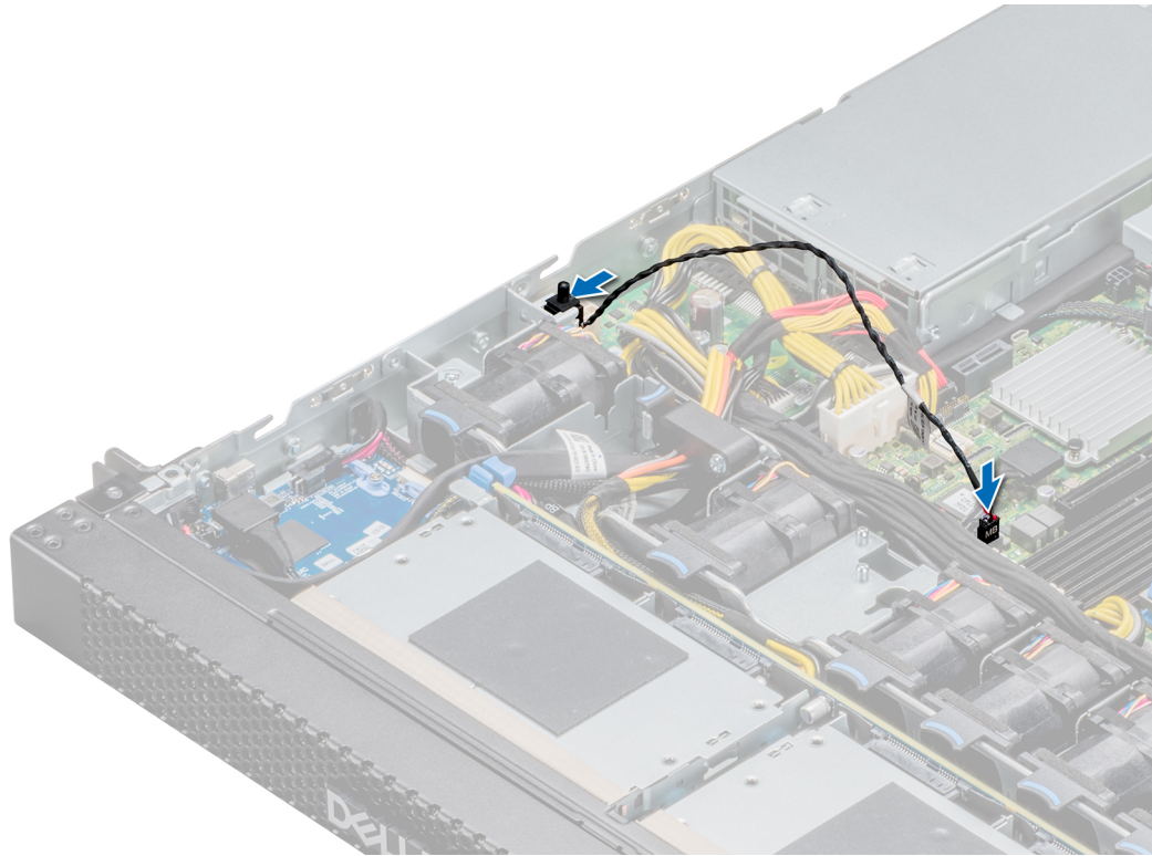
그림 42. 침입 스위치 설치
