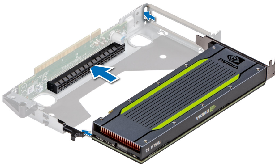
그림 74. 로우 프로파일 라이저에 GPU 카드 설치
