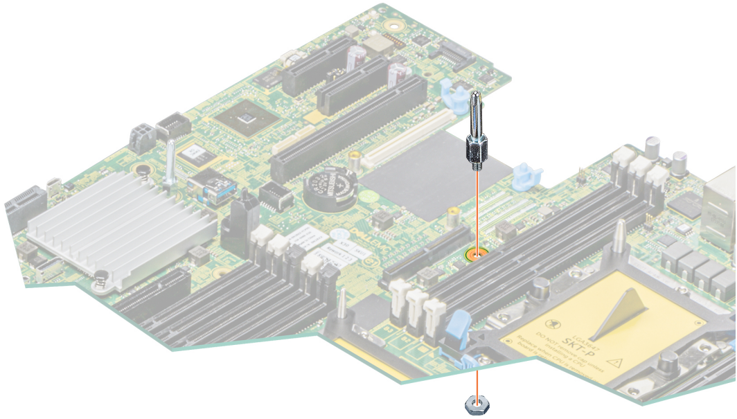
그림 114 . 시스템 보드에서의 격리 애자 육각 스페이서 제거
