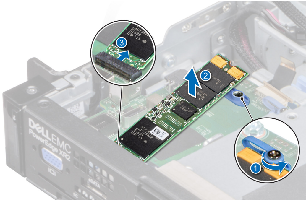
그림 35 . 내부 M.2 SSD 모듈 제거
