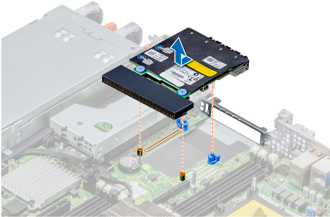
그림 89 . LOM 라이저 카드 분리
