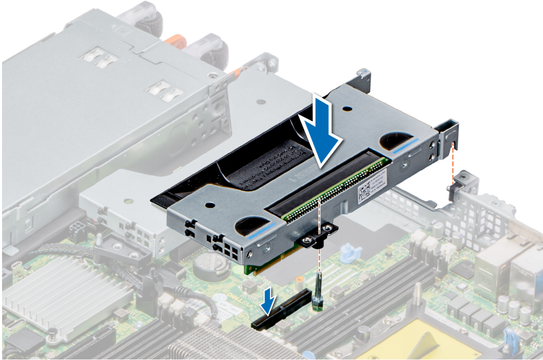
그림 65. 로우 프로파일 라이저 오른쪽(라이저 1) 설치
