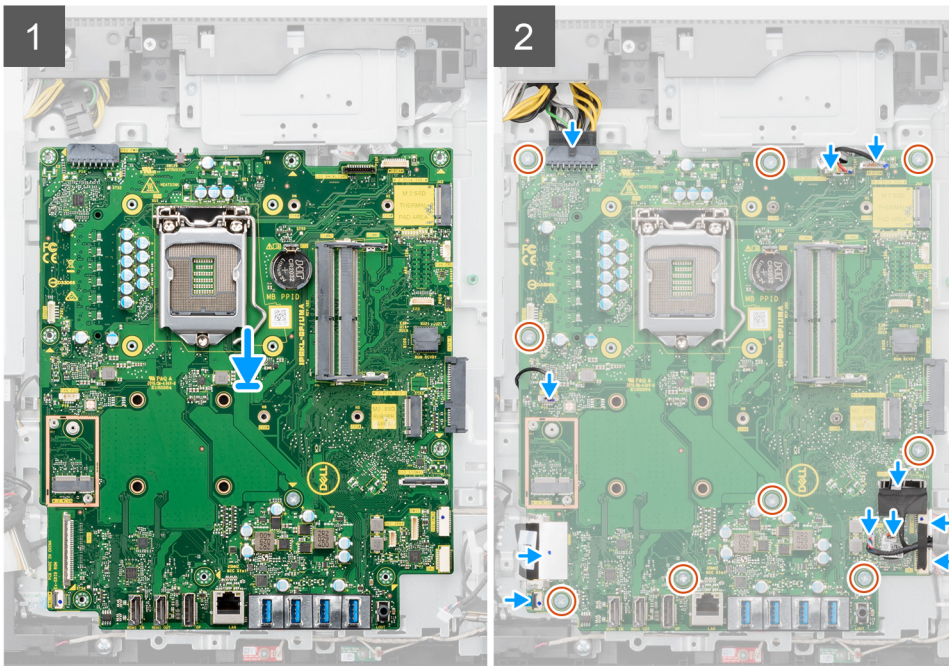
9x M3x5
