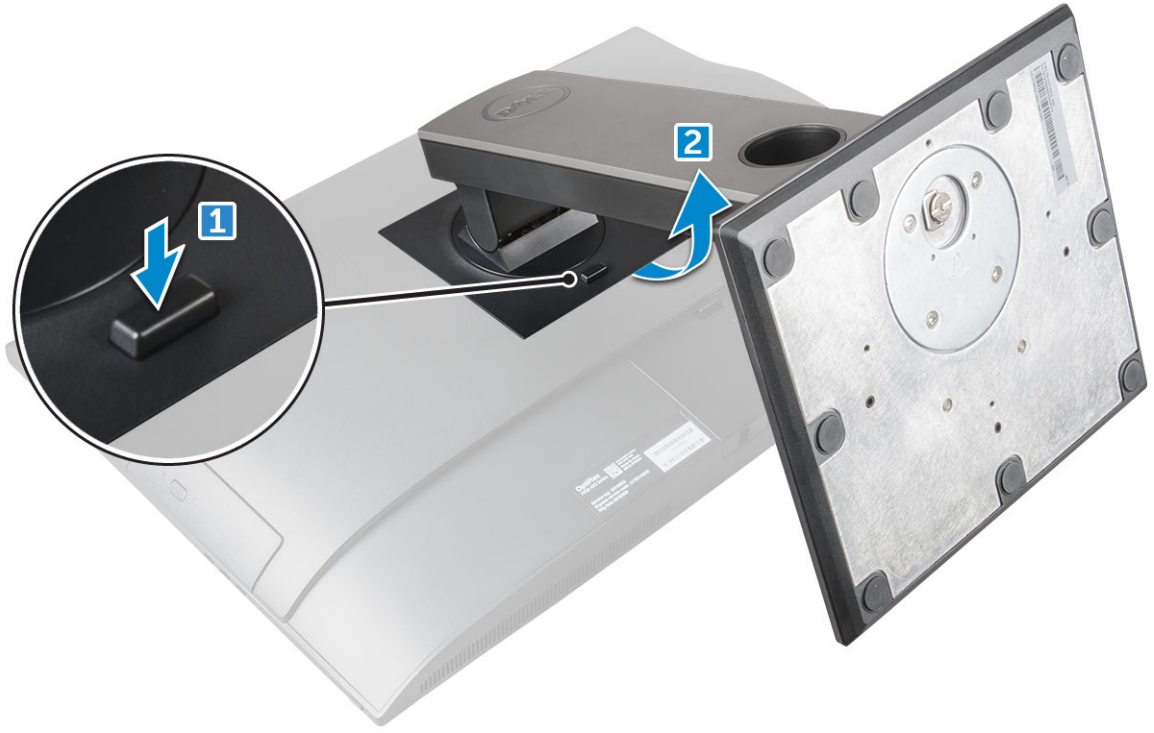
Rakam 1. Yüksekliđi Ayarlanabilir Stand
