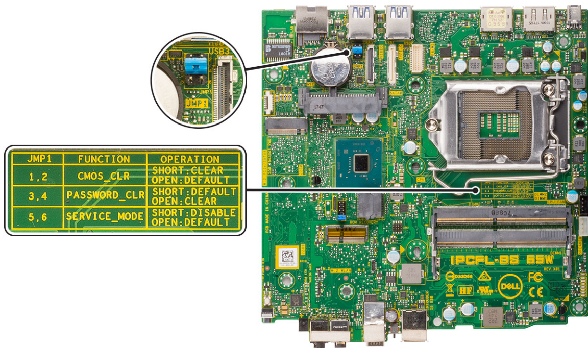
Abbildung 4. Systemplatinenjumper
