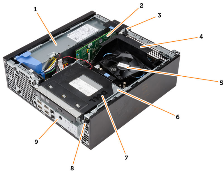
Rysunek 2. Widok wewnątrz
