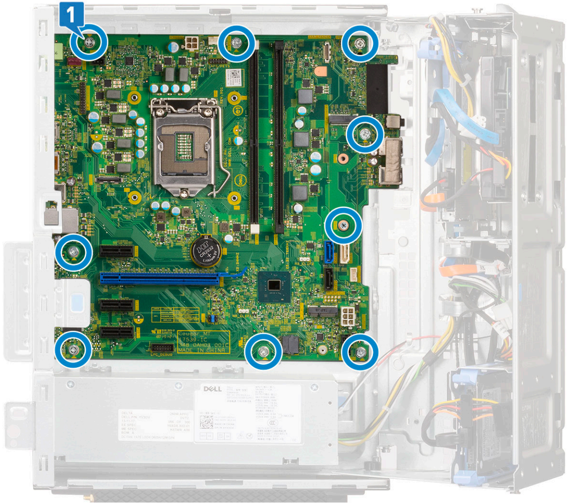
b. החלק והרם את לוח המערכת והוצא אותו מהמחשב [2, 1].
