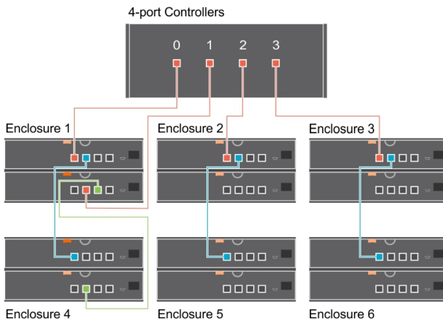
图 1: 将 4 端口控制器连接到单个多路径中的机柜
