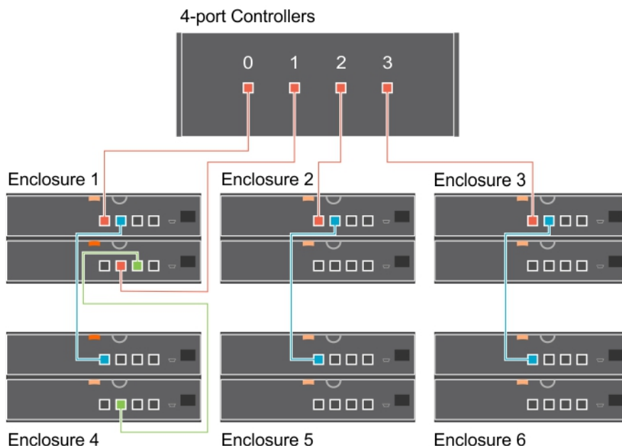
図 1. 単一マルチパスでのエンクロージャへの 4 ポートコントローラーの接続
