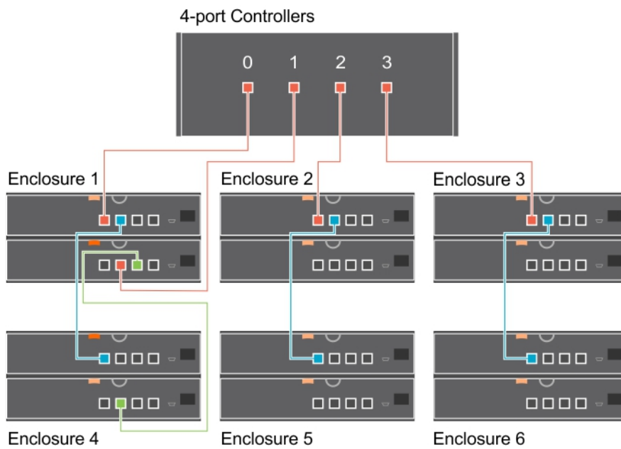
Ilustración 1. Conexión de una controladora de 4 puertos a gabinetes en una conexión única de múltiples rutas
