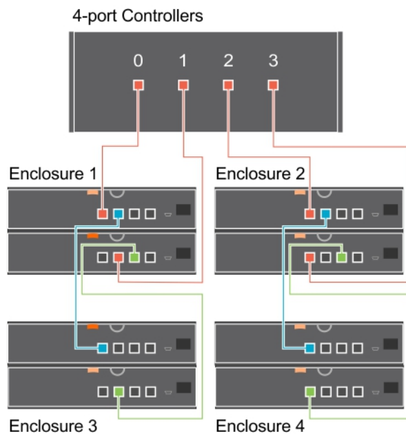
Ilustración 2. Conexión de una controladora de 4 puertos a gabinetes en una conexión múltiple de varias rutas
