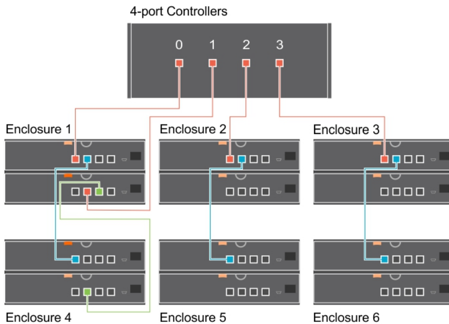
Ilustración 1. Conexión de una controladora de 4 puertos a gabinetes en una conexión única de múltiples rutas
