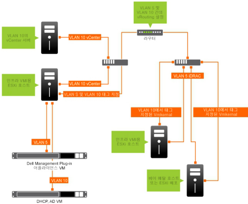
그림 2. VLAN 네트워크.
