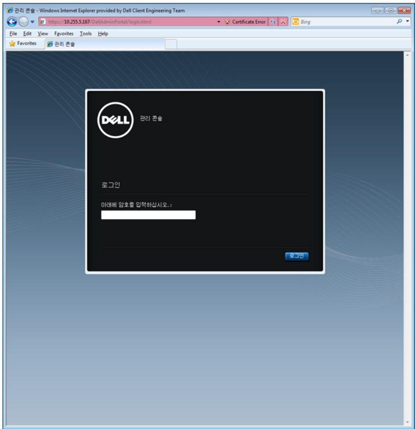
그림 2. 관리 콘솔
