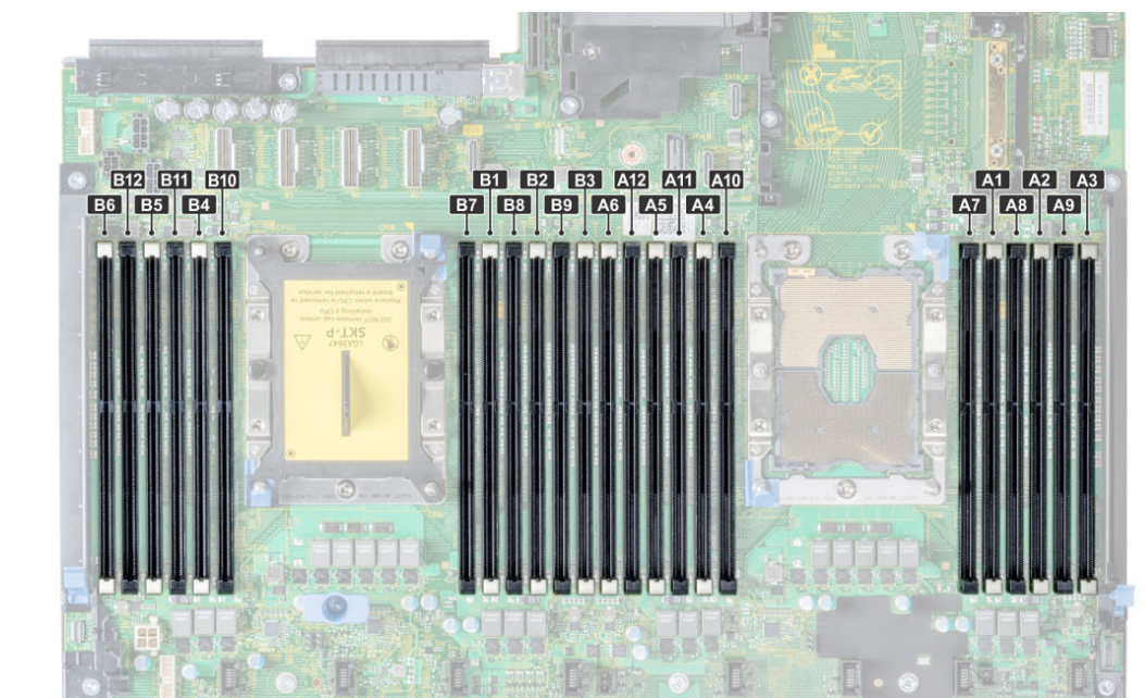
Figure 5. Disposition de la mémoire sur les serveurs R740/R740XD
