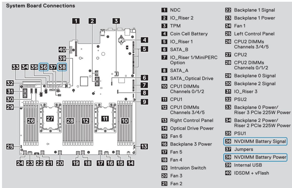
Figure 8. Connexions sur la carte système R740/R740XD
