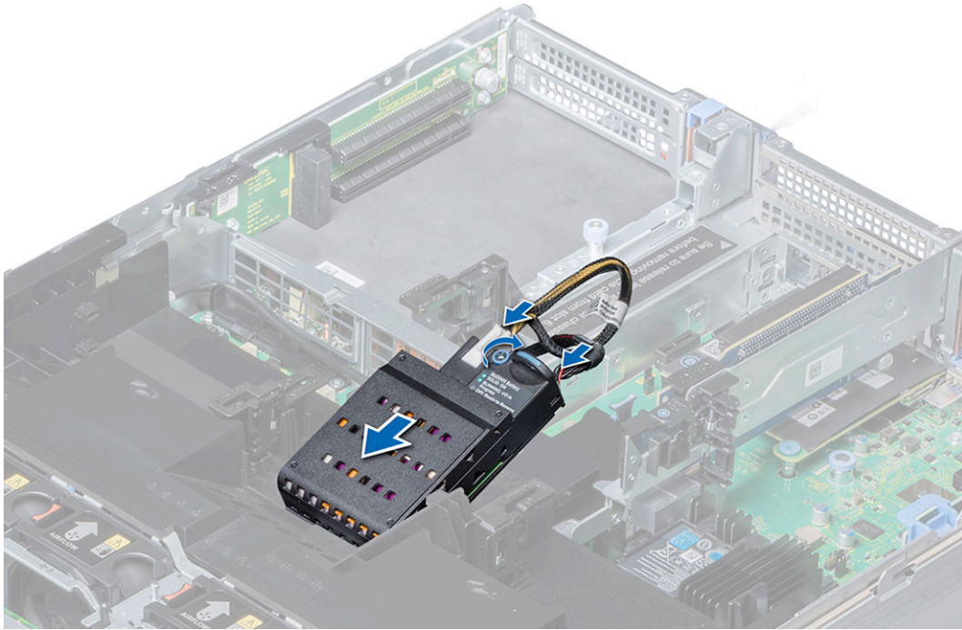
Figure 9. Instructions d'installation de la batterie R740
