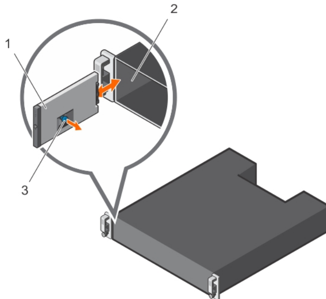
Abbildung 21. Bedienfeldplatte entfernen und installieren
