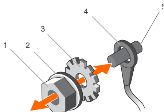
Abbildung 17. Schutzerdungskabel montieren und anschließen
