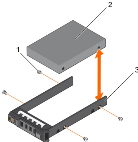
Abbildung 10. Entfernen eines Festplattenlaufwerks aus einem und Installieren in einen 2,5-Zoll-Festplattenlaufwerksträger.
