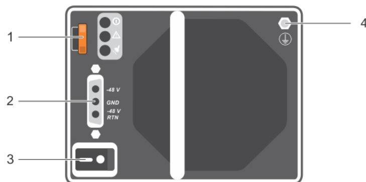
Abbildung 16. Rückseitenmerkmale eines Gleichstrom-Netzteilmoduls
