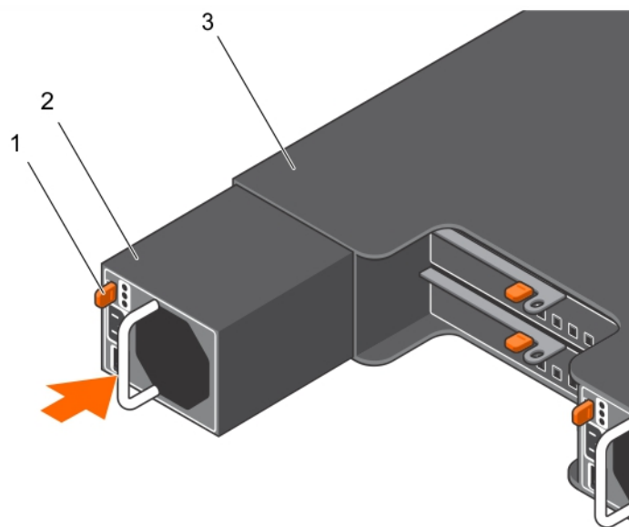
Abbildung 13. Entfernen und Installieren eines Netzteil oder Lüftermoduls
