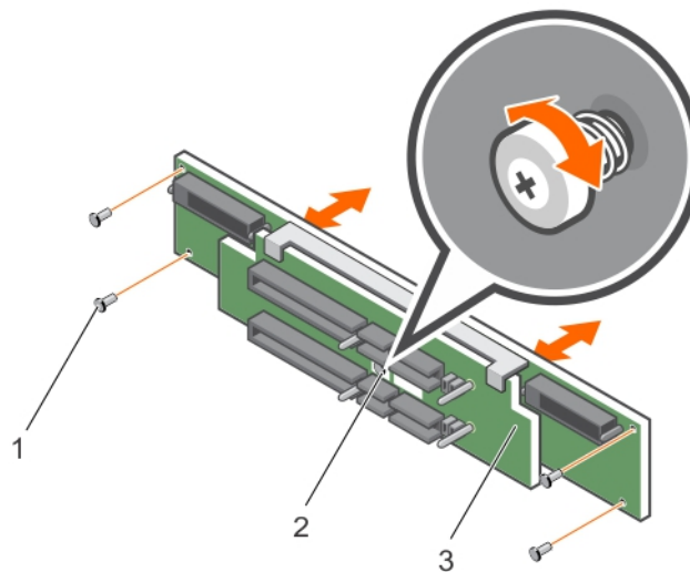
Abbildung 23. Rückwandplatine entfernen und installieren
