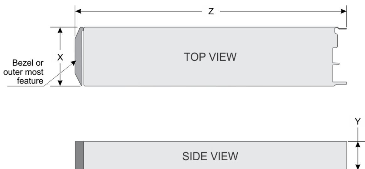
图 6: 机箱尺寸
