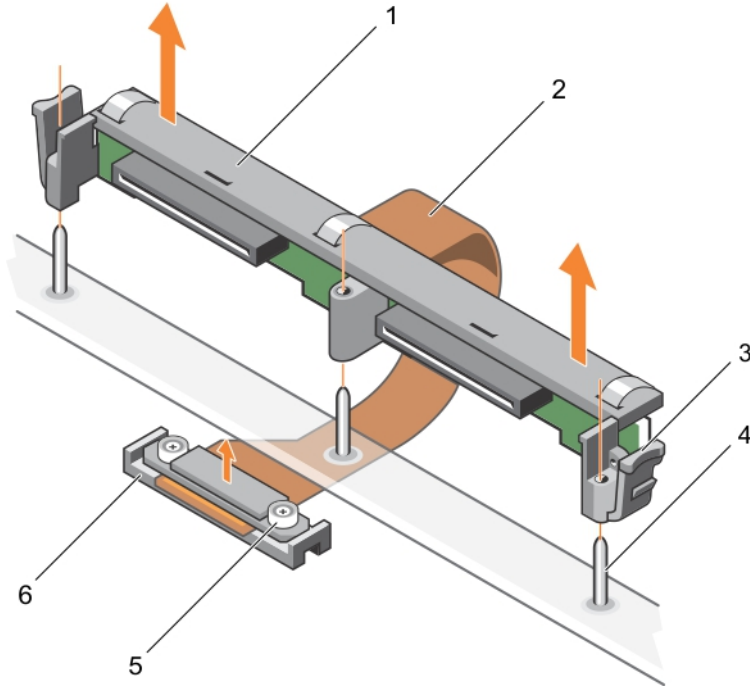
Rakam 54. 2,5 İnç (x2) sabit sürücü veya SSD arka panelini çıkarma
