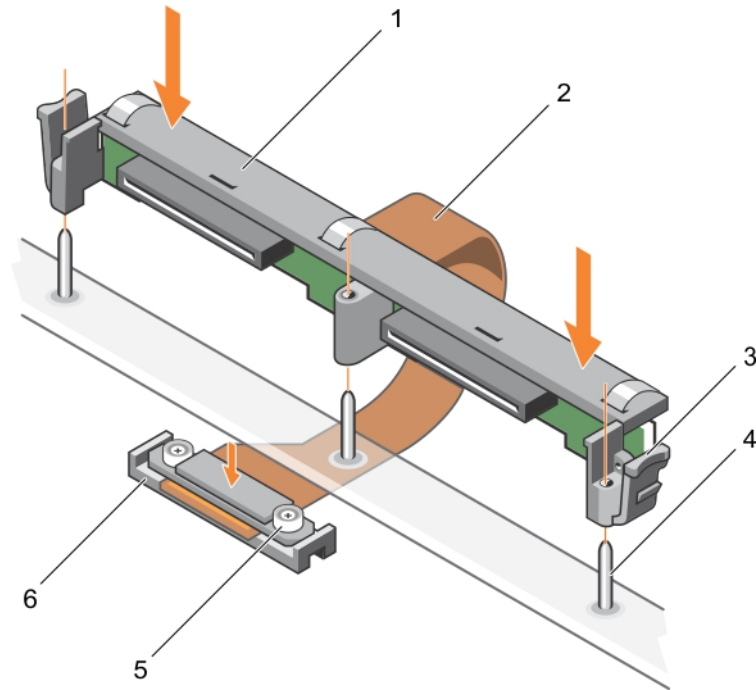
Rakam 56. 2,5 İnç (x2) sabit sürücü veya SSD arka panelini takma
