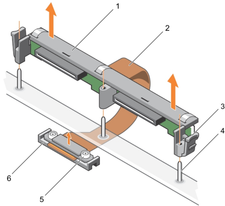
Ilustración 54. Extracción del plano posterior de la unidad de disco duro o SSD de 2,5 pulgadas (x2).
