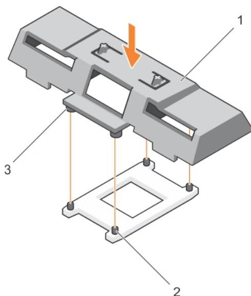
Ilustración 15. Instalación de un procesador/DIMM de relleno
