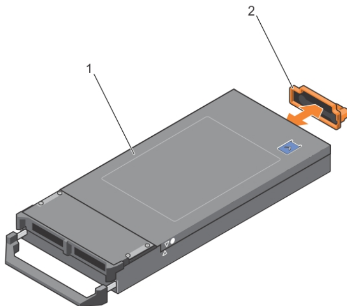
Ilustración 7. Extracción e instalación de la cubierta del conector de E/S
