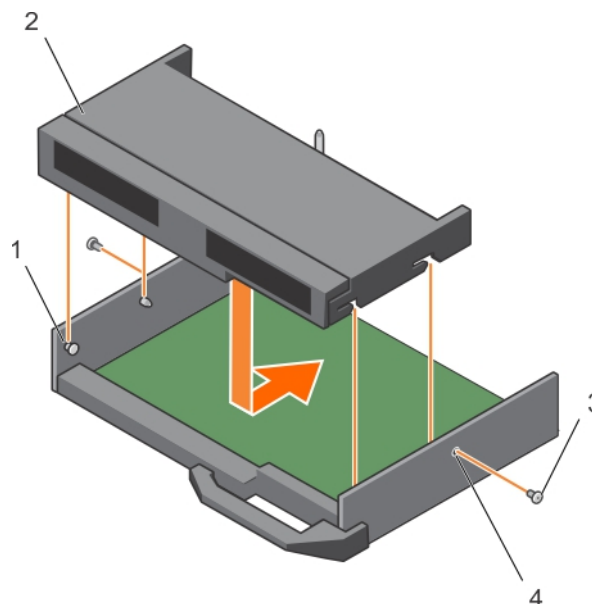
Ilustración 53. Instalación del compartimiento de una unidad de disco duro o SSD
