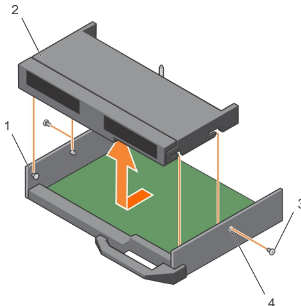
Ilustración 52. Extracción del compartimiento de una unidad de disco duro o SSD
