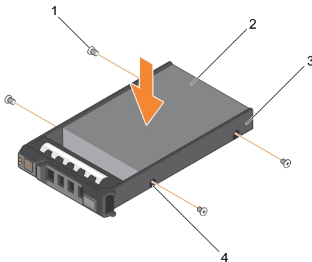
Ilustración 49. Instalación de una unidad de disco duro o SSD de 2,5 pulgadas en un portaunidades de disco duro o SSD de 2,5 pulgadas
