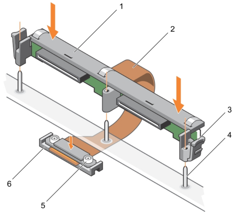
Ilustración 56. Instalación del plano posterior de la unidad de disco duro o SSD de 2,5 pulgadas (x2).
