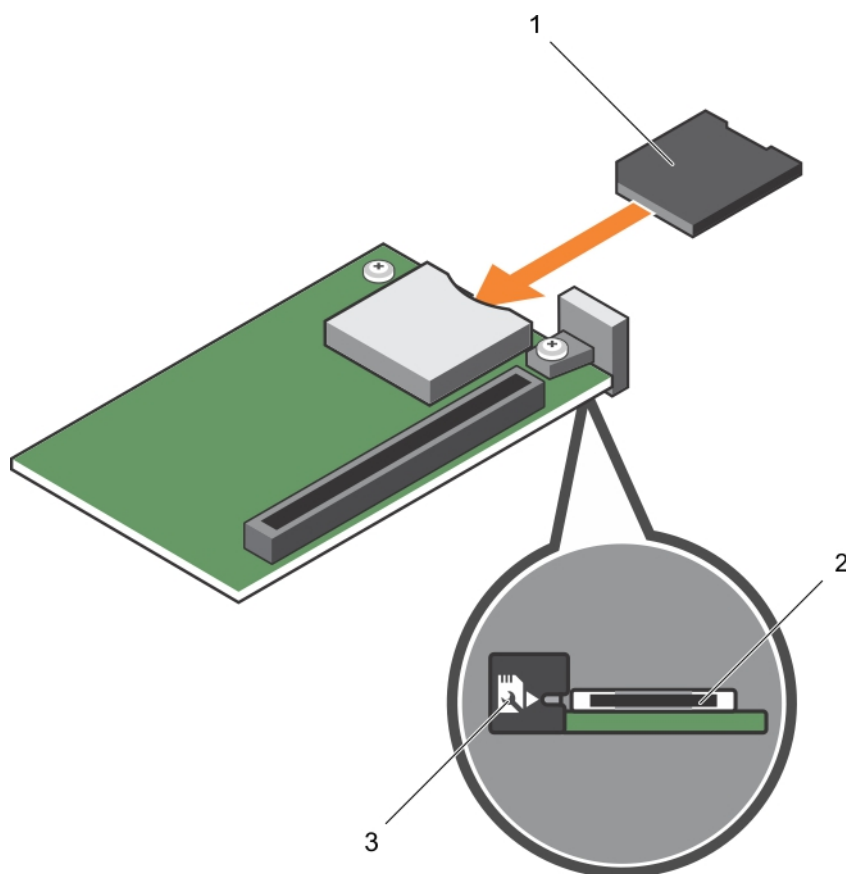
Ilustración 30. Instalación de la tarjeta SD vFlash
