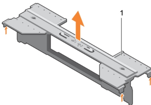
Ilustración 12. Extracción de la cubierta de refrigeración
