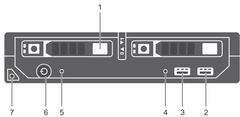
Ilustración 2. Componentes del panel frontal: unidad de disco duro de 2,5 pulgadas o sistema de la unidad SSD
