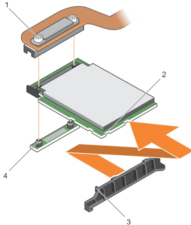
Ilustración 63. Extracción de la tarjeta extendida PCIe o controladora de almacenamiento
