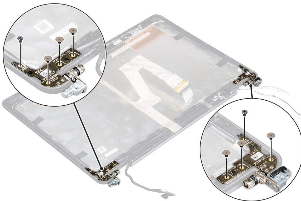
図 2. タッチシステム用ヒンジの取り外し
