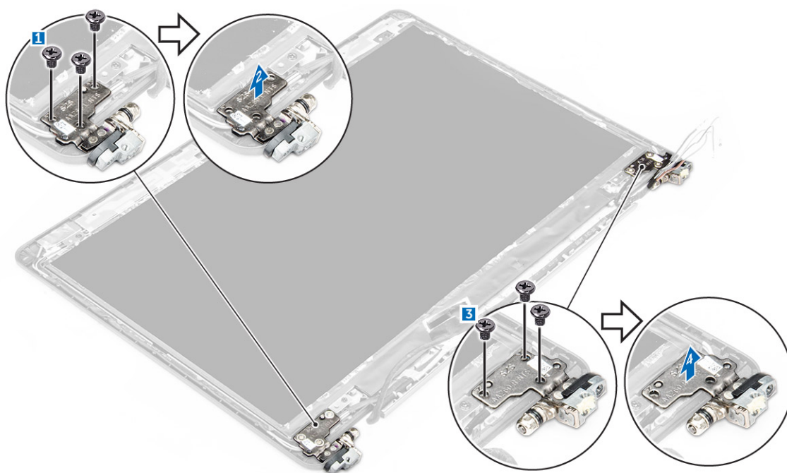
図 1. 非タッチシステム用ヒンジの取り外し
