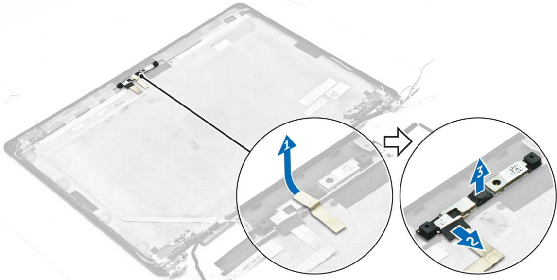
図 5. 非タッチシステムからのカメラの取り外し
