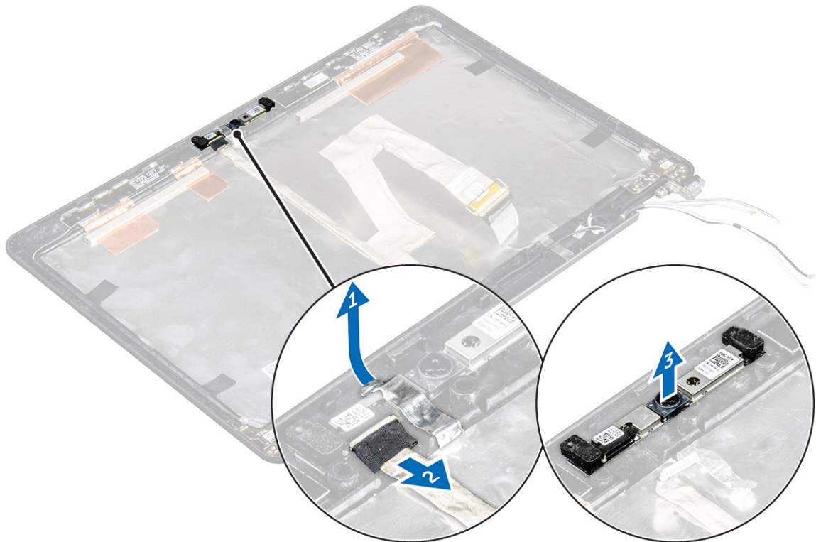
図 6. タッチシステムからのカメラの取り外し
