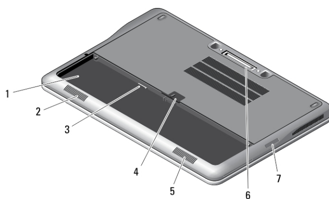
図 6. 底面図 (バッテリーなしの状態)
