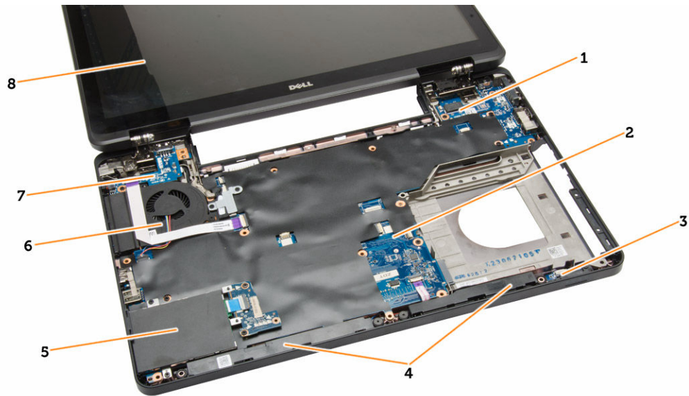
Afbeelding 2. Binnenaanzicht — voorzijde
