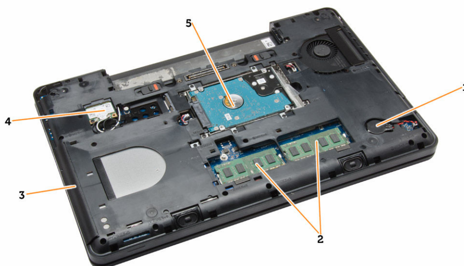
Afbeelding 1. Binnenaanzicht — achterzijde
