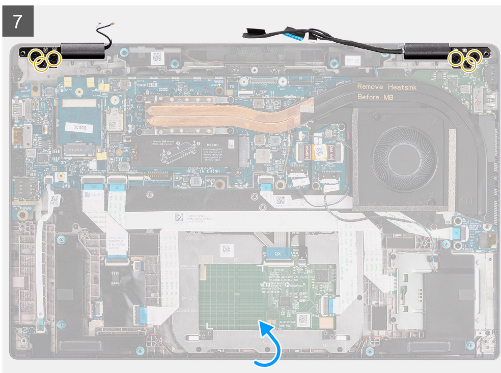
Abbildung 3. Bildschirmbaugruppe mit WLAN- und WWAN-Antenne
