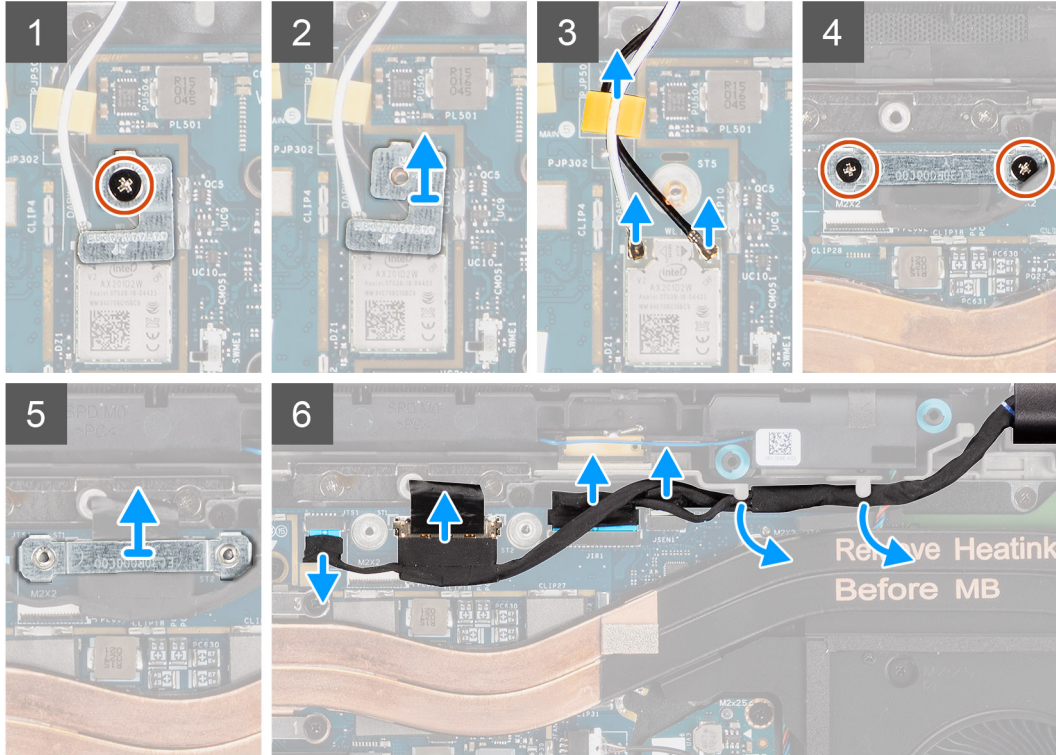
그림 2 . WLAN 안테나가 있는 디스플레이 어셈블리
