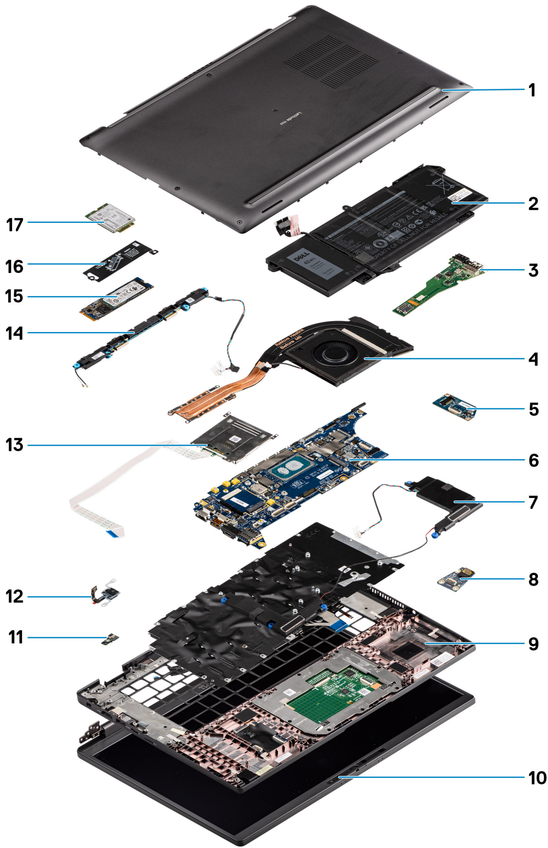
1. 베이스 커버
