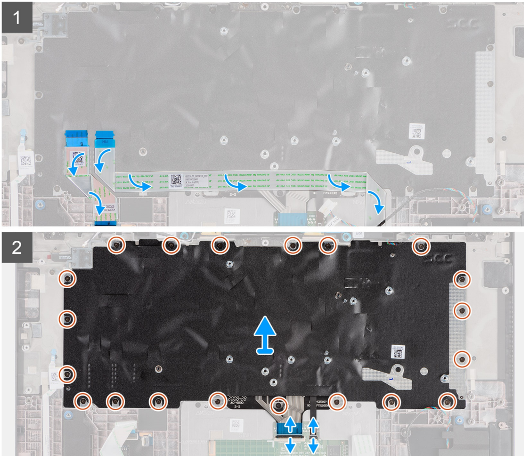
20x M1.6x1.7
