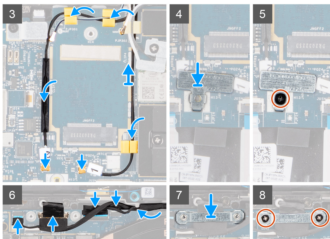
Figure 7. Assemblage d'écran avec câbles d'antenne WLAN et WWAN
