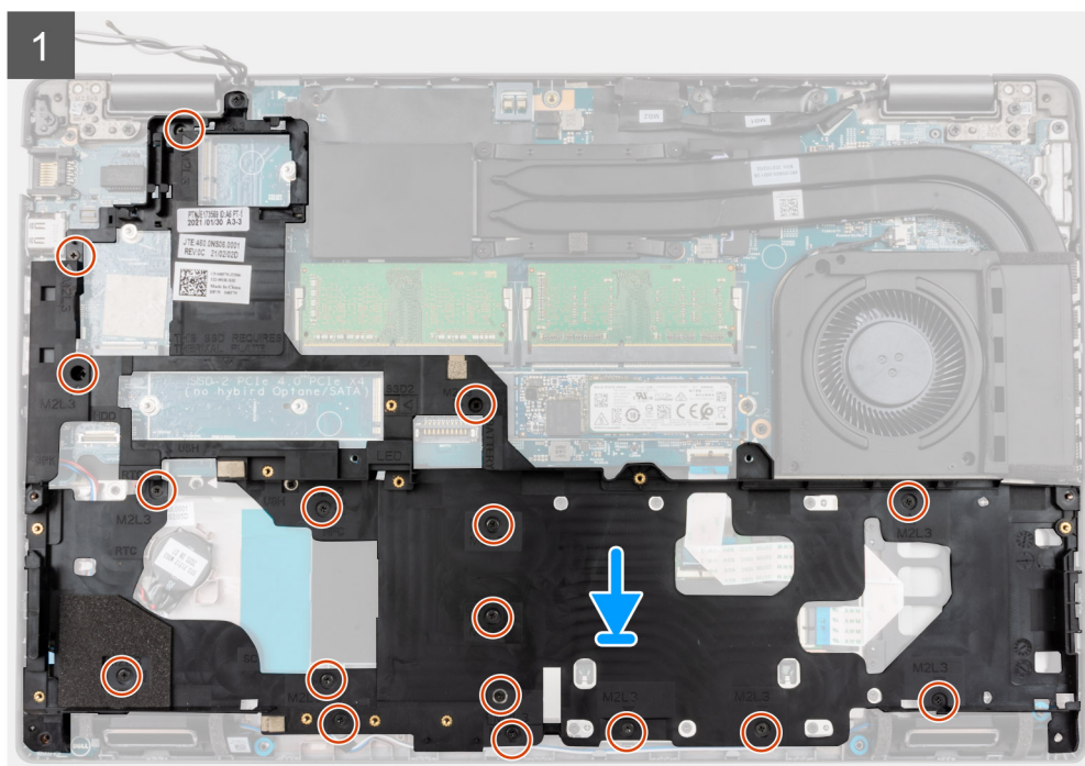
19x M2x3
