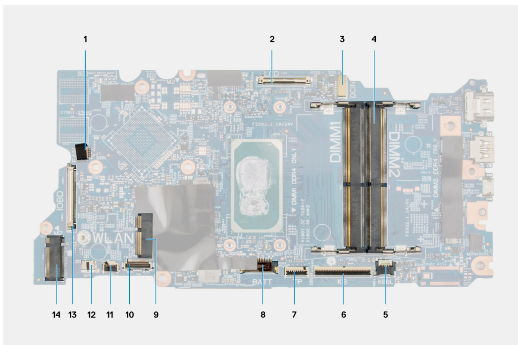
図 2. システム ボードのコネクタース
