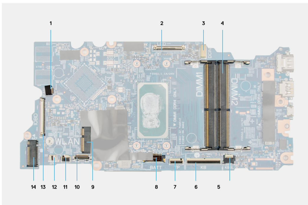
図 4. システム ボードのコネクタース
