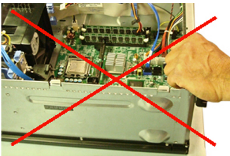
Figura9. Ligação à terra de superfície metálica do chassis (Inaceitável)
