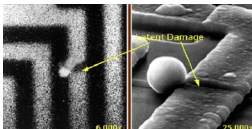
Figura8. Dano intermitente (latente) num rastro de fio
