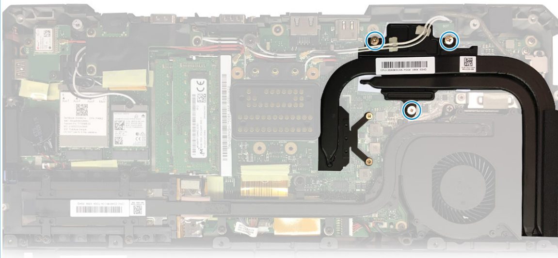
kølelegememodul
