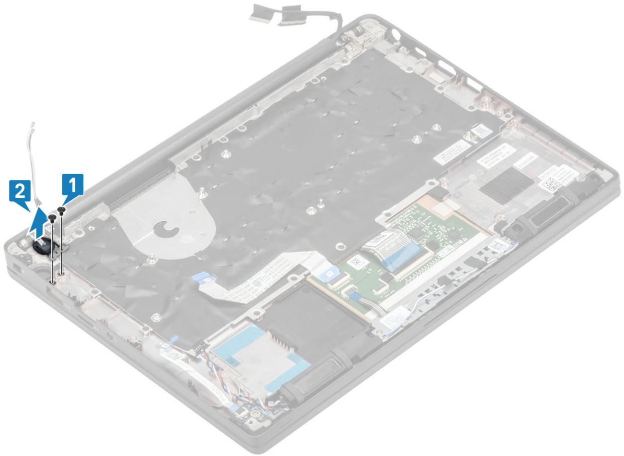
그림 3. FPR이 포함되지 않은 전원 버튼 보드
