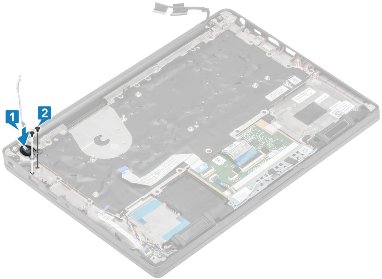
그림 5. 전원 버튼 보드 - FPR 불포함
