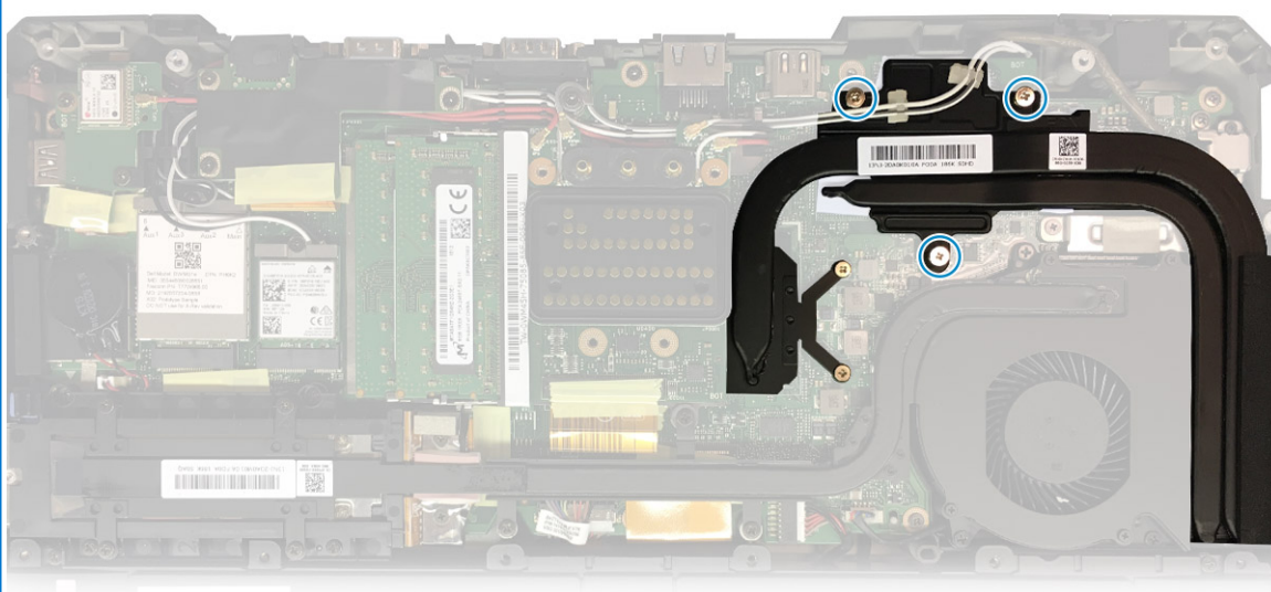
radiatorului DSC
