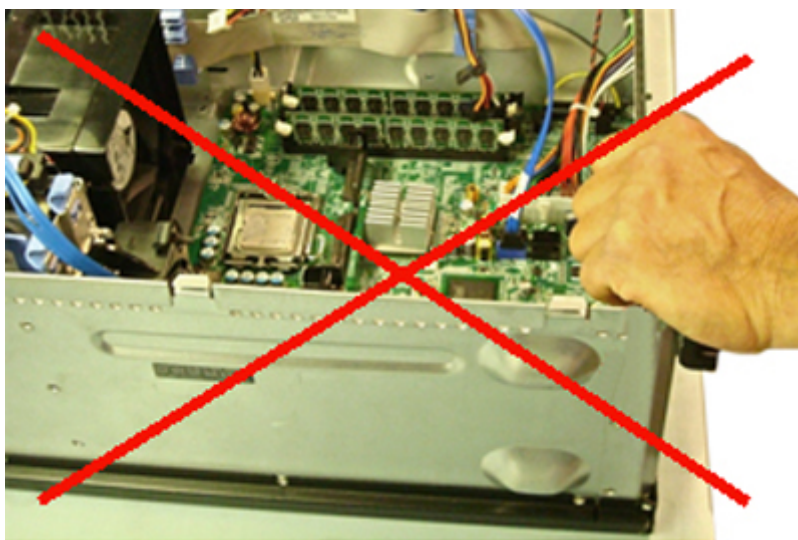
Figura 9. Aterramento em metal descoberto do chassi (inaceitável)
