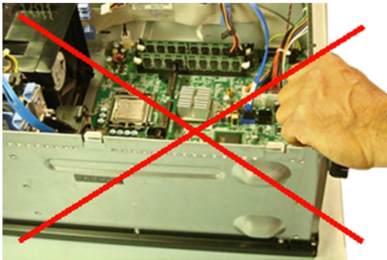
図 9. シャーシの「ベアメタル」接地（非許容）
