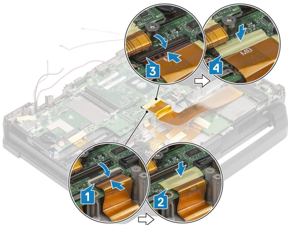
Carte mère
