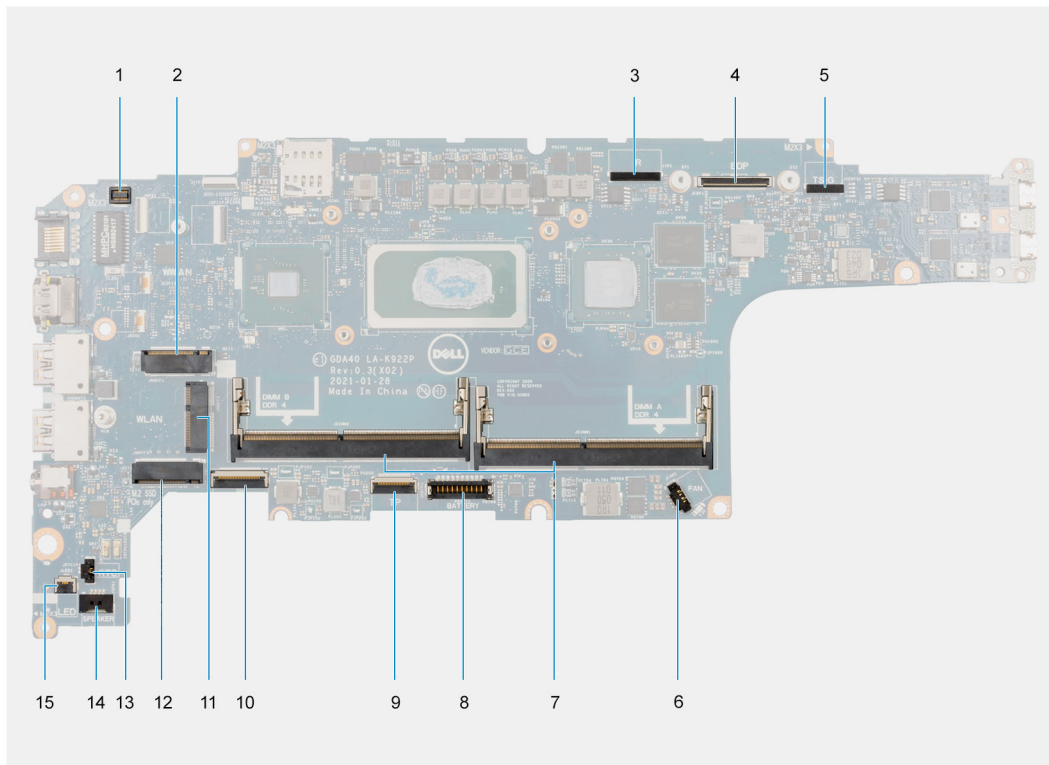
그림 2. 시스템 보드 커넥터
