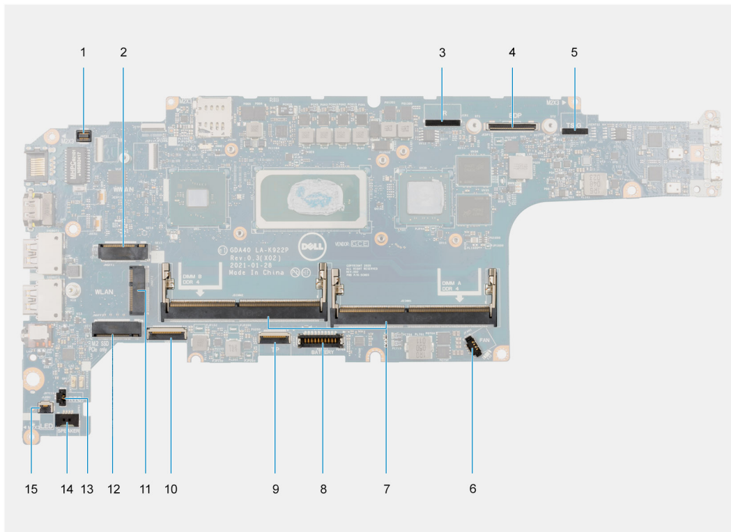
그림 1. 시스템 보드 커넥터
