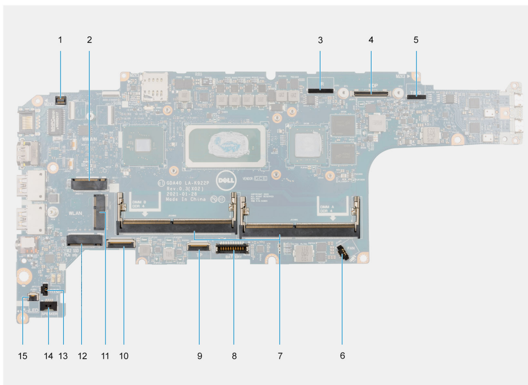
Figure 2. Connecteurs de la carte système
