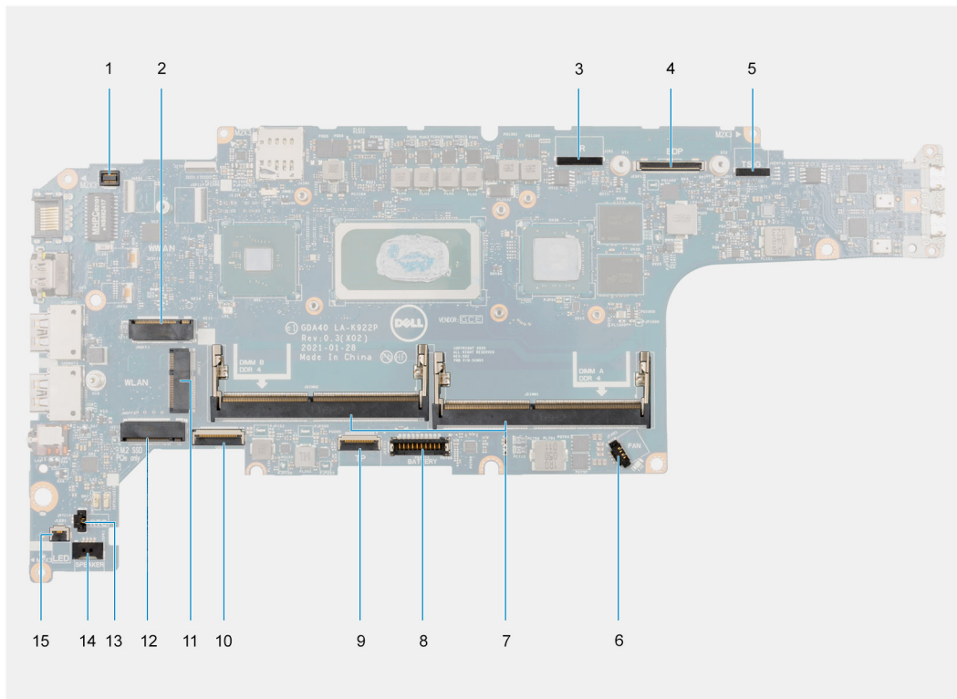
Abbildung 1. Hauptplattenanschlüsse
