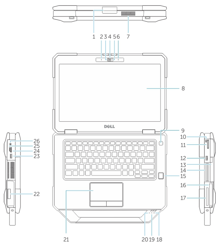
Ilustración 1. Descripción general del sistema
